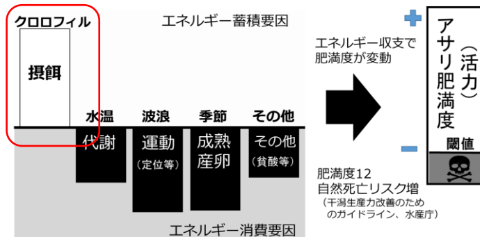
アサリ個体におけるエネルギー収支のイメージ（Sindo and Hibino, 2025を改変）
