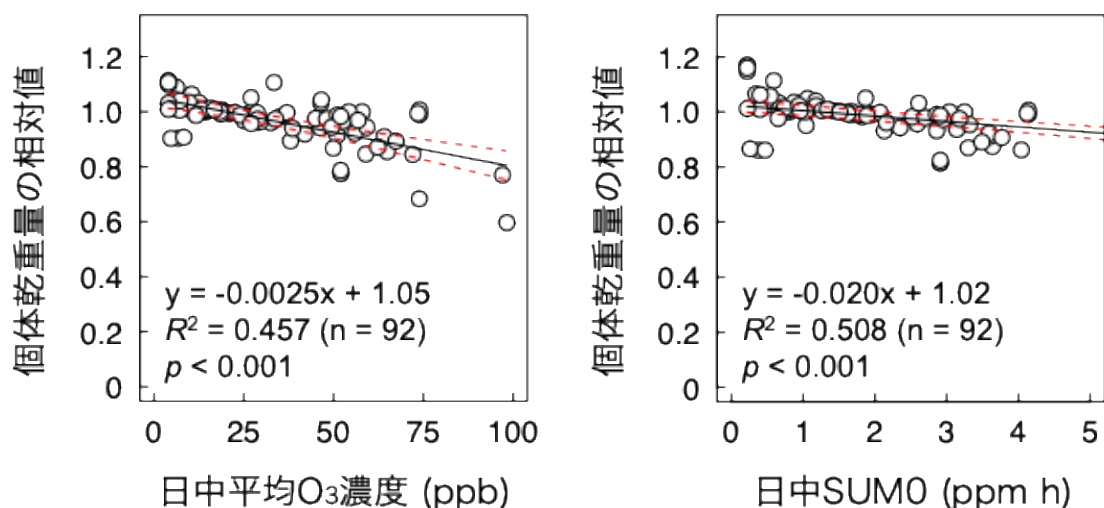
図 62 ハツカダイコン（品種：コメット）の個体乾重量の O 3 曝露-応答関係.
