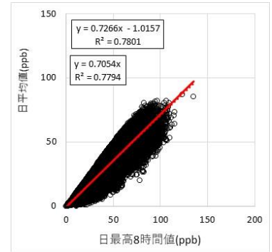
図 89 【2016 年度】(n=386802, 測定局数=1083, 相関係数=0.883)
