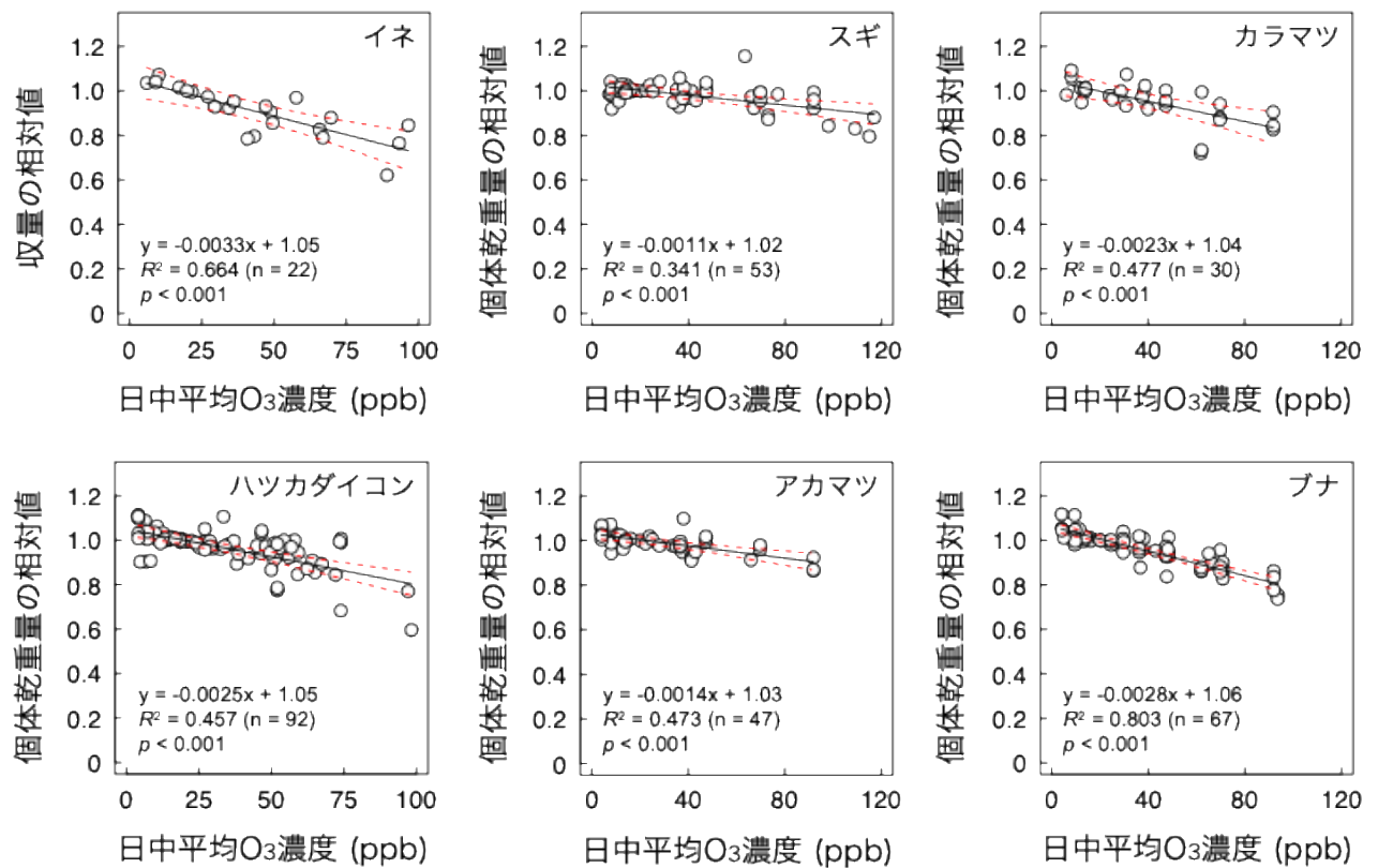
図 67 イネ（品種：コシヒカリ）の収量とハツカダイコン（品種：コメット）、スギ、アカマツ、カラマツ及びブナの個体乾重量の O 3 曝露-応答関係。
