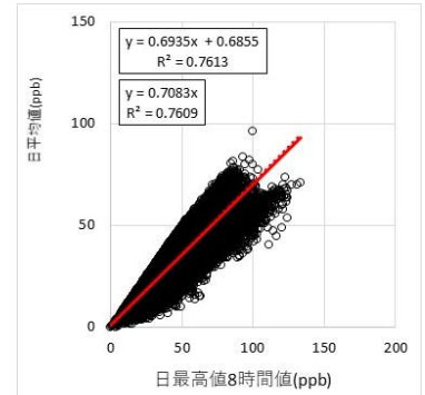
図 95 【2022 年度】(n=398916, 測定局数=1115, 相関係数=0.873)
