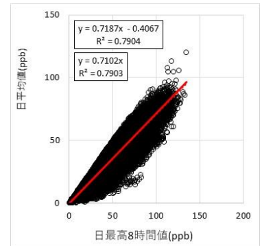
図 92 【2019 年度】(n=404285, 測定局数=1131, 相関係数=0.889)
