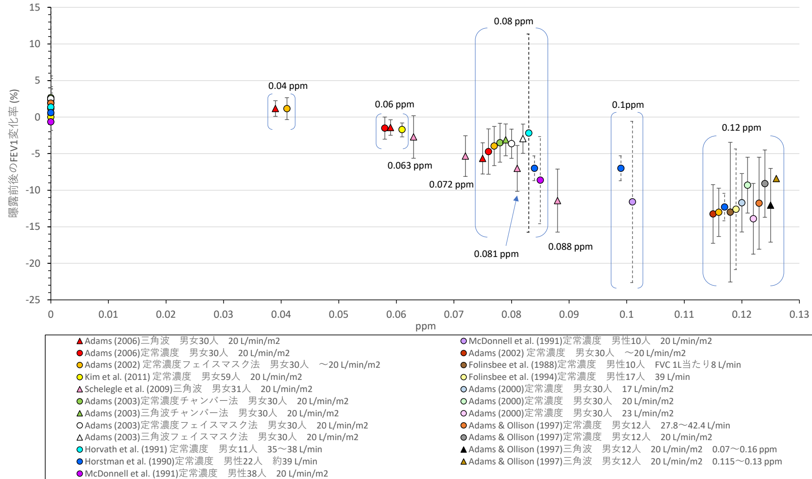
図 9 健康な被験者を間欠運動条件下で 6.6 時間 O_3 に曝露した研究における FEV 1 変化率
