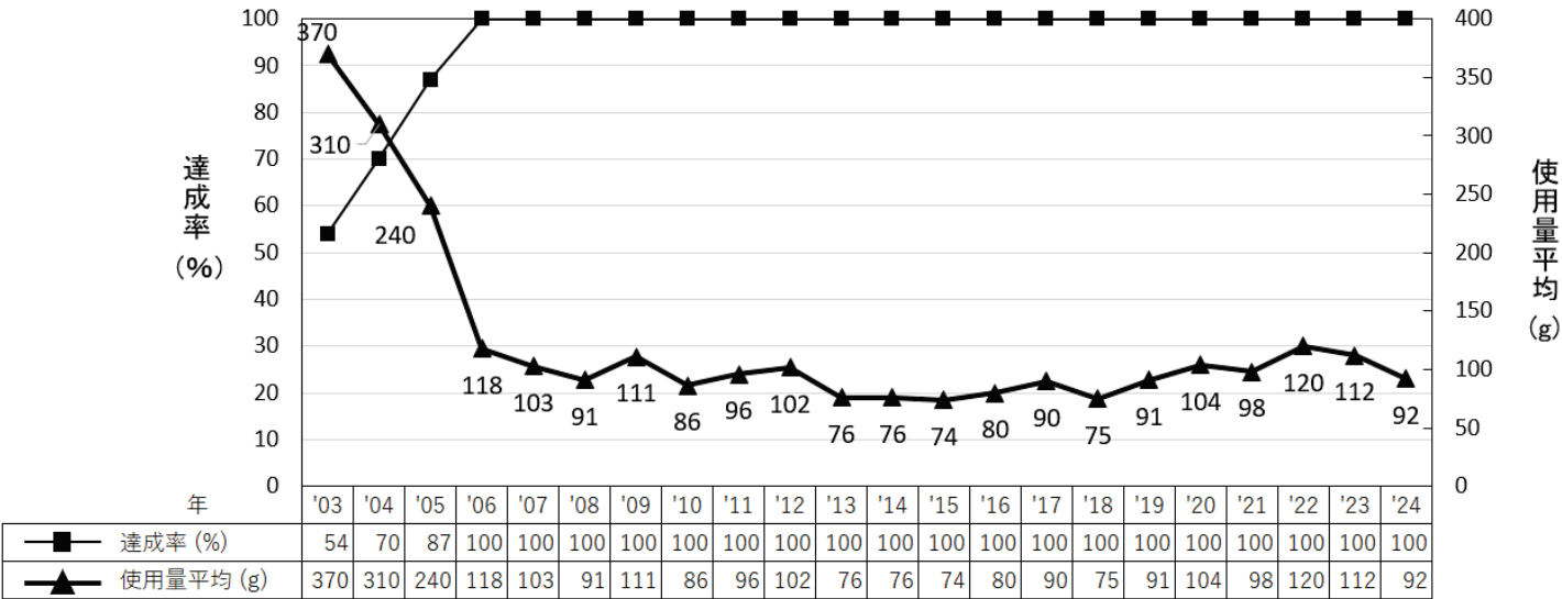
図1. 鉛使用量削減状況(乗用車平均)2003年～2024年(1～12月)推移
