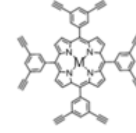
M: Ni, Co, Cu M-P_8e
