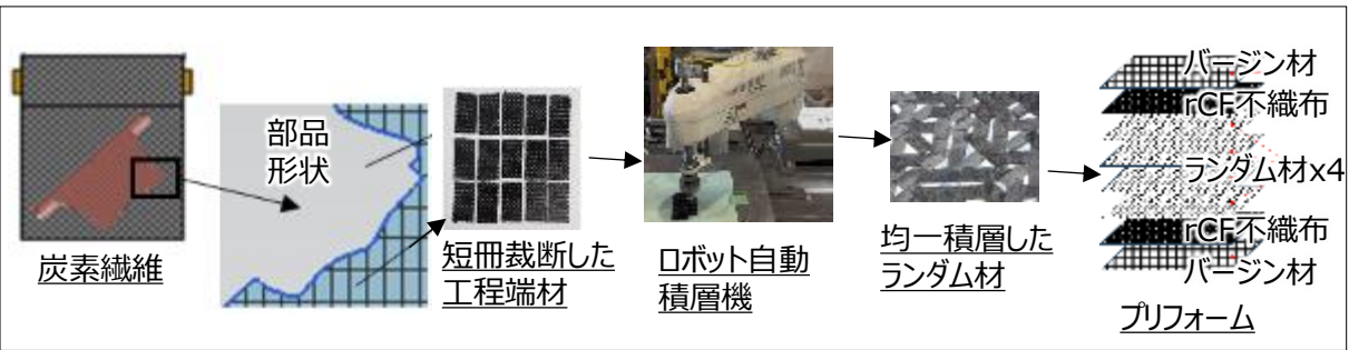
図1.プリフォーム工程の流れ
