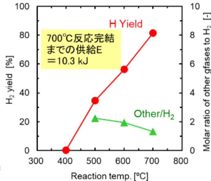
混練法 50 mol%-NiO/AlOx触媒の水素収率と他ガス生成比の反応温度依存性
