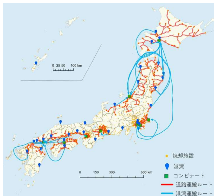
図 一般廃棄物からのコンビナートにおけるWaste to Steam（廃棄物焼却施設から産業施設への蒸気供給）の多目的最適化結果
