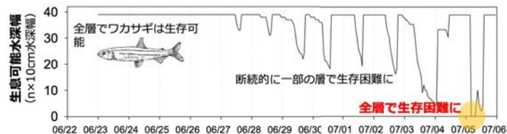
図 高水温と貧酸素の現状とワカサギへの影響。
