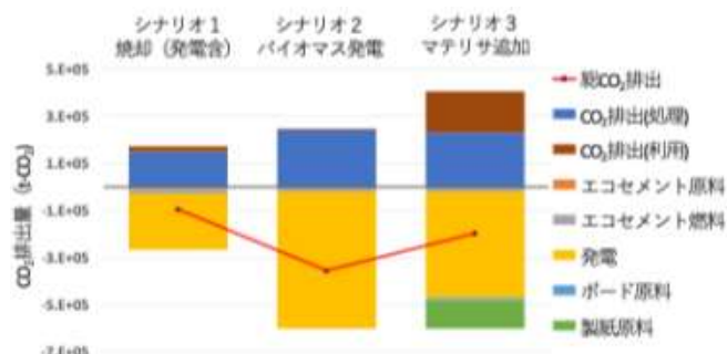
図 木質系災害廃棄物処理シナリオのライフサイクルカーボン（LCCO2）評価結果
