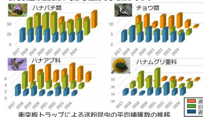
図 避難指示区域等における昆虫のモニタリングの結果（左）とカメラトラップによる2023年のイノシシの撮影頻度（右）
