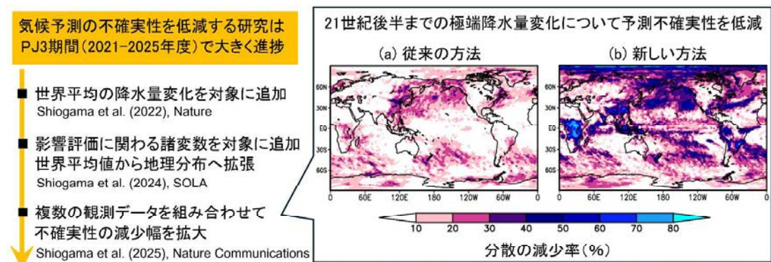
図 極端降水量の将来予測を観測データで制約したことによる予測不確実性（分散）の減少率
