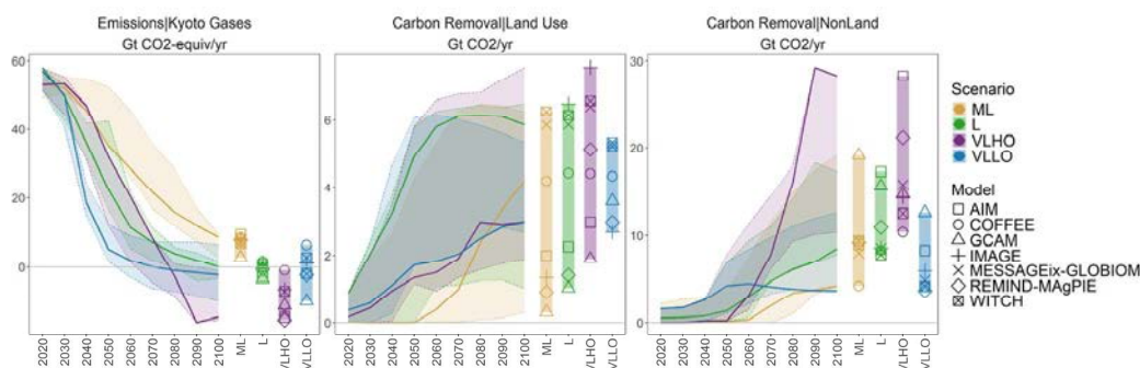
図 Scenario MIPにおけるGHG排出および技術由来・土地由来の二酸化炭素除去の経路 ML：緩和努力の遅滞を伴うシナリオ L：2℃未満に抑える可能性が高いシナリオVLHO：大規模オーバーシュート VLLO：小規模オーバーシュート
