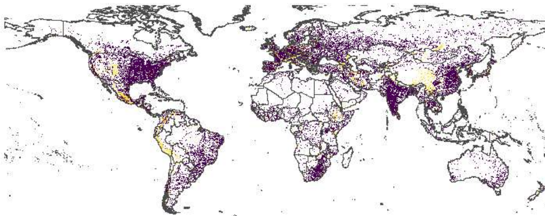
図 再生可能エネルギー資源の適地の空間分布
