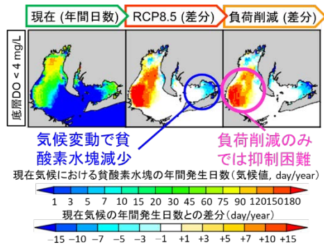
図 2-1 伊勢湾・三河湾におけるシミュレーション結果
