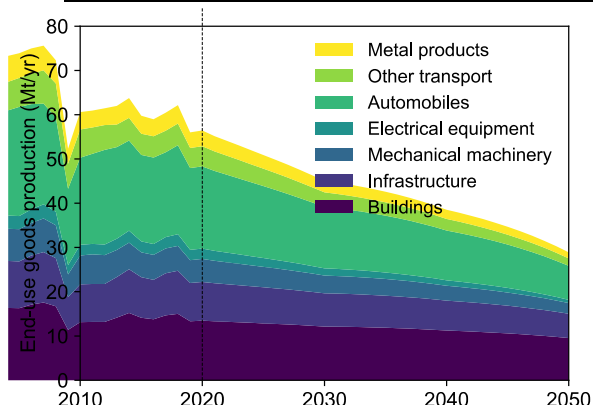
図 CN炭素制約と整合する日本の鉄鋼利用の推移
