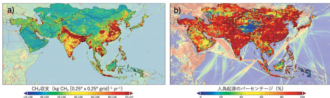
図 アジアのCH 4 収支分布。a) 合計収支、b) 総放出に対する人為起源放出の割合
