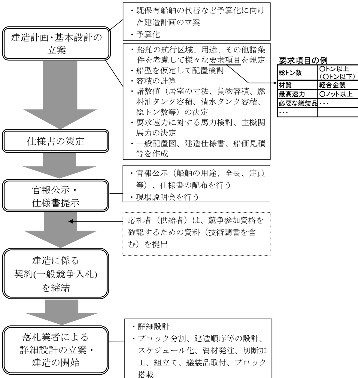
図IV-2-1 調達者が概要設計、基本設計を行う場合の標準的なフロー
