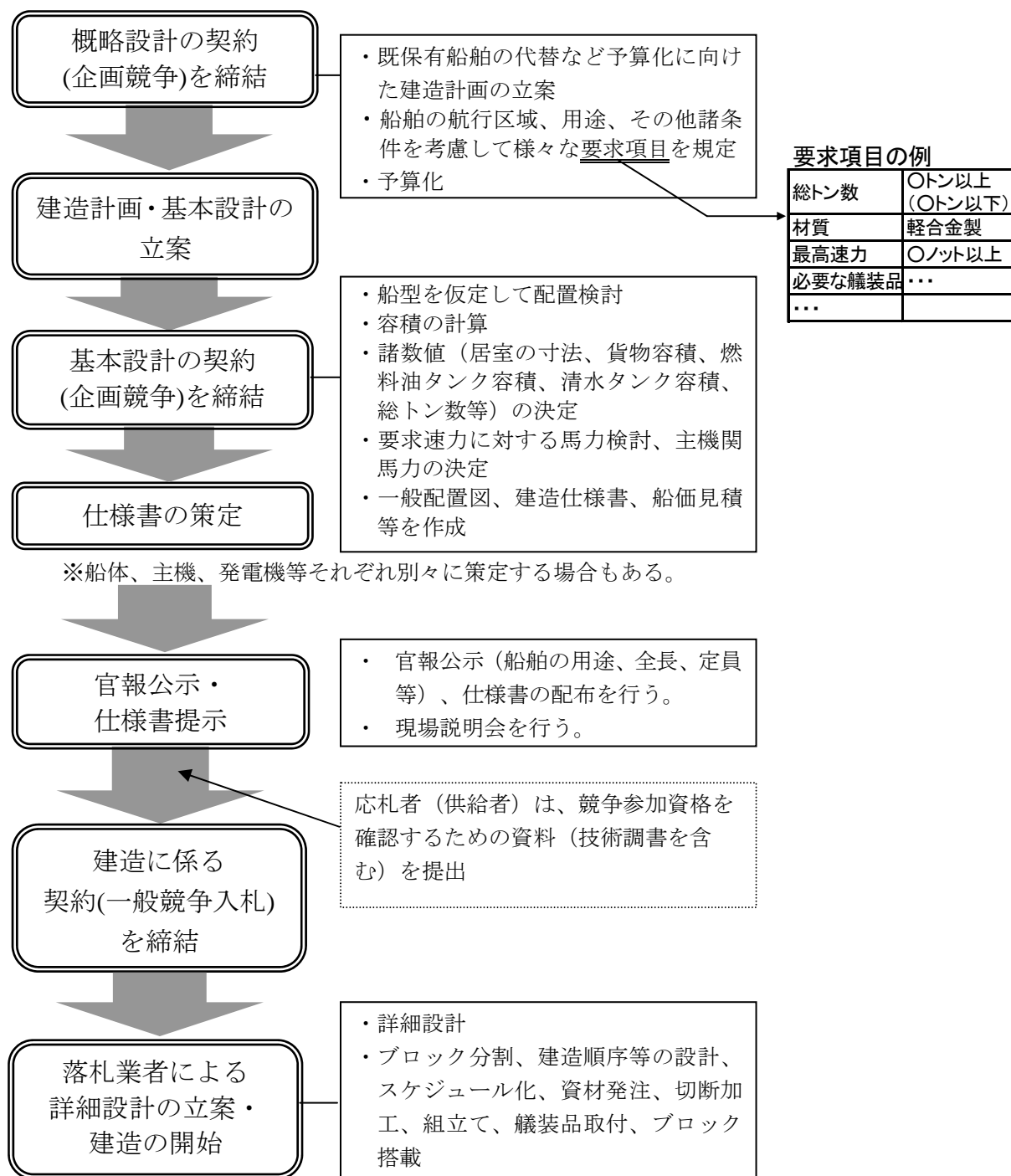
図IV-2-2 調達者が設計者に概要設計、基本設計を発注する場合の標準的なフロー
