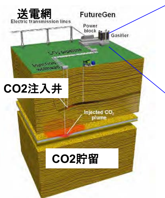
ゼロエミッション石炭火力発電所の例（米国FutureGen）
