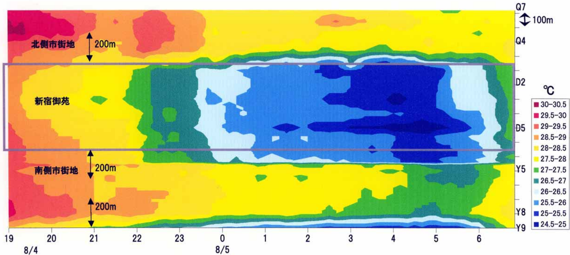
第5図 Q-D-Y測線の気温アイソプレス図 (8/4 19:00 ~ 8/5 7:00)
