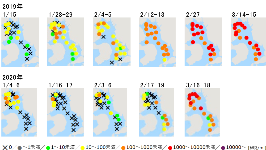
図 2.8.3-10 Eucampia zodiacus の出現状況の変化(2019(令和元)年1月～3月及び2020(令和2)年1月～3月)
