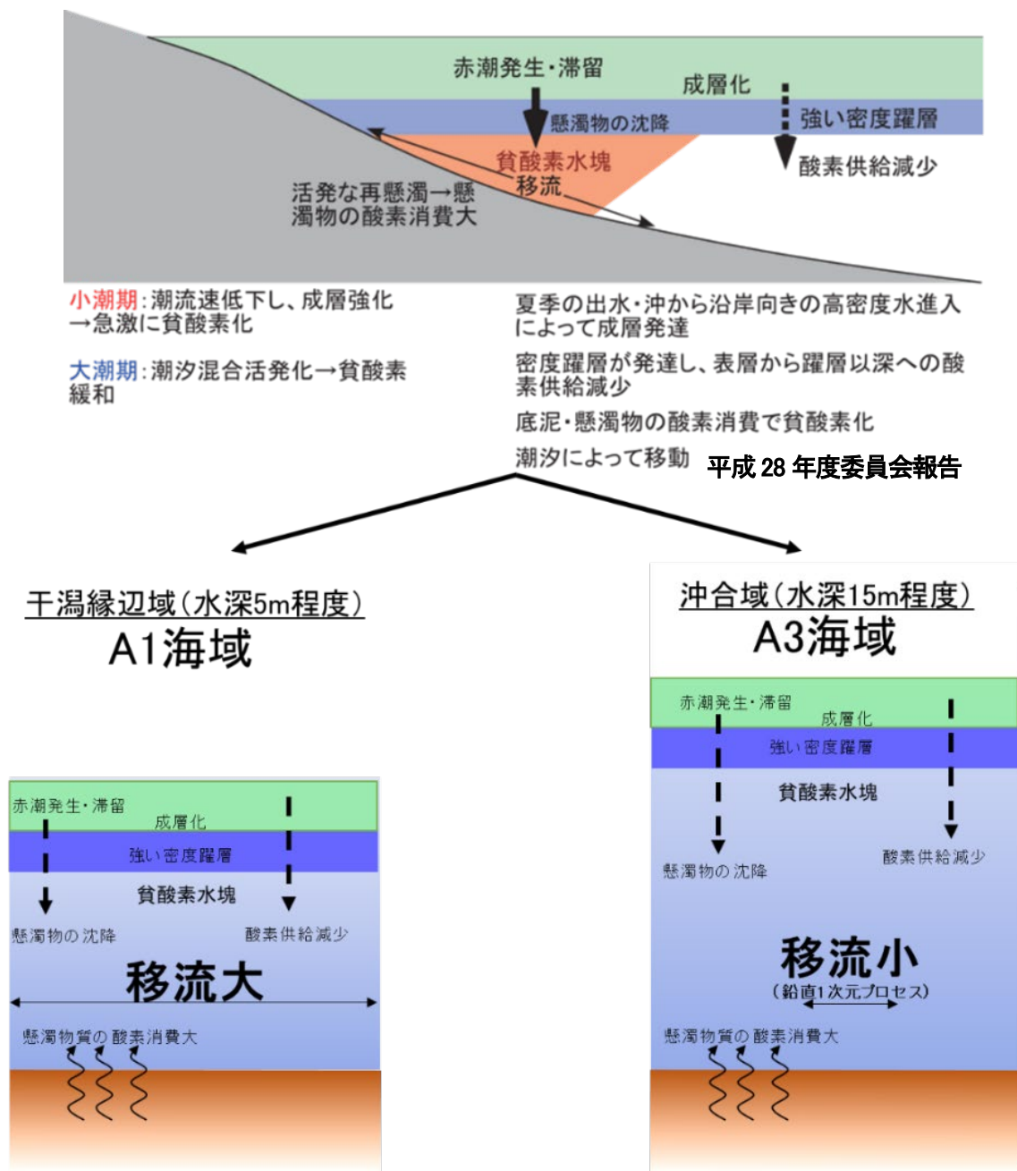
図 2.6.2-2 有明海湾奥部における貧酸素水塊発生の模式図
