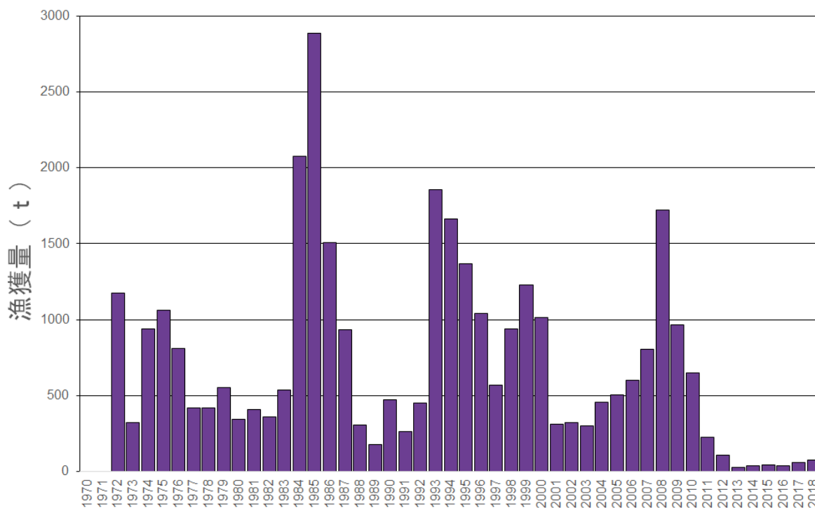
図 2.9.3-11 八代海におけるアサリ類漁獲量の推移
