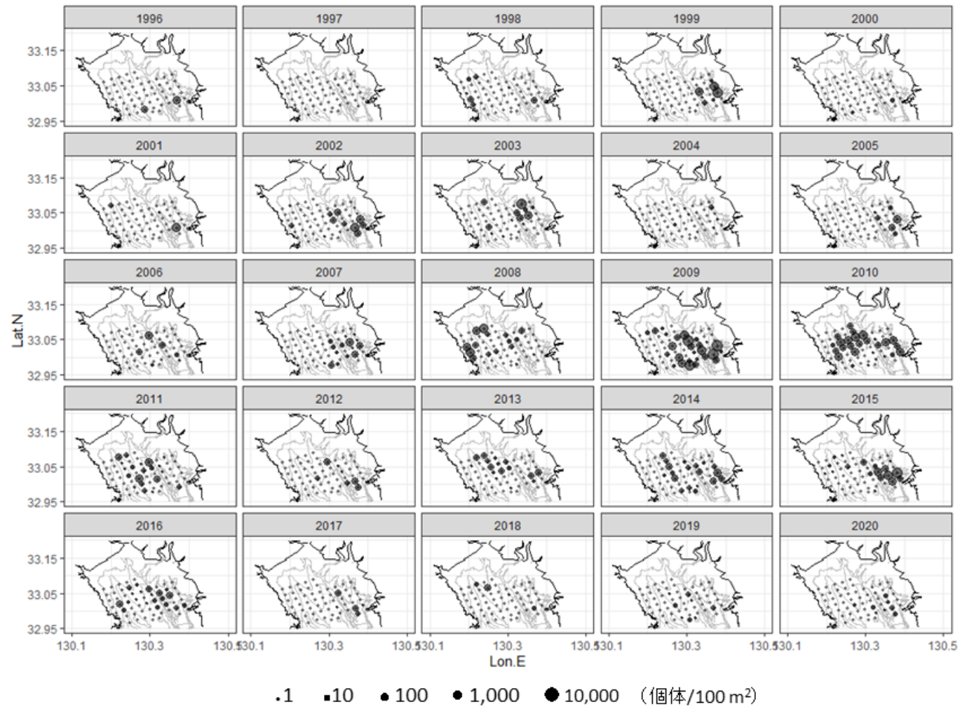
図 2.9.3-3 タイラギ稚貝の分布の推移(1996(平成8)～2019(令和元)年)
