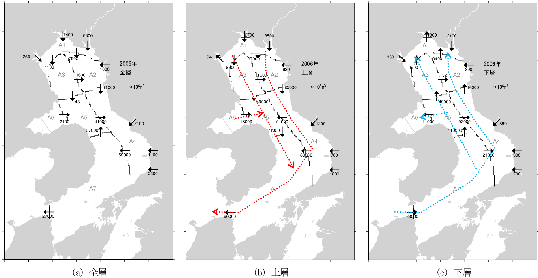
図 12 2006 年通年の流量収支
