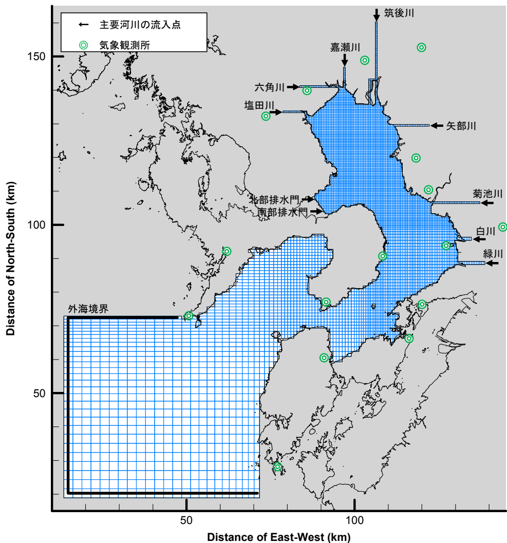
図3 計算格子
