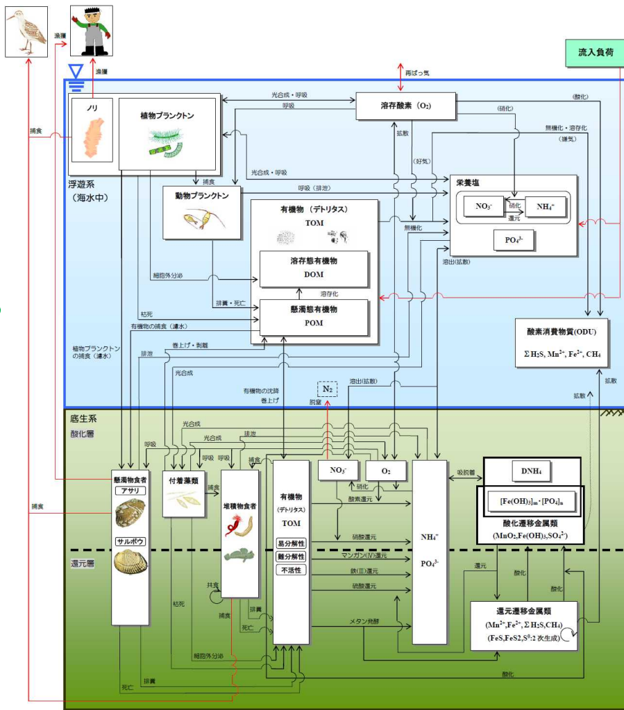
図4 水質・底質・底生生物サブモデルで考慮する物質循環
