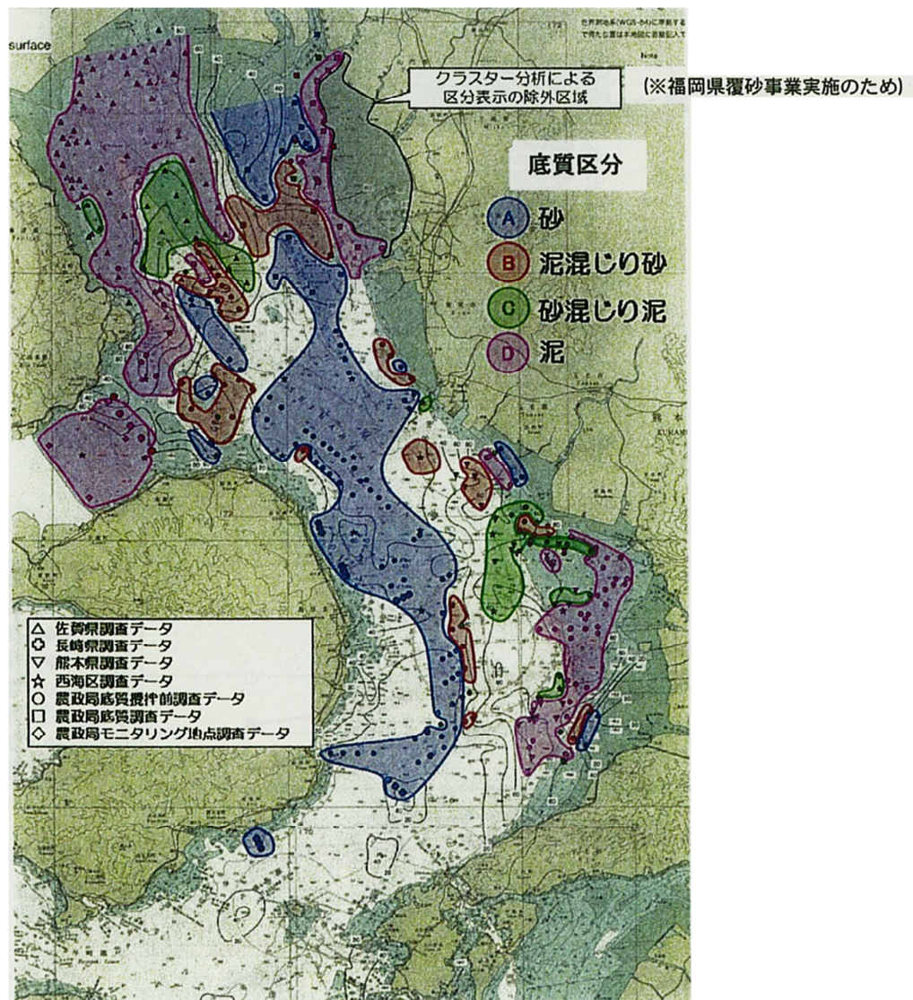
図1 有明海の底質特性別海域区分図(2014年)
