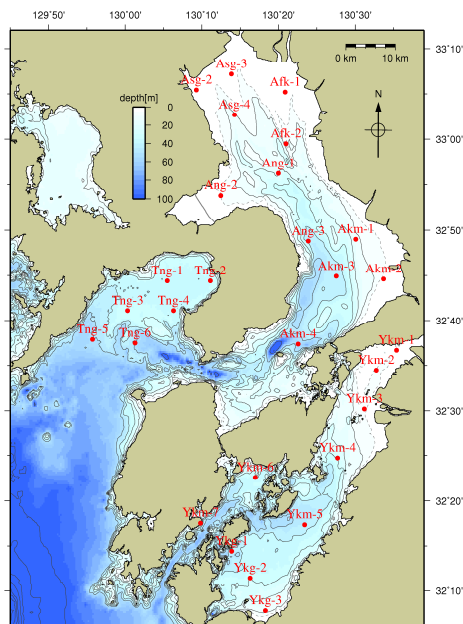
図4 有明海における底質の調査地点
