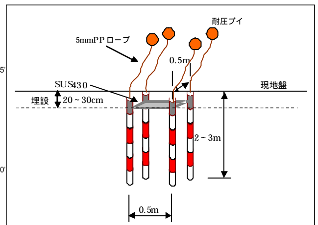
図7 埋没測定板の装置の概要
