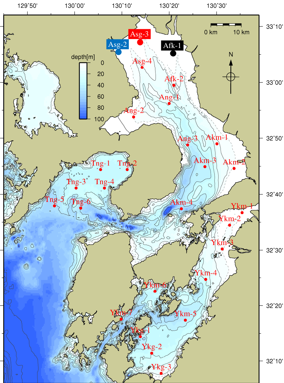
図 3 A 1 海域におけるベントス調査地点
