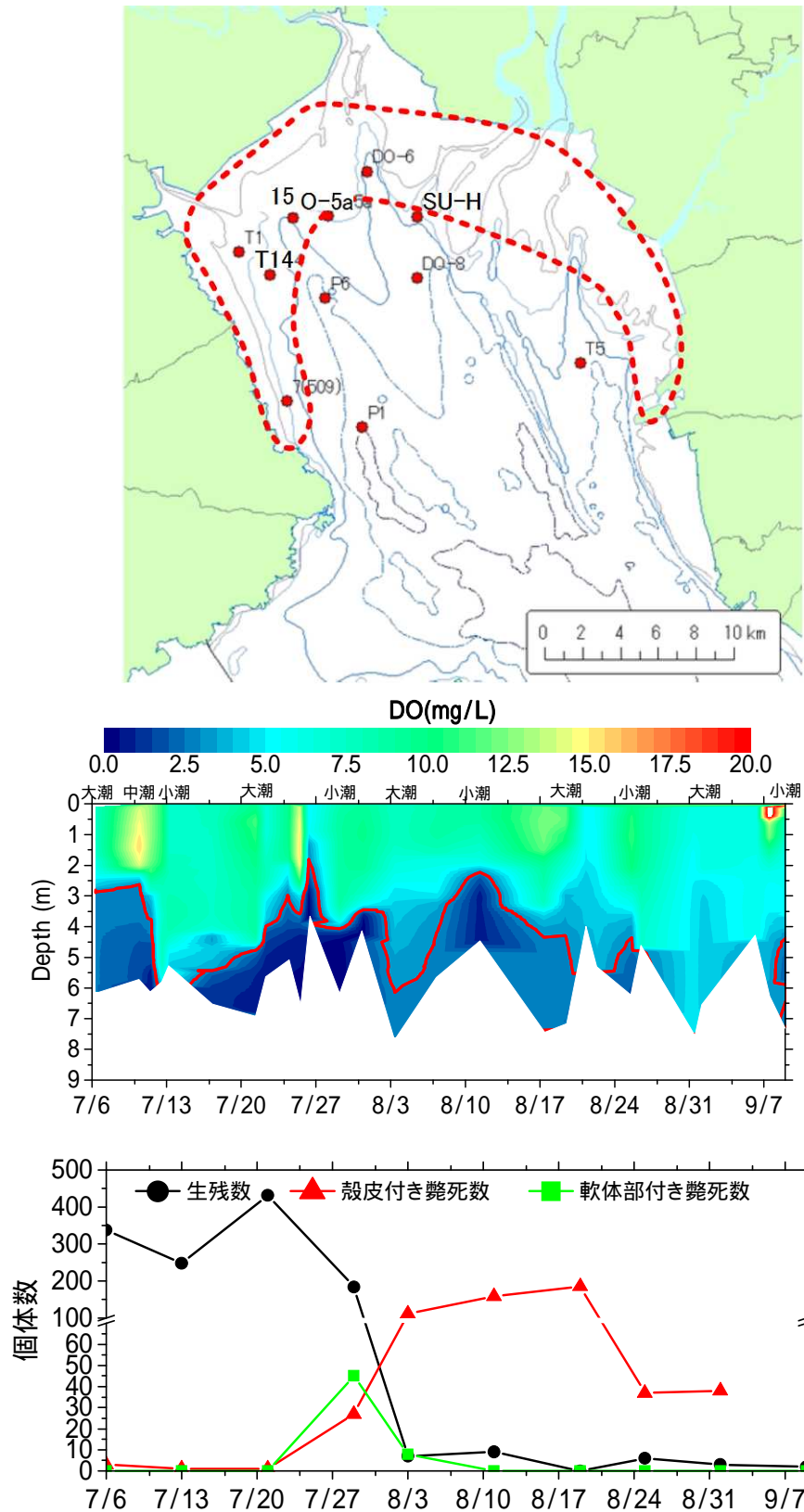
図 13 A 1 海域 浜川沖 (T14) における溶存酸素濃度分布とサルボウ生息状況の変動 (2012 年)
