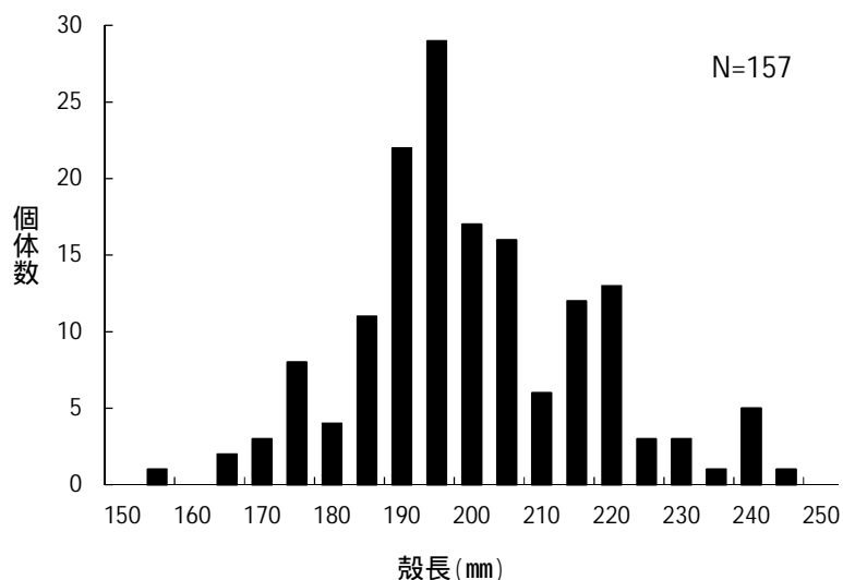
図12 干潟で採捕されたタイラギの殻長組成(2014年調査)
