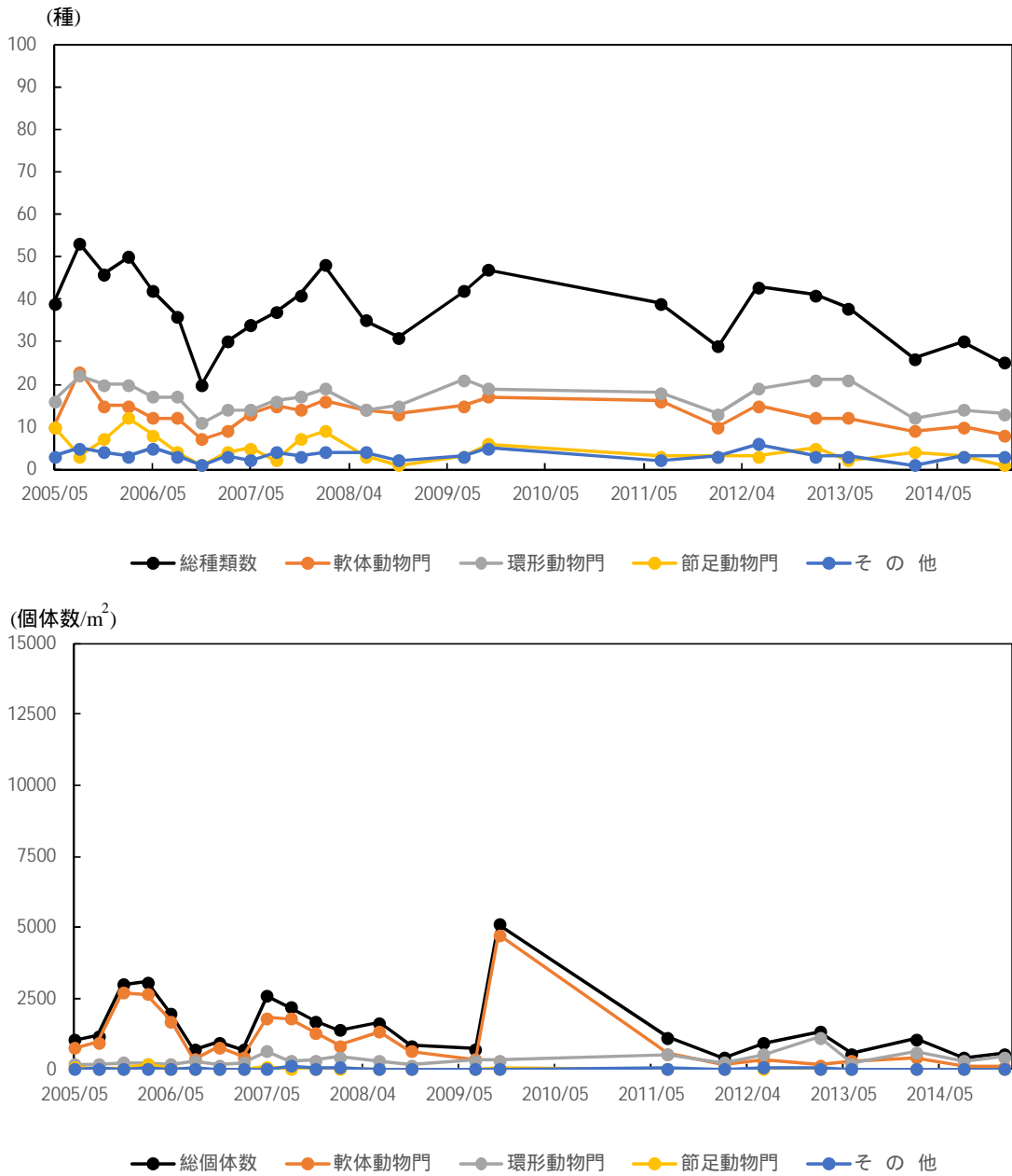
図 4(2) A 1 海域におけるベントスの推移 (Asg-3)
