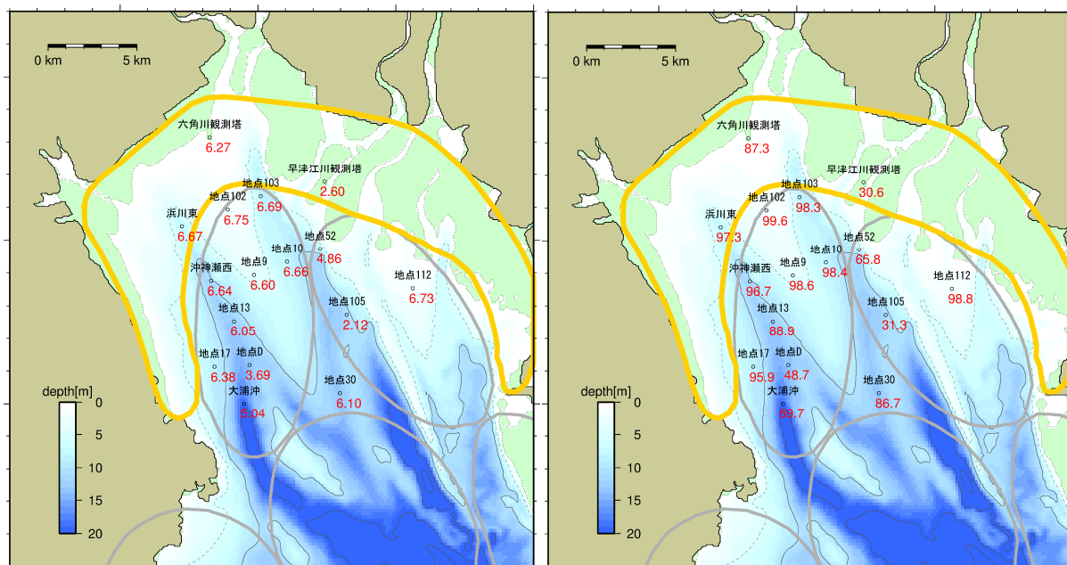
図9 埋没測定板の粒度組成 (左図: Md、右図: 粘土シルト含有率(%))
