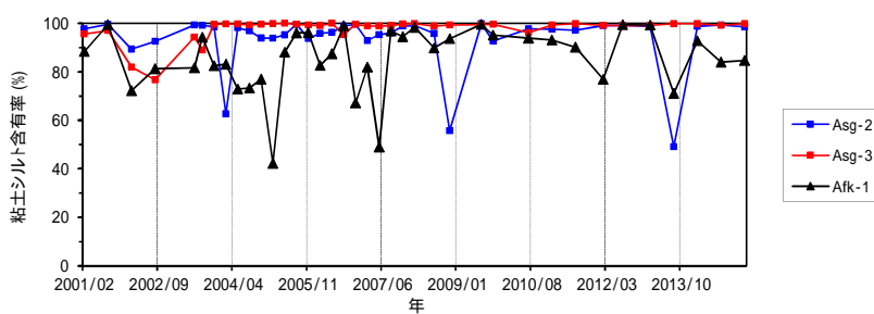
図5 A1海域における底質の推移
