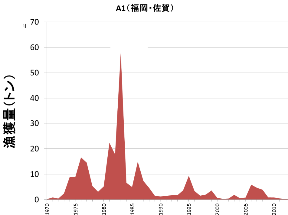
図 16 A 1 海域のアサリ漁獲量の推移
