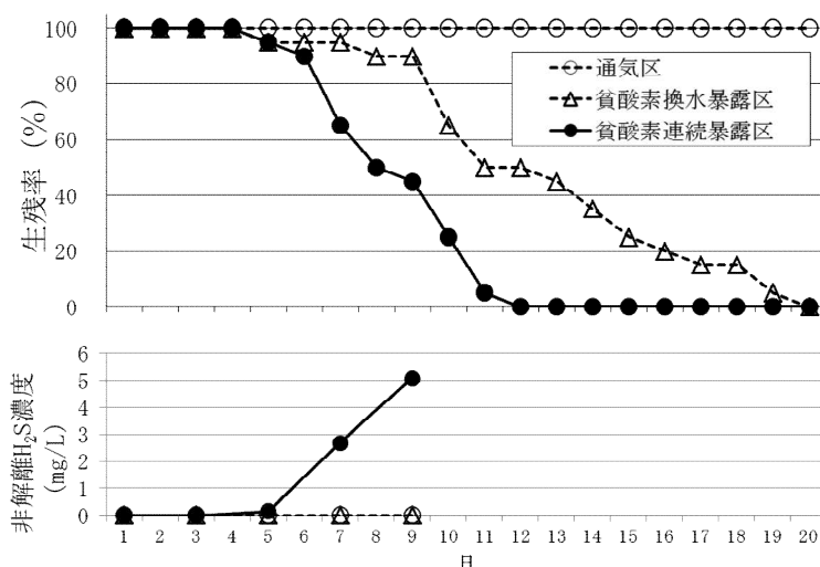
図 14 サルボウの貧酸素曝露実験結果（佐賀県有明水産振興センター提供資料）
