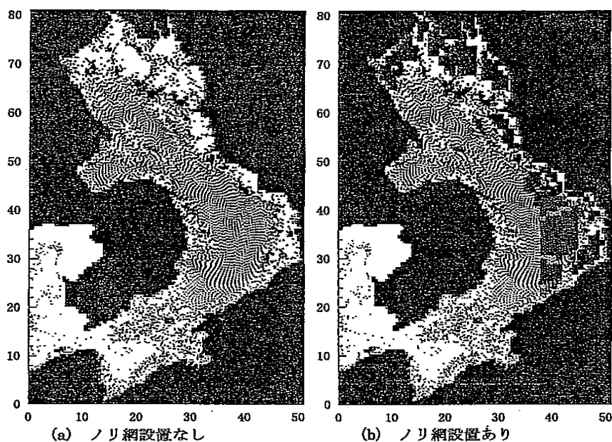
図 17 ノリ網設置の有無による流況変化（粒子追跡開始 3 潮汐後）
