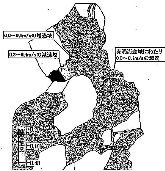
図 16 最大潮流速度の偏差分布 (潮受堤防の影響)
