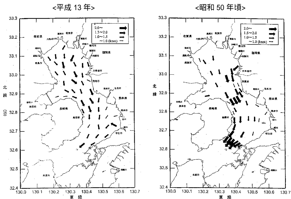
図12 平成13年と昭和50年頃の下げ潮時の流速水平分布
