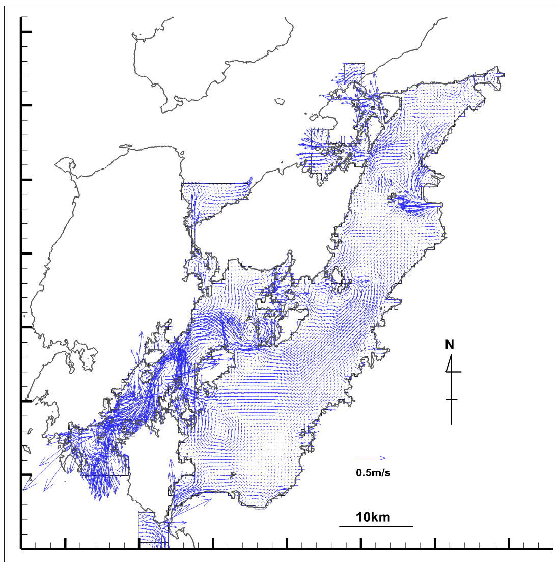
図 18 八代海における表層の平均流(平均的な夏季 1 ヶ月間：8 月)
