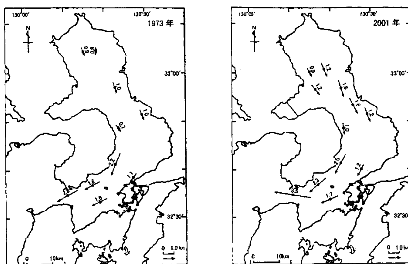
図 10 1973 年と 2001 年の平均大潮時の海面下 3m における下げ潮流の比較
