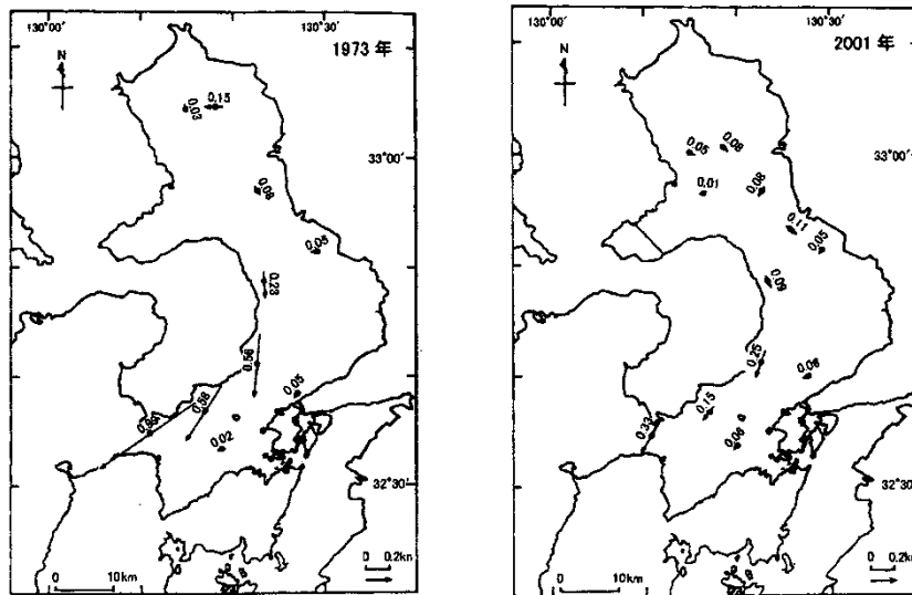
図11 1973年と2001年の15昼夜観測の平均流の比較
