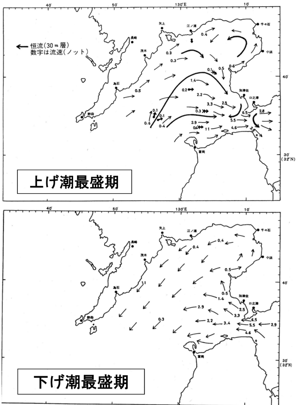
図 19 橘湾における潮流と恒流(30m層)の概況 出典：第 30 回有明海・八代海総合調査評価委員会 資料 3（中田）
