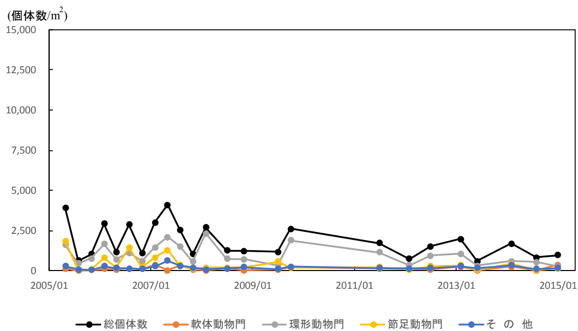
図 4.4.109(3) A7海域におけるベントスの推移(Ang-3)
