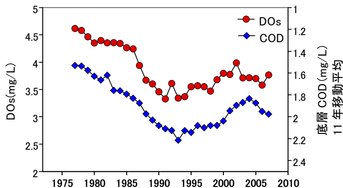
図 4.4.74 有明海湾奥部底層における 11 年間で年々の成層強度変動を除いた溶存酸素量 (DO s ) と 11 年移動平均した COD の経年変化 資料：速水祐一 (2007)：有明海奥部の貧酸素水塊，海洋と生物，第 173 号，pp. 577-583 を改変
