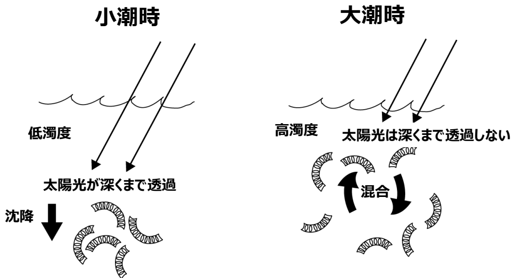
図 15 有明海における Eucampia zodiacus による赤潮の発生機構(概念図)。Ito et al. (2013)をもとに作成。
