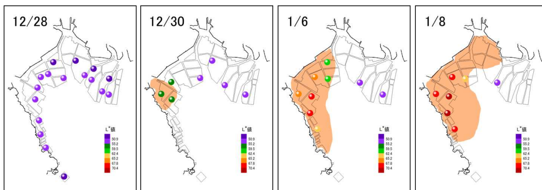
図 17 有明海佐賀県海域における Asteroplanus karianus による赤潮の発生海域とノリの色落ち状況の推移(2011 年度)
