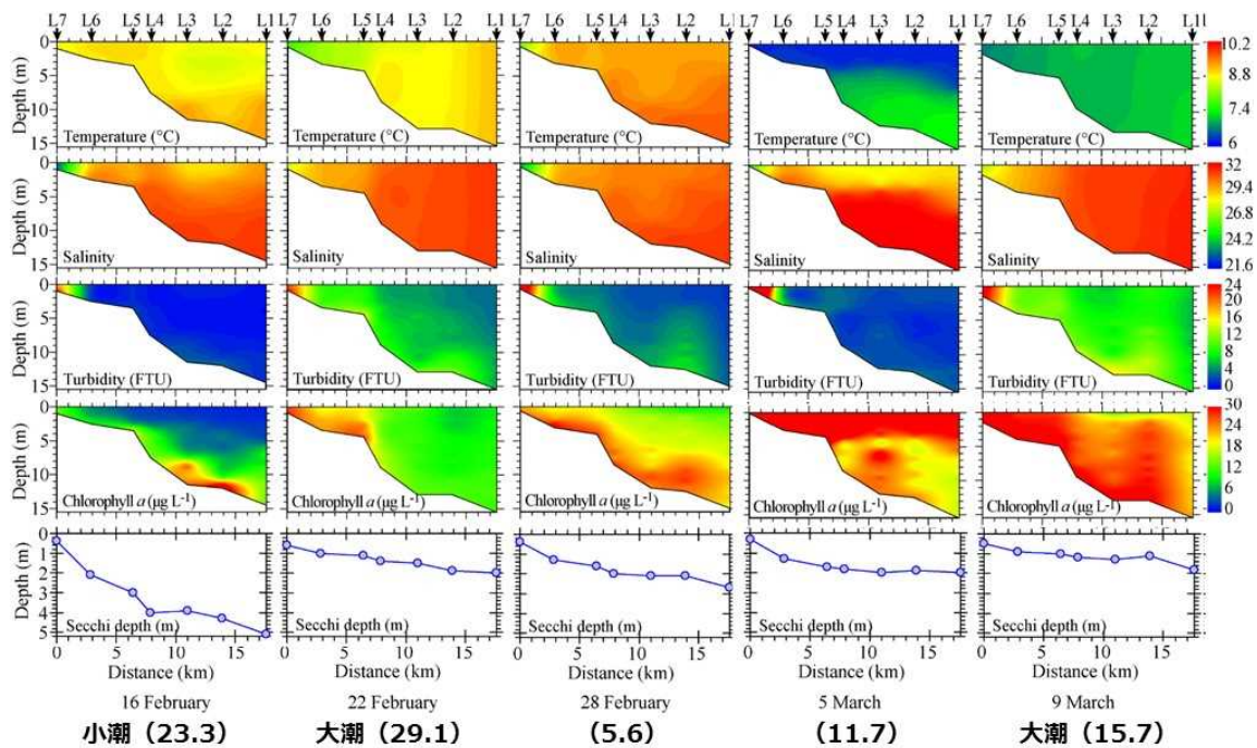
図 14 有明海湾奥部の観測定線における水温、塩分、濁度、クロロフィル a 濃度の鉛直分布および透明度の経時変化(2012年2月~4月)。Ito et al. (2013)より引用。
