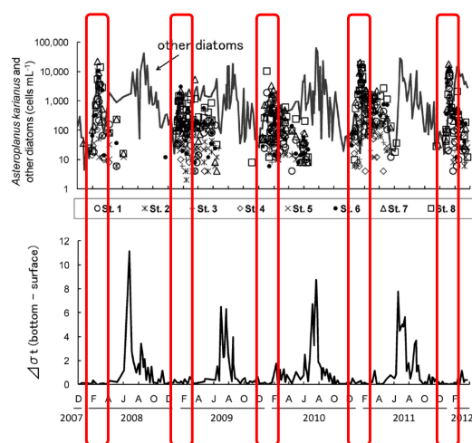
図 19 有明海佐賀県海域表層における珪藻類の細胞密度と鉛直安定度 \Delta\sigma_t の推移（2007年12月～2012年3月）。松原ら（2014）をもとに作成。
