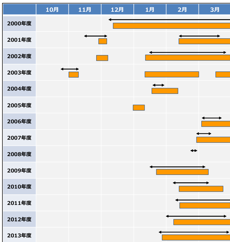
図 9 有明海福岡県海域におけるノリの色落ちの発生期間(■)と珪藻赤潮の発生期間(矢印)
