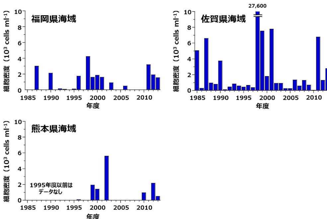
図 12 有明海福岡県海域、佐賀県海域および熊本県海域における Eucampia zodiacus の最高細胞密度の経年変化
