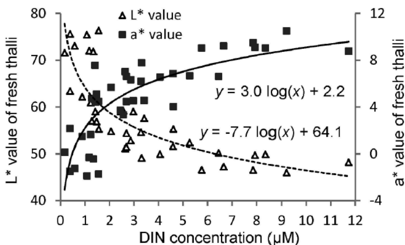
図7 備讃瀬戸海域における溶存態無機窒素(DIN)濃度とノリの色調(L*値, a*値)との関係。村山ら(2015)より引用。L*値は明るさ、a*値は赤みを示す指標で、ともに色彩色素計などで測定される。
