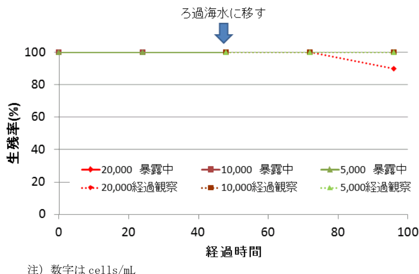
図 4. 4. 106 アサリの生残に対する培養 Chattonella antiqua の影響評価
