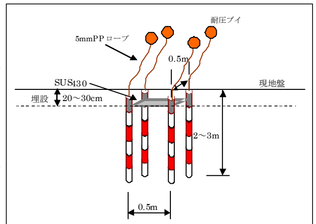
図 4.4.67 埋没測定板の装置の概要
