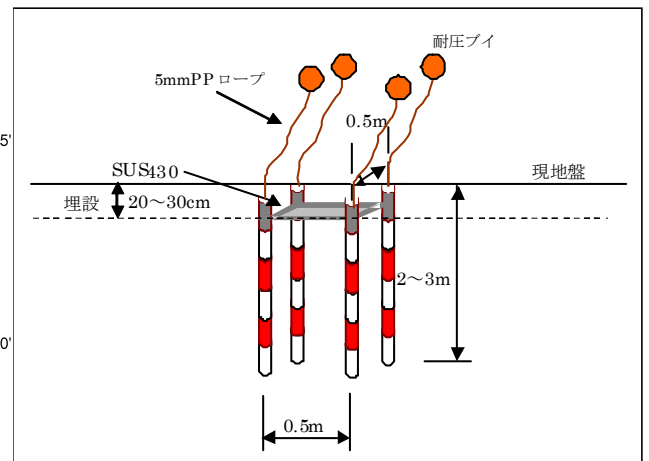
図 4.4.33 埋没測定板の装置の概要
