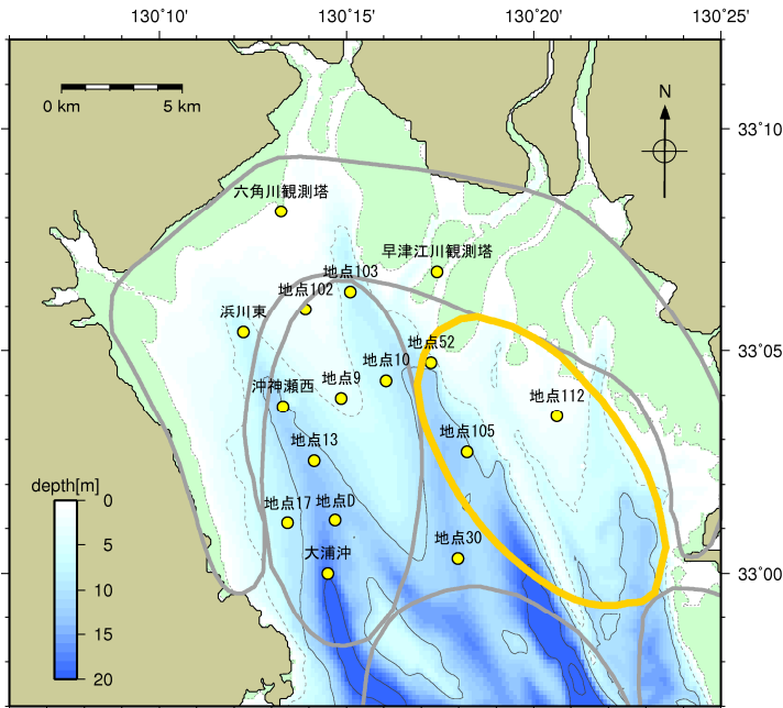
図 4.4.32 埋没測定板の設置地点
