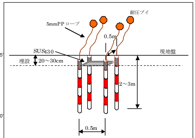
図 4.4.7 埋没測定板の装置の概要
