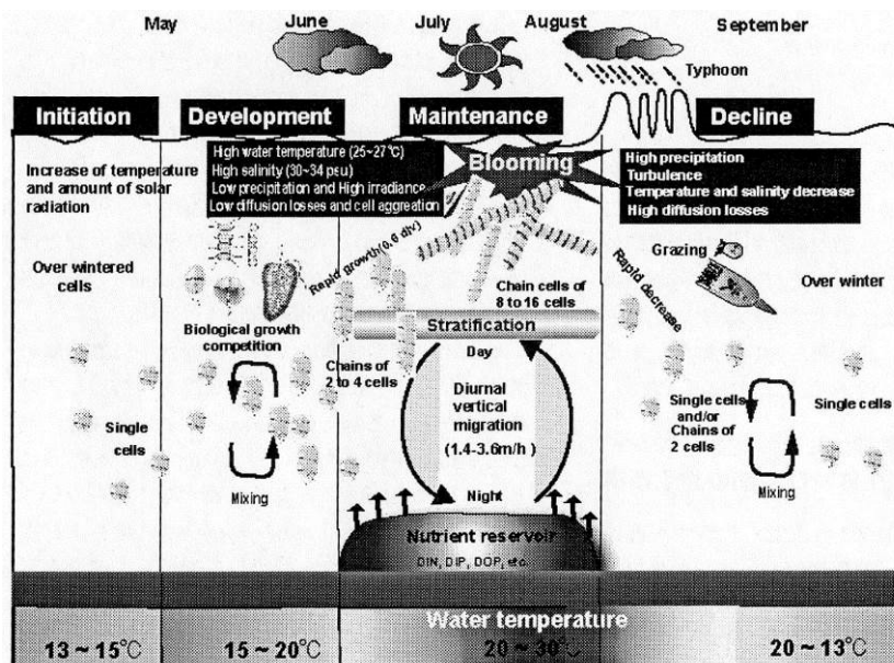
図 3.8.8 八代海における Cochlodinium polykrikoides の赤潮発生機構模式図
