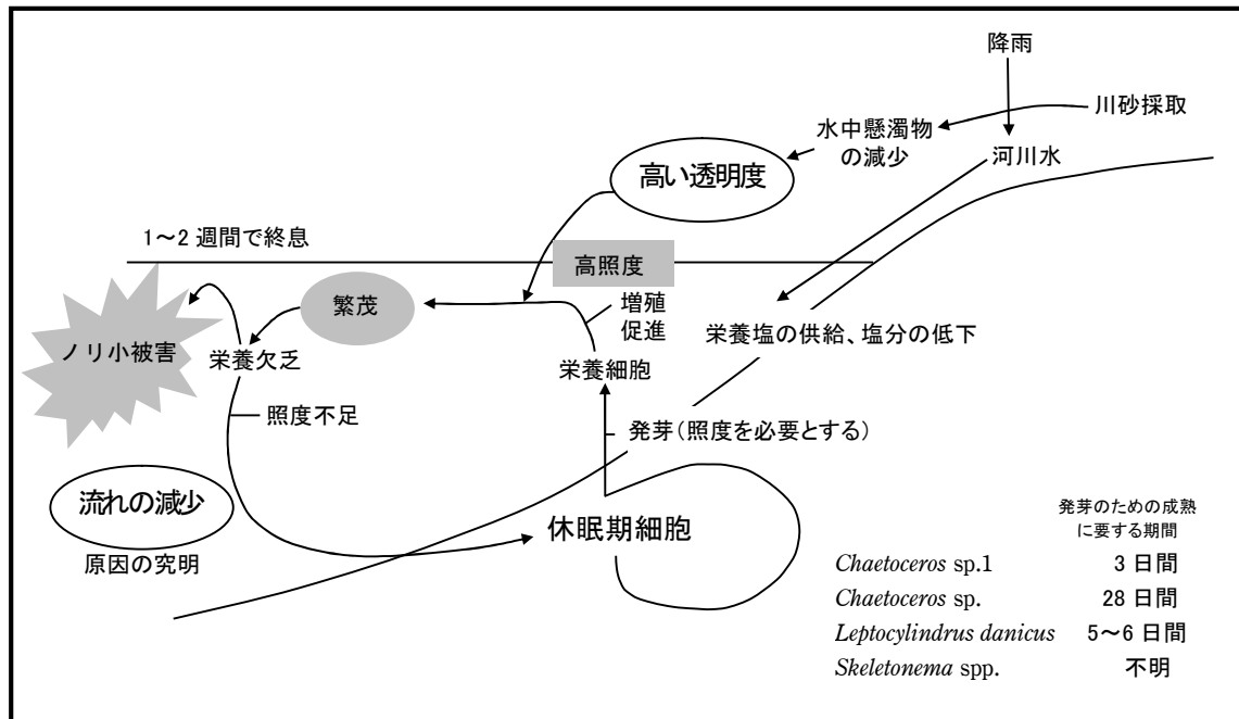
図 3.8.4 小型珪藻の発生機構
