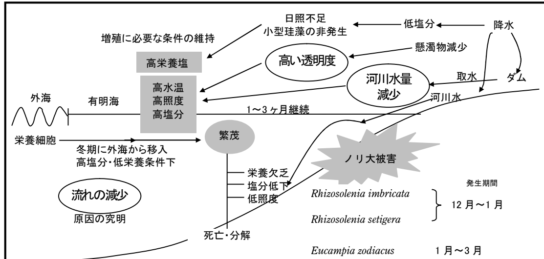
図 3.8.5 大型珪藻の発生機構
