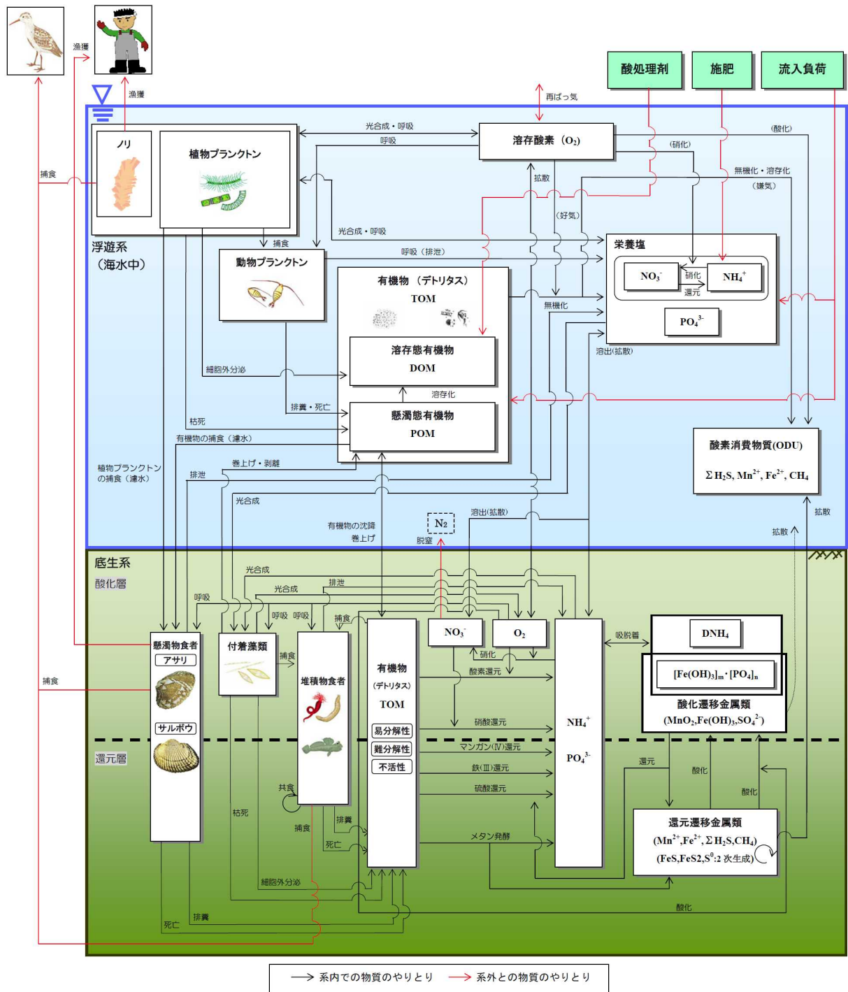
図 2.4 水質サブモデル、底質サブモデル、底生生物サブモデルで考慮する物質循環
