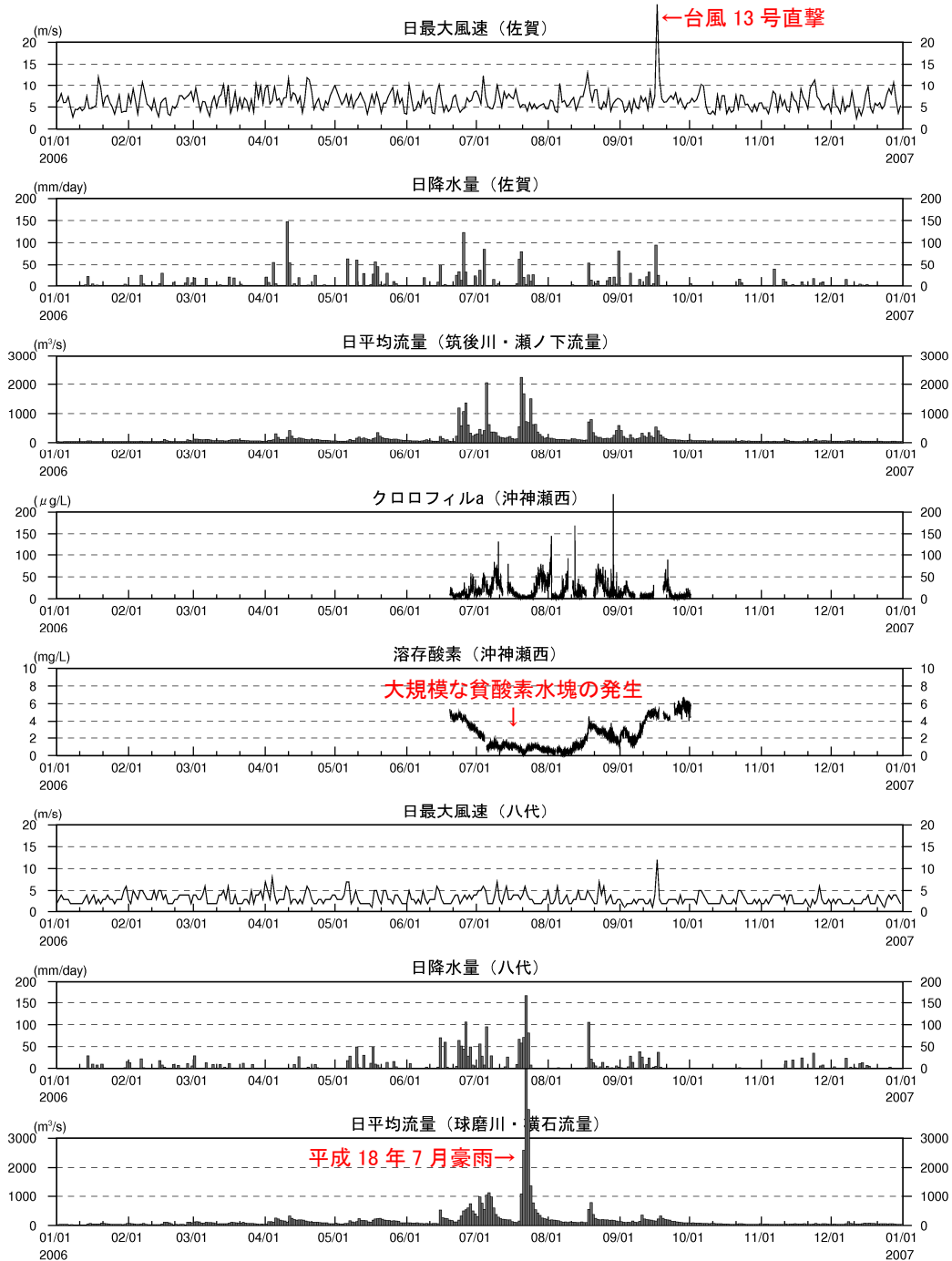
図 2.6 2006 年の気象水文状況とクロロフィル a および DO の時系列
