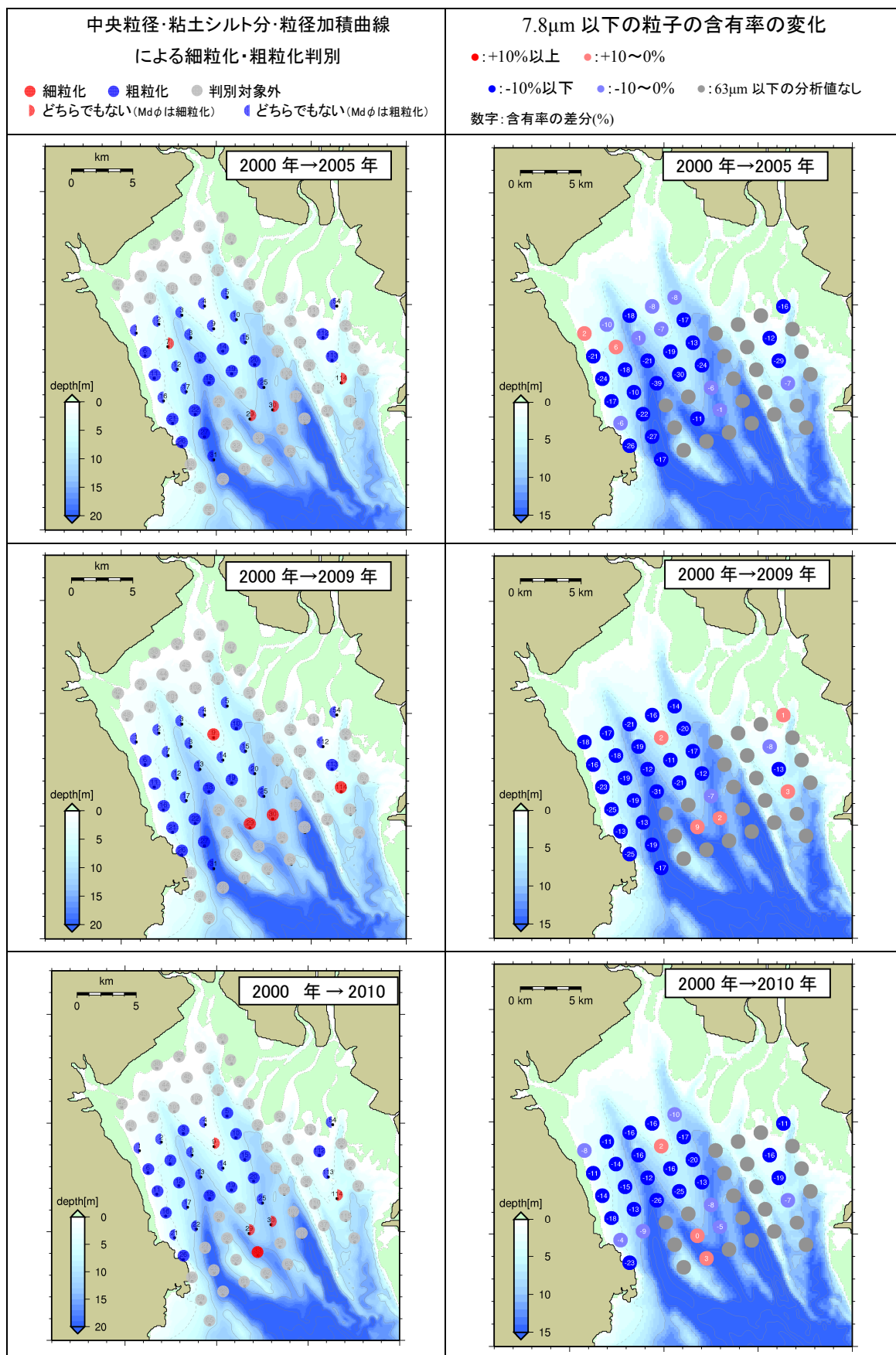
図 4.11 細粒化・粗粒化判別結果と 7.8μm 以下の粒子の含有率の変化 出典：環境省 平成 22 年度有明海・八代海再生フォローアップ調査(懸濁物調査)業務 報告書
