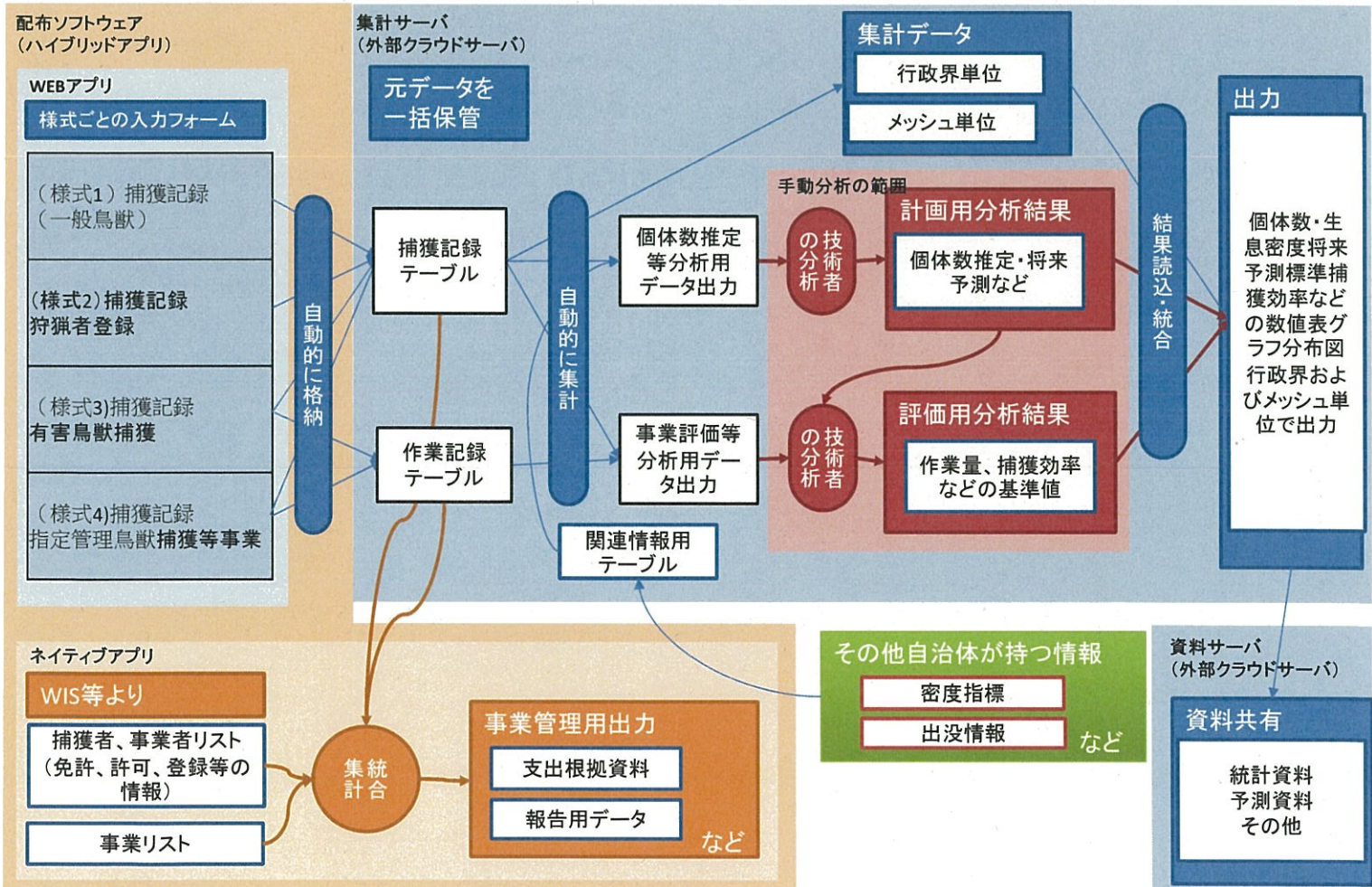
「平成27年度鳥獣の保護・管理に係る科学的情報の収集基盤設計検討業務」システム概要図（入カー出力の流れ）
