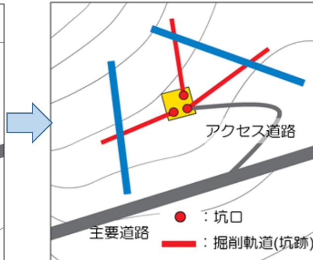
傾斜掘削の場合
