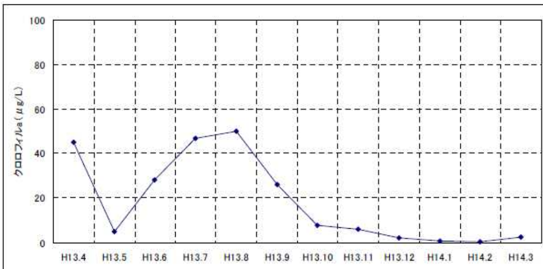
図 3.3.5 相模ダム貯水池のクロロフィル a の経月変化 (平成 13 年度)
