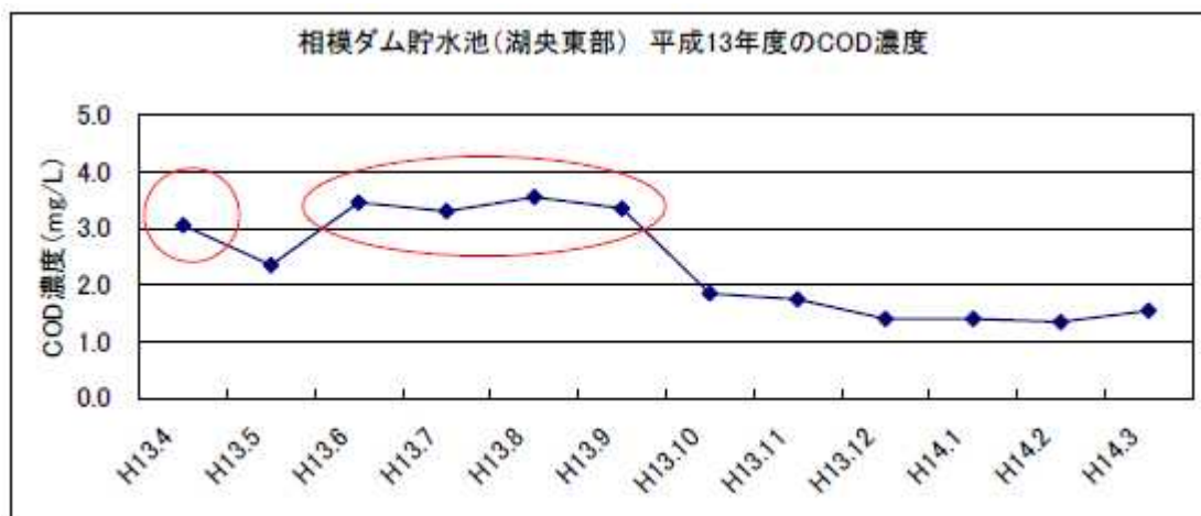
図 3.3.4 相模ダム（湖中央部）のCOD濃度の経月変化（平成13年度）
