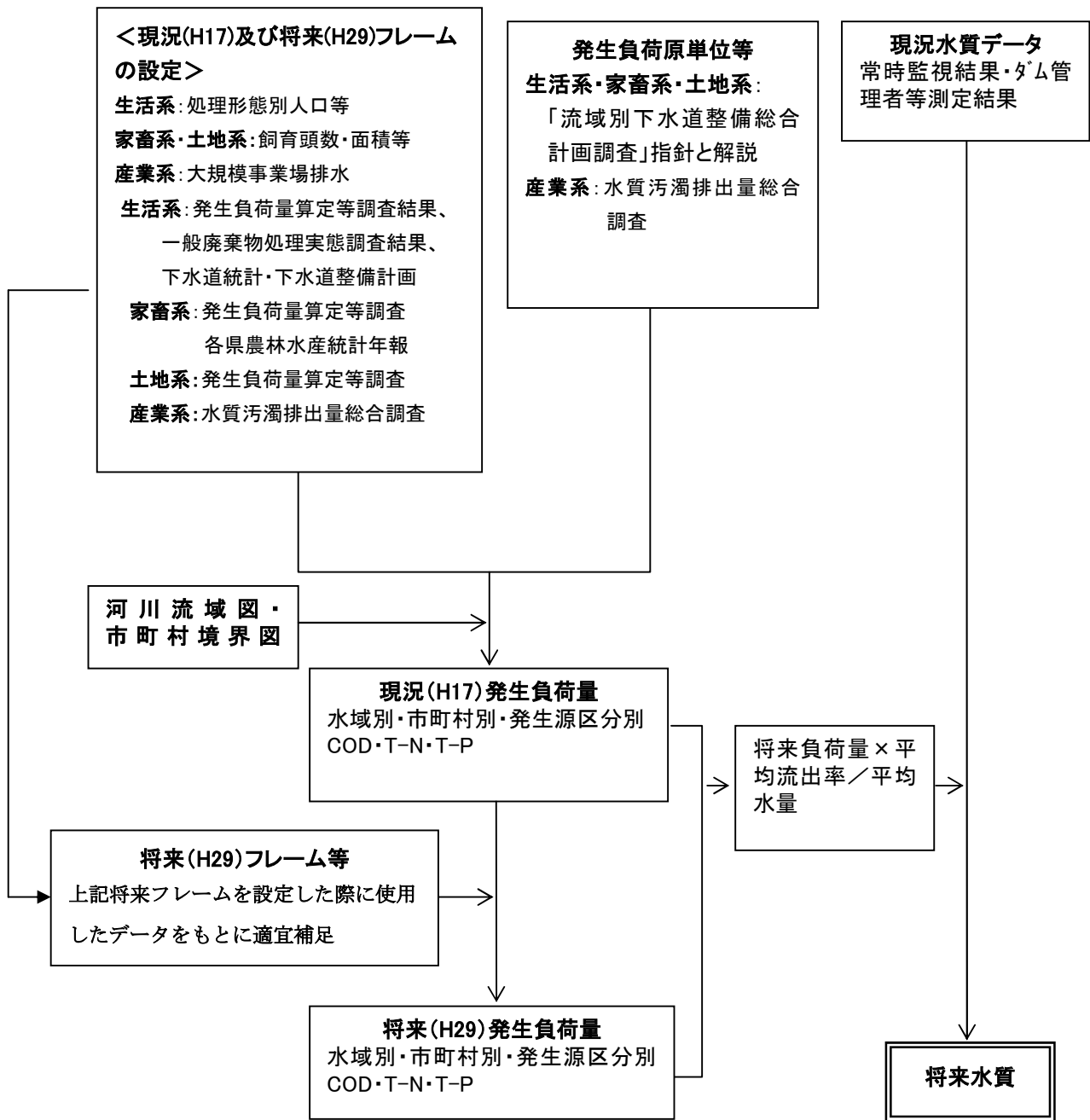
図 6.1 水質汚濁負荷量の算定及び将来水質予測手法の概要
