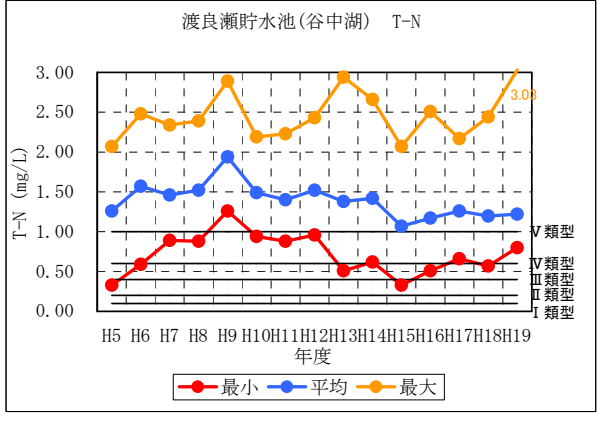
図 4.1 渡良瀬貯水池(谷中湖)における水質の推移
