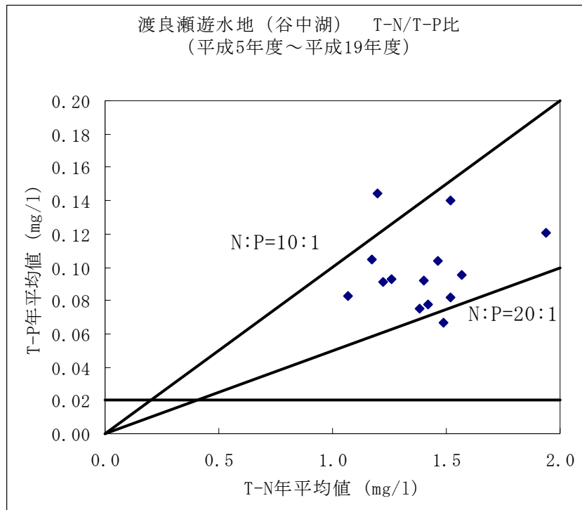
図 4.2 渡良瀬貯水池（谷中湖）N/P 比の状況
