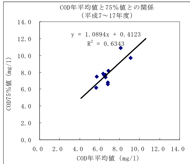
図 7.1 渡良瀬貯水池（谷中湖）のCOD年平均値と75%値との関係
