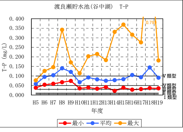
図 4.1 渡良瀬貯水池(谷中湖)における水質の推移
