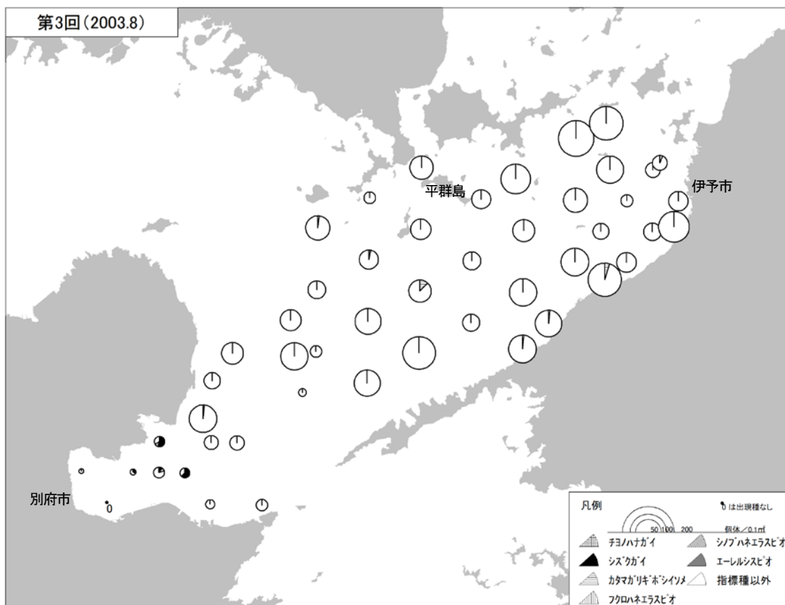
図 2-45(1) 伊予灘 底生生物個体数(汚濁指標種及び汚濁指標種以外別:個体/0.1m 2 )
