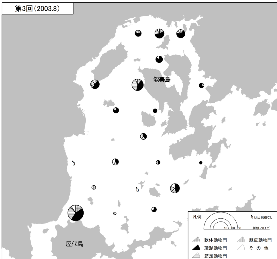
図 2-35 (1) 広島湾 底生生物種類数(分類群別)
