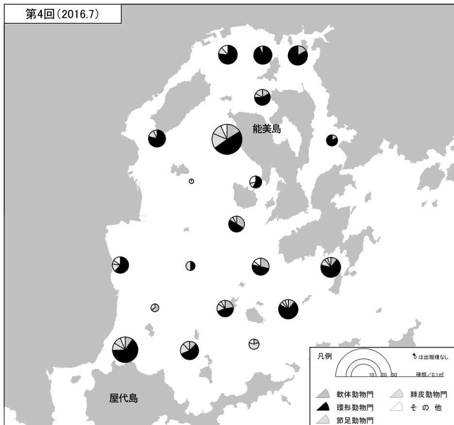
図 2-35(2) 広島湾 底生生物種類数(分類群別)
