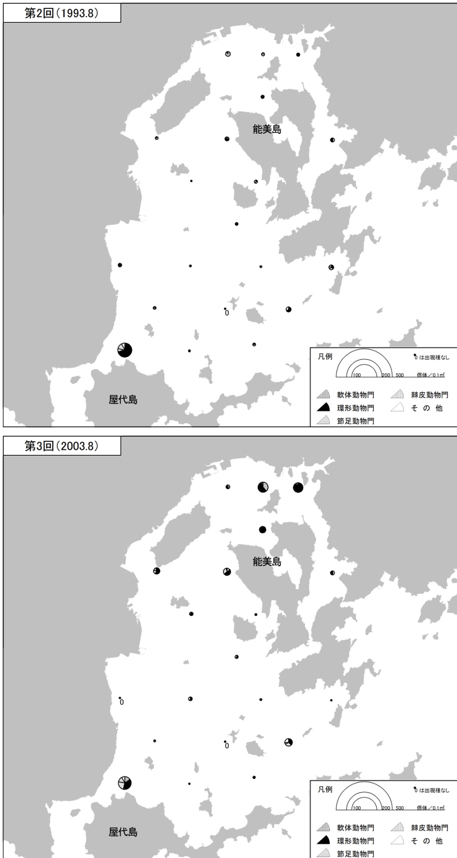
図 2-36(1) 広島湾 底生生物個体数(分類群別:個体/0.1m 2 )
