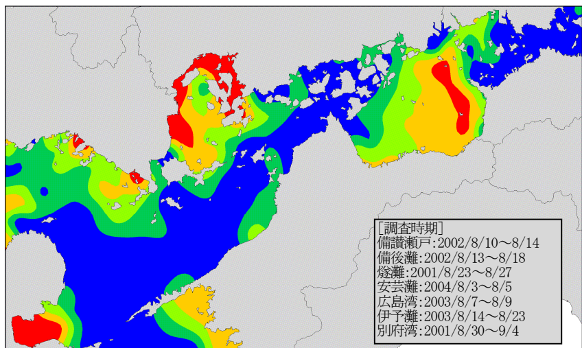
図 1-5(6) TOC(mg/g)の水平分布の変化
