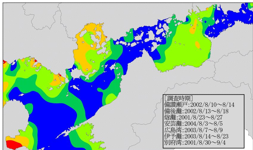
図 1-5(5) COD(mg/g)の水平分布の変化
