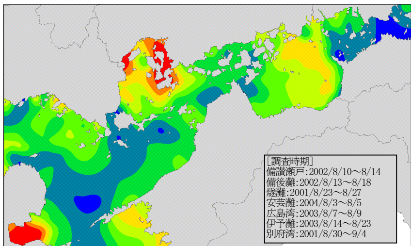
図 1-5(4) IL(%)の水平分布図の変化
