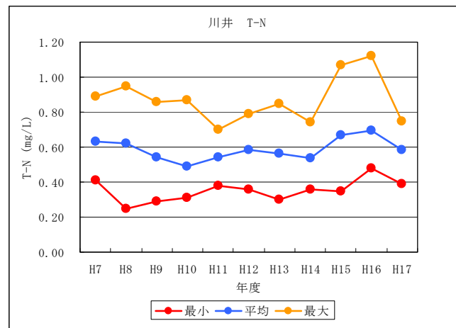
図 5.19 土師ダム貯水池流入水質 (T-N) の推移
