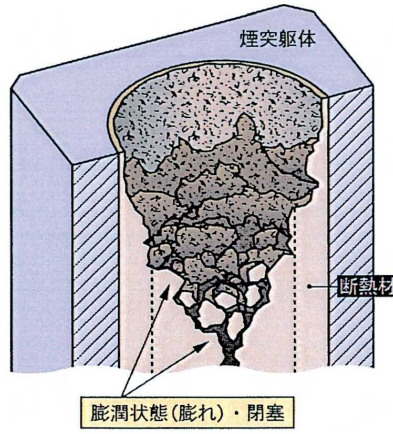
膨潤，閉塞
