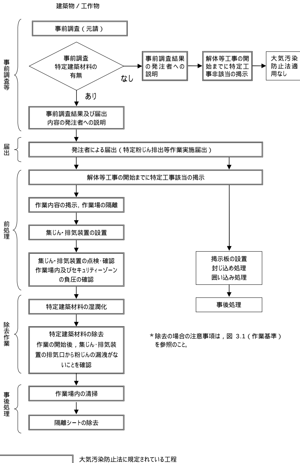
図 3.2 石綿含有吹付け材及び保温材等を掻き落とし、切断若しくは破砕による除去又は封じ込め・囲い込みを行う場合の一般的手順 (改造・補修)
