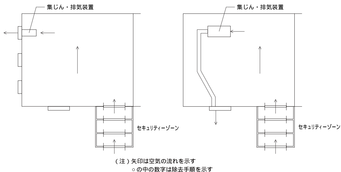
図 3. 48 集じん・排気装置の設置位置（ア）
