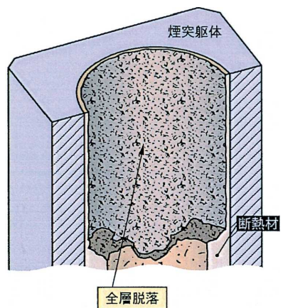
断熱材脱落
