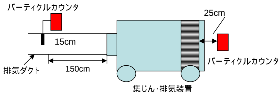
図 3.24 パーティクルカウンタによる測定位置
