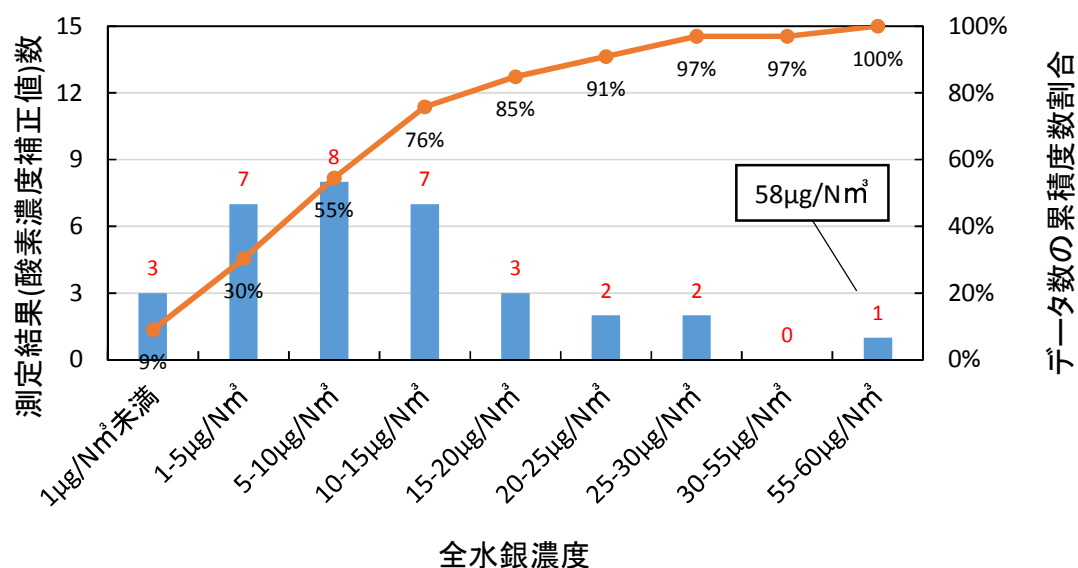
図Ⅱ-4-3-1 排ガス中全水銀濃度 ヒストグラム（下水污泥焼却炉）
