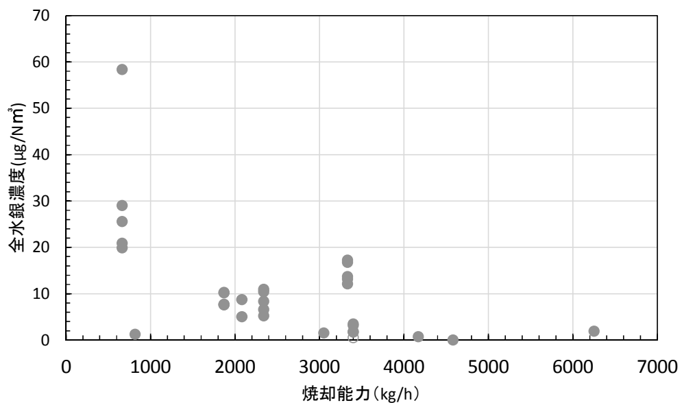
図Ⅱ-4-3-7 焼却能力と全水銀濃度との相関図
