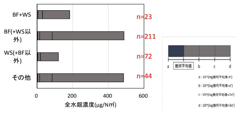
図 II-4-1-8 対数標準偏差による排ガス処理方式と全水銀濃度 (産業廃棄物焼却炉)
