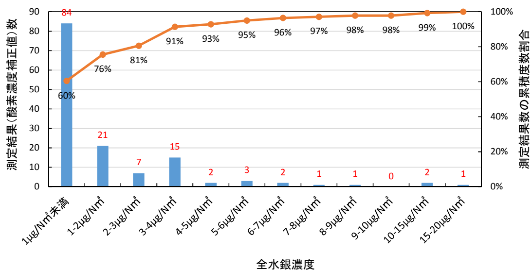
図Ⅱ-1-5 排ガス中全水銀濃度 ヒストグラム (石炭火力発電所及び産業用石炭燃焼ボイラー)
