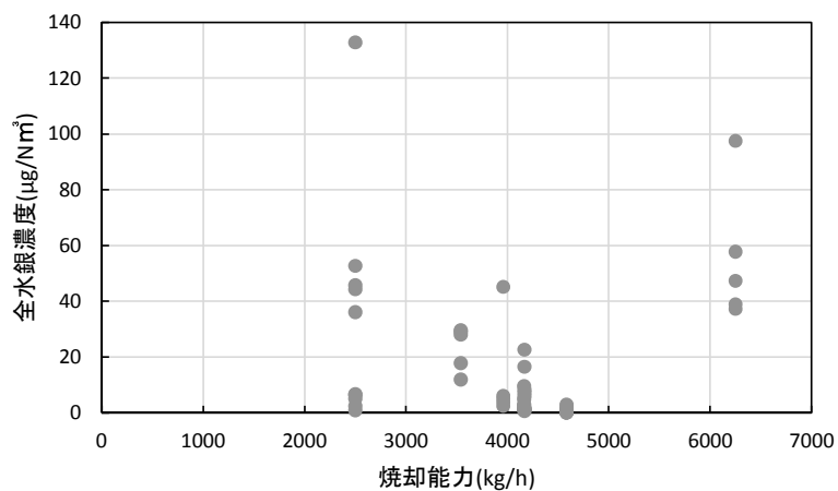
図Ⅱ-4-2-6 焼却能力と全水銀濃度との関係
