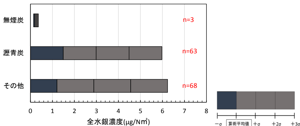
図Ⅱ-1-8 使用石炭の種類と全水銀濃度
