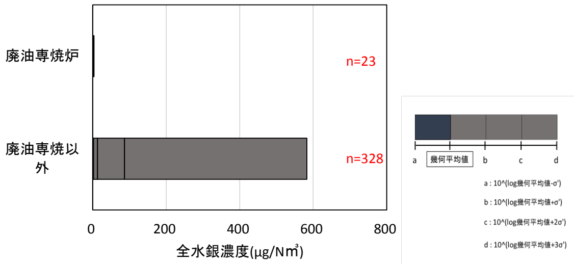
図 II-4-1-8 焼却対象物の種類（廃油）と全水銀濃度（対数標準偏差）
