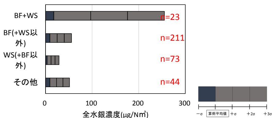
図 II-4-1-2 排ガス処理方式と全水銀濃度（産業廃棄物焼却炉）
