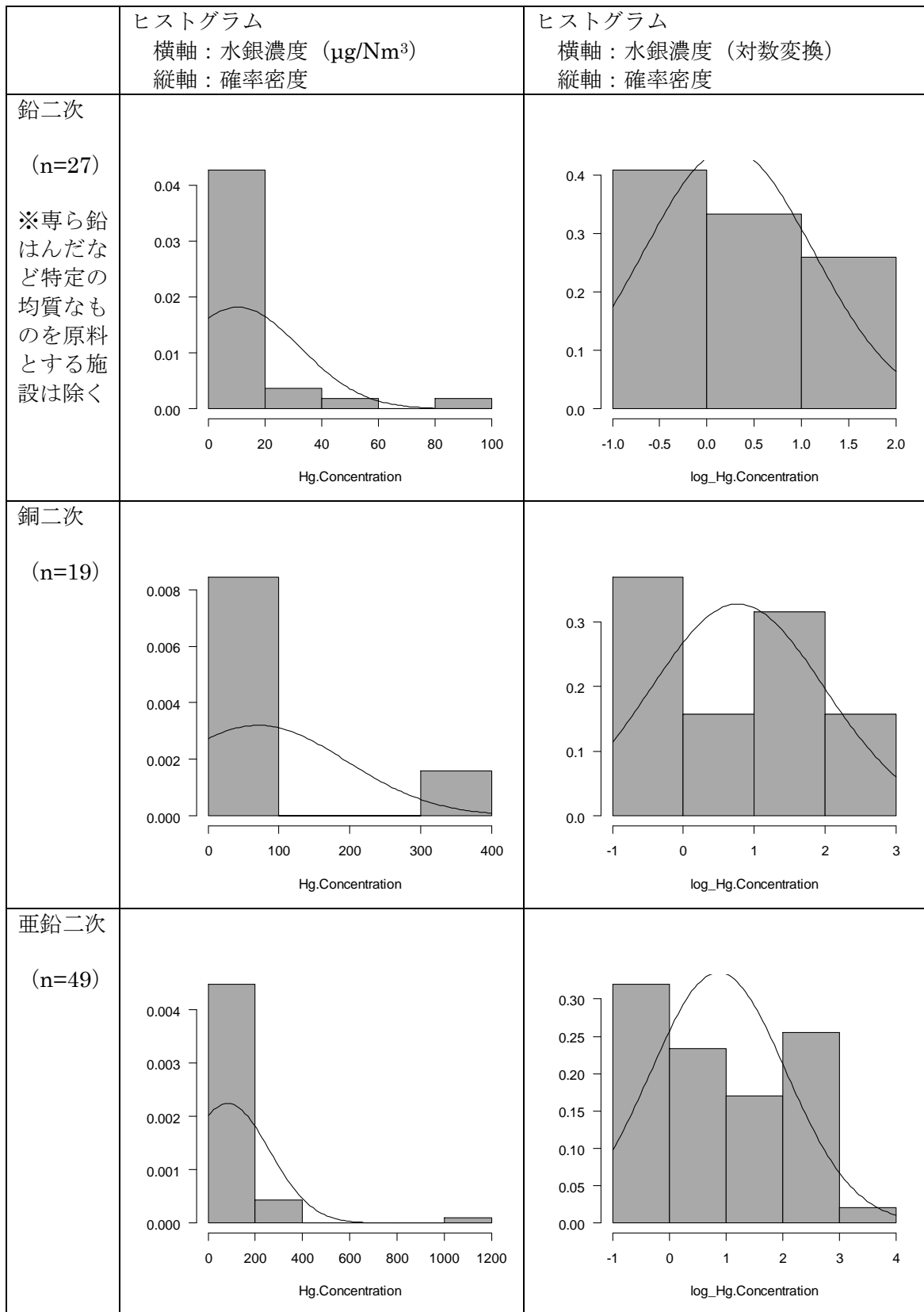
図Ⅲ-2-3 排ガス中の水銀濃度（全水銀）のヒストグラム（非鉄二次施設）（1/2）
