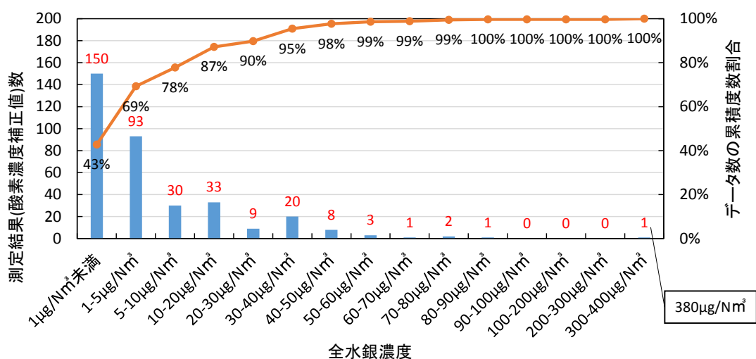
図 II-4-1-1 排ガス中全水銀濃度 ヒストグラム（産業廃棄物焼却炉）
