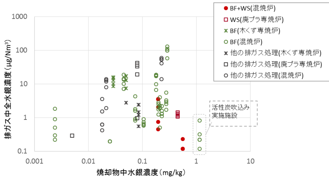
図 II-4-1-4 排ガス処理設備ごとの焼却物中水銀濃度と全水銀濃度 (産業廃棄物焼却炉)
