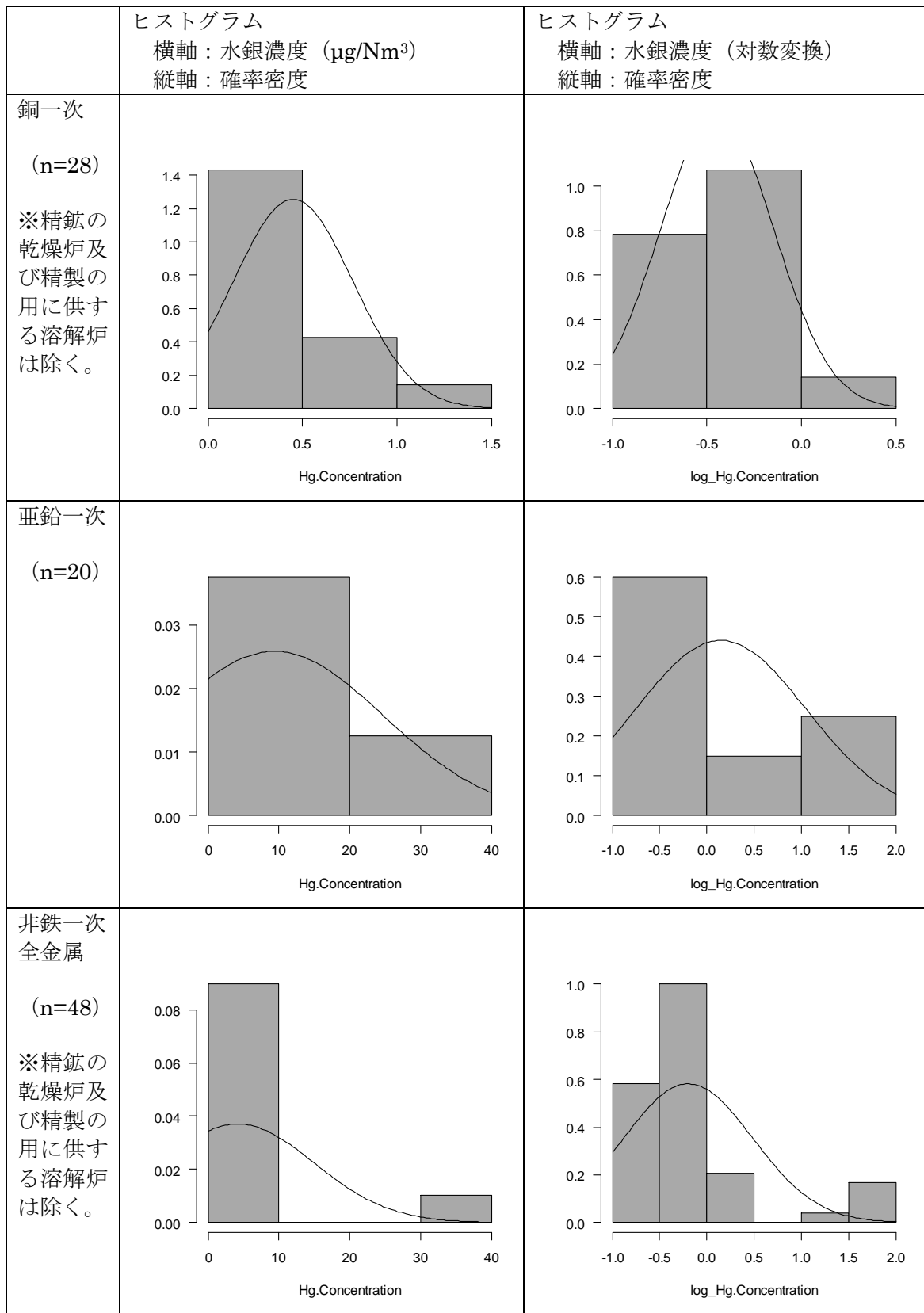
図Ⅲ-2-2 排ガス中の水銀濃度（全水銀）のヒストグラム（非鉄一次施設）
