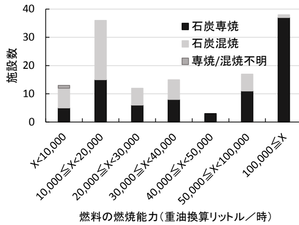
図 II-1-2 燃料の燃焼能力による規模分布
