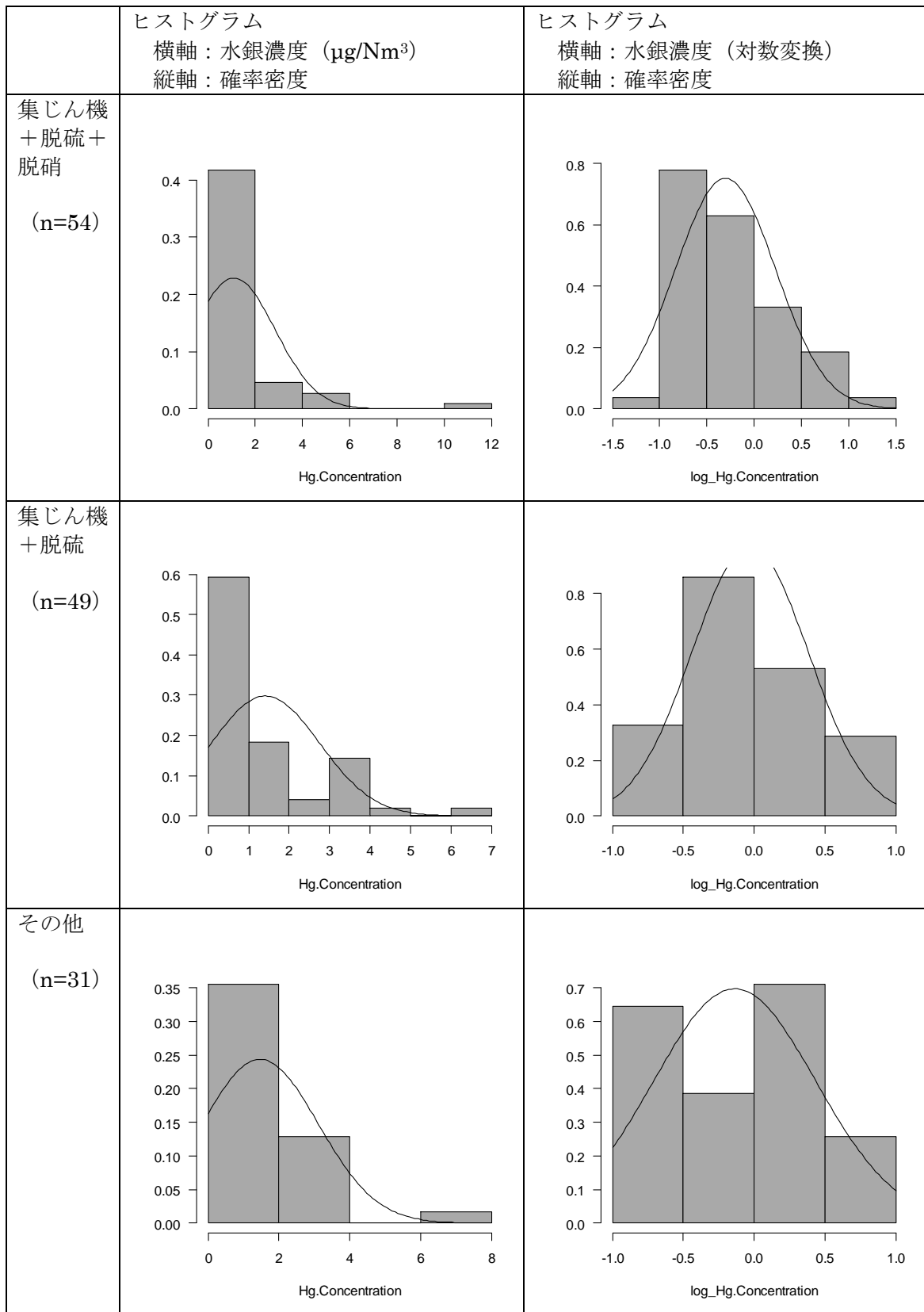
図Ⅲ-2-1 排ガス中の水銀濃度（全水銀）のヒストグラム（石炭ボイラー）
