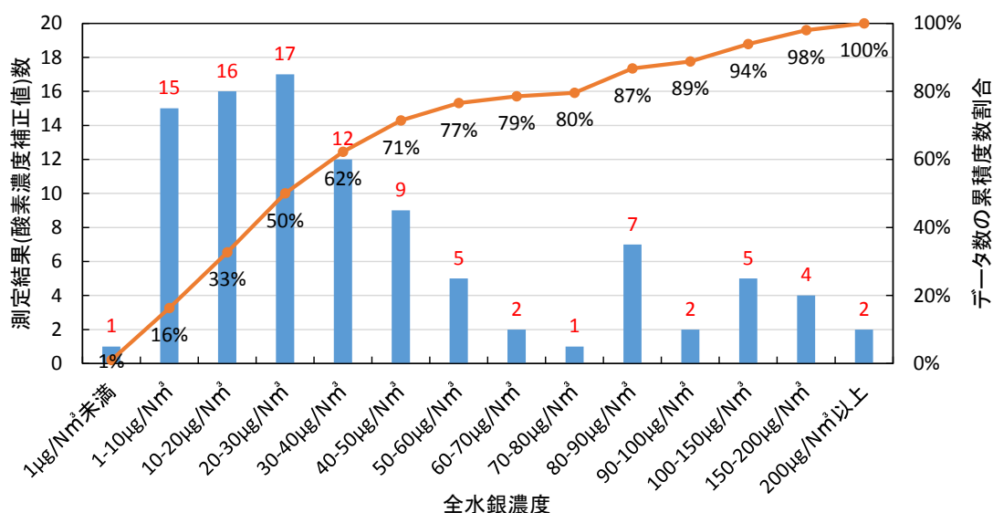
図 II-5-3 排ガス中全水銀濃度 ヒストグラム（セメントクリンカー製造設備）
