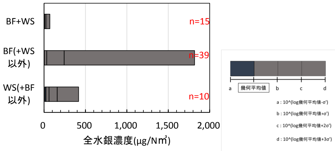
図 II-4-2-3 一般廃棄物焼却炉における排ガス処理施設の種類の全水銀濃度 (対数標準偏差)
