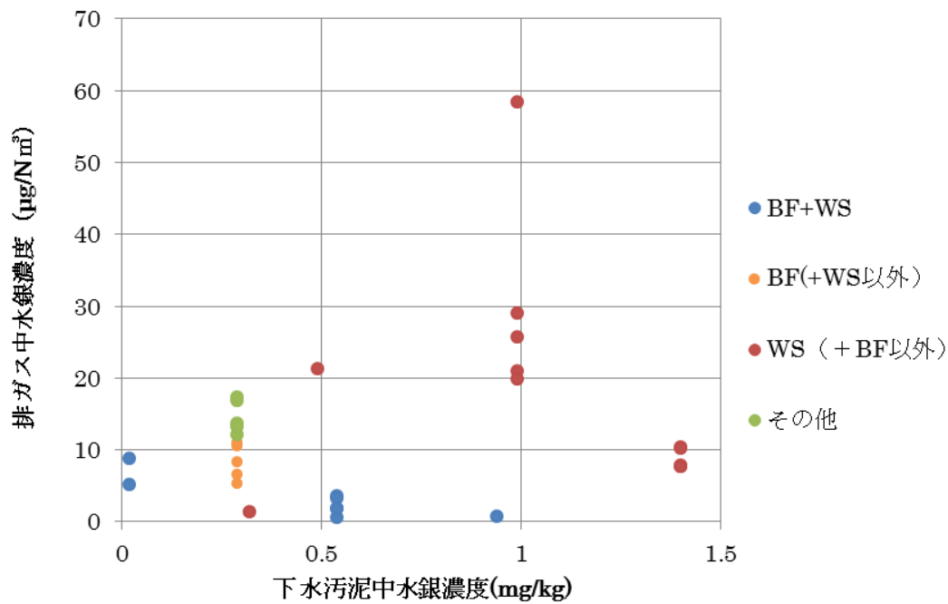
図 II-4-3-4 排ガス処理設備ごとの下水汚泥中水銀濃度と排ガス中水銀濃度
