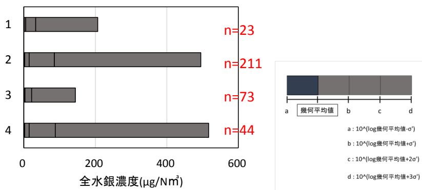
図 II-4-1-3 対数標準偏差による排ガス処理方式と全水銀濃度（産業廃棄物焼却炉）
