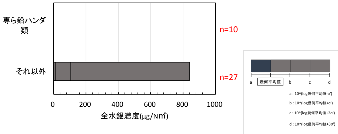
図Ⅱ-3-5 鉛二次施設における原料の種類と全水銀濃度（対数標準偏差による）
