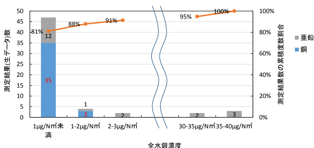
図 II-2-1 排ガス中全水銀濃度 ヒストグラム（一次施設全体）
