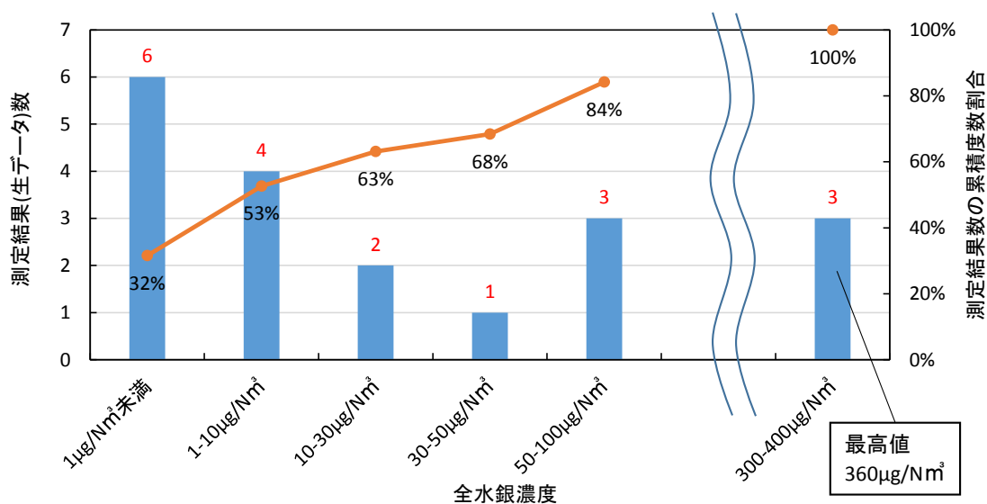
図 II-3-1 排ガス中全水銀濃度 ヒストグラム (非鉄二次施設 銅)
