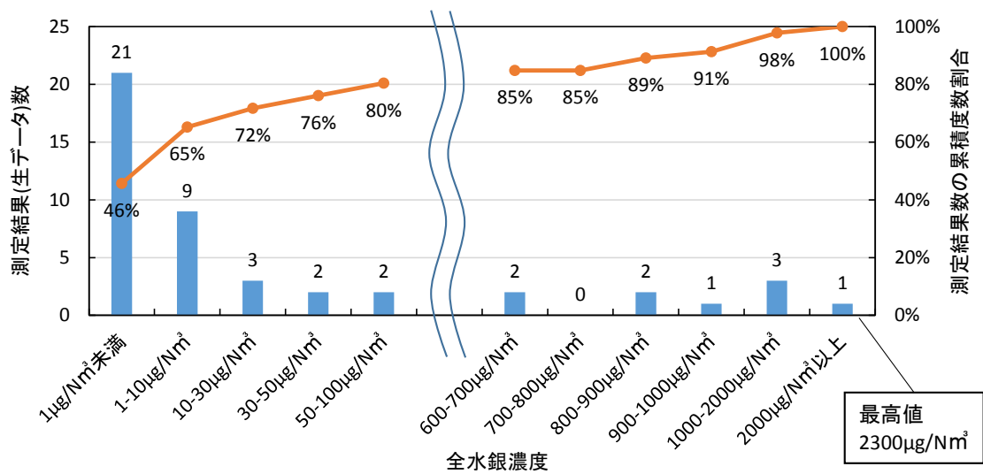
図 II-3-3 排ガス中全水銀濃度 ヒストグラム (非鉄二次施設 鉛)
