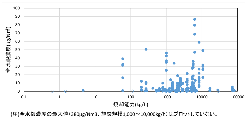
図 II-4-1-9 焼却能力と全水銀濃度（産業廃棄物焼却炉）
