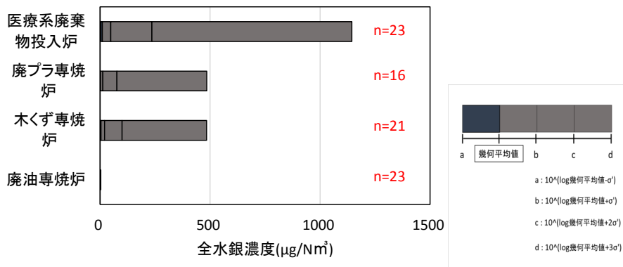
図 II-4-1-6 産業廃棄物焼却炉における焼却対象物の種類と全水銀濃度 (対数標準偏差)
