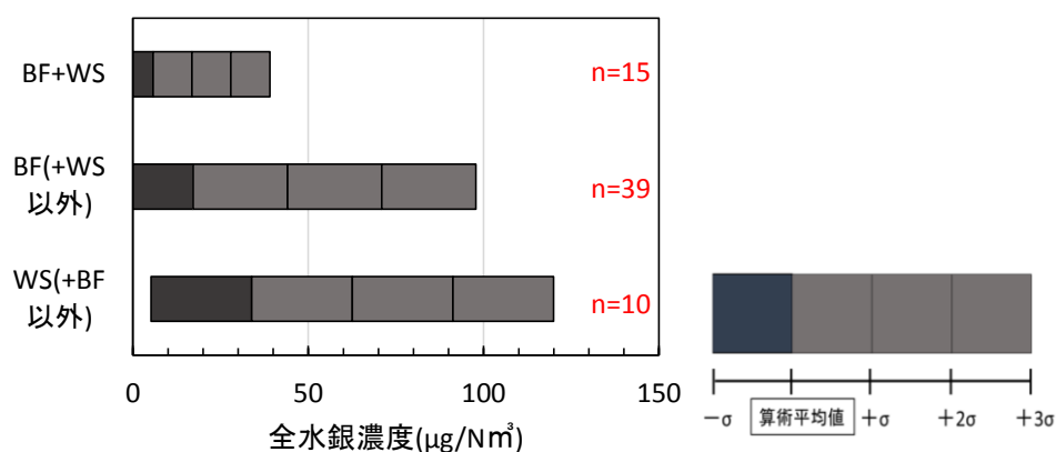
図 II-4-2-2 一般廃棄物焼却炉における排ガス処理施設の種類と全水銀濃度
