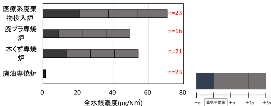
図 II-4-1-5 産業廃棄物焼却炉における焼却対象物の種類と全水銀濃度
