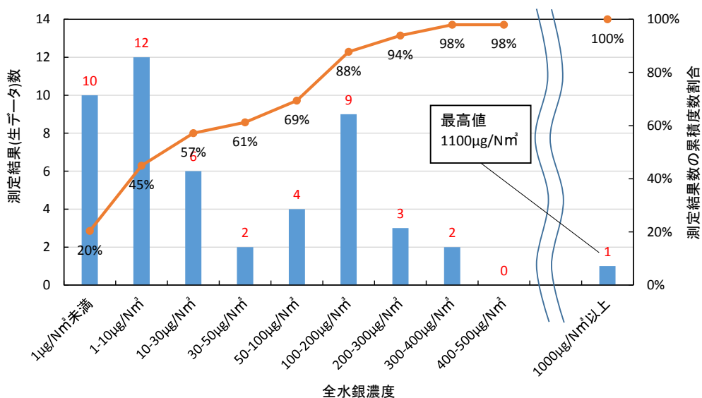
図 II-3-2 排ガス中全水銀濃度 ヒストグラム (非鉄二次施設 亜鉛)
