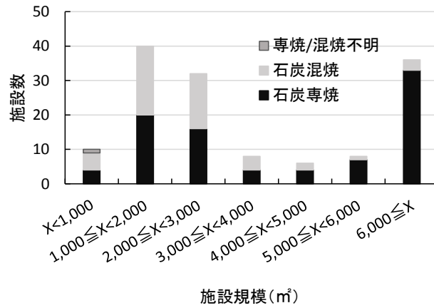
図 II-1-1 伝熱面積による規模分布
