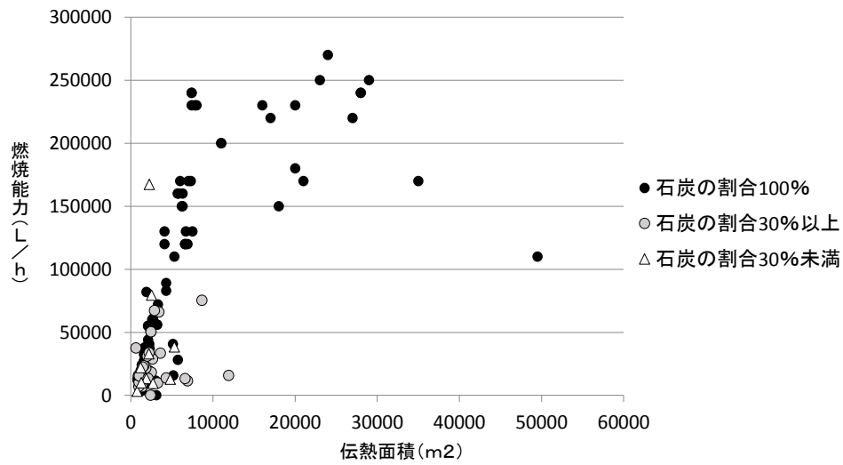
図 II-1-3 燃焼能力と伝熱面積の関係
