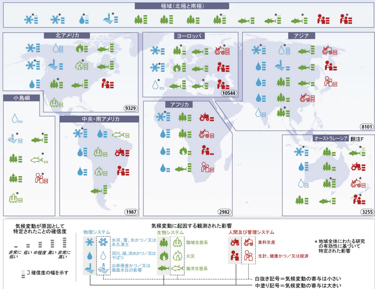
図SPM.4: 第4次評価報告書以降の入手可能な研究に基づく、ここ数十年におけるかなり多くの影響が、今では気候変動に原因特定されている。原因特定には、気候変動が果たす役割について定義された科学的証拠が必要である。気候変動に原因特定される追加的影響がこの地図上に示されていないことも、そのような影響が起きていないことを意味するものではない。気候変動に起因する影響を裏付ける文献は知識基盤の拡大を反映しているが、文献は多くの地域、システム及びプロセスについて未だに限定的であり、データ及び研究におけるギャップを浮き彫りにしている。記号は、気候変動に起因する影響の項目を示しており、観測された影響に対する気候変動の相対的寄与度（大もしくは小）及び気候変動を原因として特定した確信度を示す。各記号は、第2作業部会報告書表SPM.A1の1つあるいはそれ以上の事項を参照しており、関連する地域規模の影響をグループ化している。楕円中の数字は2001～2010年の間に公表された気候変動に関する文献の地域別の総数で、英語による文献を対象とするスコパス文献データベースにおける表題、要旨またはキーワードで言及されている各国名に基づいている（2011年7月現在）。これらの数字は気候変動に関する入手可能な研究文献について地域間を比較する総合的尺度を与えているが、各地域における気候変動影響の原因特定を裏付ける公表文献数を示すものではない。文献を原因特定評価に含めるかどうかに関しては、第2作業部会報告書第18章で定義されているIPCCの科学的証拠の判定基準に従った。極域及び小島嶼に関する研究は隣接する大陸地域のものと一緒に分類している。原因特定の解析で検討された公表文献は、第5次評価報告書の第2作業部会報告書で評価されたより広範に及ぶ文献に由来する。原因特定された影響に関する説明については、第2作業部会報告書の表SPM.A1を参照されたい。 [図1.11]
