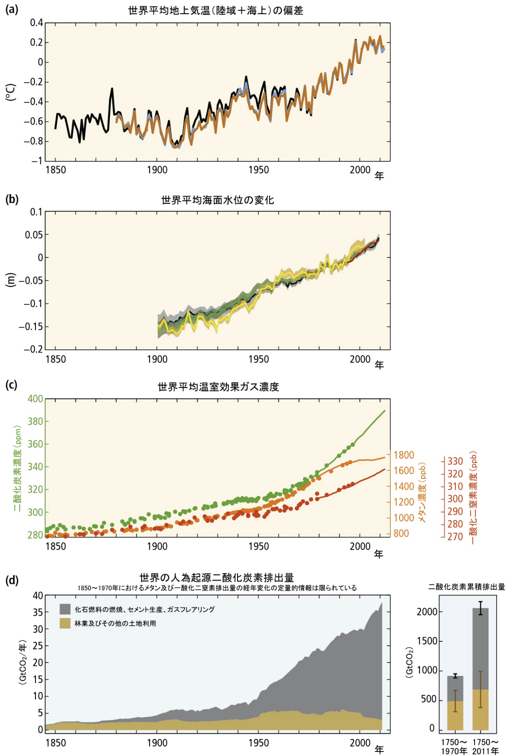
図SPM.1: 観測値(図 (a) (b) (c)、背景は黄色)と排出量(図 (d)、背景は薄青)の複合的な関係は、第1.2節及びトピック1で取り上げられている。世界全体でみた気候システムの観測値と他の指標の変化。観測値: (a) 陸域と海上とを合わせた世界年平均地上気温の1861~2005年平均を基準とした偏差。色付きの線はそれぞれ異なるデータセットを示す。(b) 最も長期間連続するデータセットの1861~2005年平均を基準とした世界年平均海面水位の変化。色付きの線はそれぞれ異なるデータセットを示す。全てのデータセットは、衛星高度計データ(赤)の始めの年である1993年と同じ値になるように合わせてある。不確実性の評価結果がある場合は色付きの陰影によって示している。(c) 氷床コアデータ(点)及び大気の詳細測定(線)による温室効果ガス、すなわち二酸化炭素(CO 2 、緑)、メタン(CH 4 、オレンジ)及び一酸化二窒素(N 2 O、赤)の大気中濃度。指標: (d) 化石燃料の燃焼、セメント生産、ガスフレアリング並びに林業及びその他の土地利用による世界の人為起源二酸化炭素排出量。これらの発生源からの二酸化炭素累積排出量及びそれらの不確実性は、右側にそれぞれ棒グラフとエラーバーで示している。メタンと一酸化二窒素の排出量の蓄積の世界規模での効果は、図(c)に示される。1970~2010年の温室効果ガス排出量データは図SPM.2に示されている。
