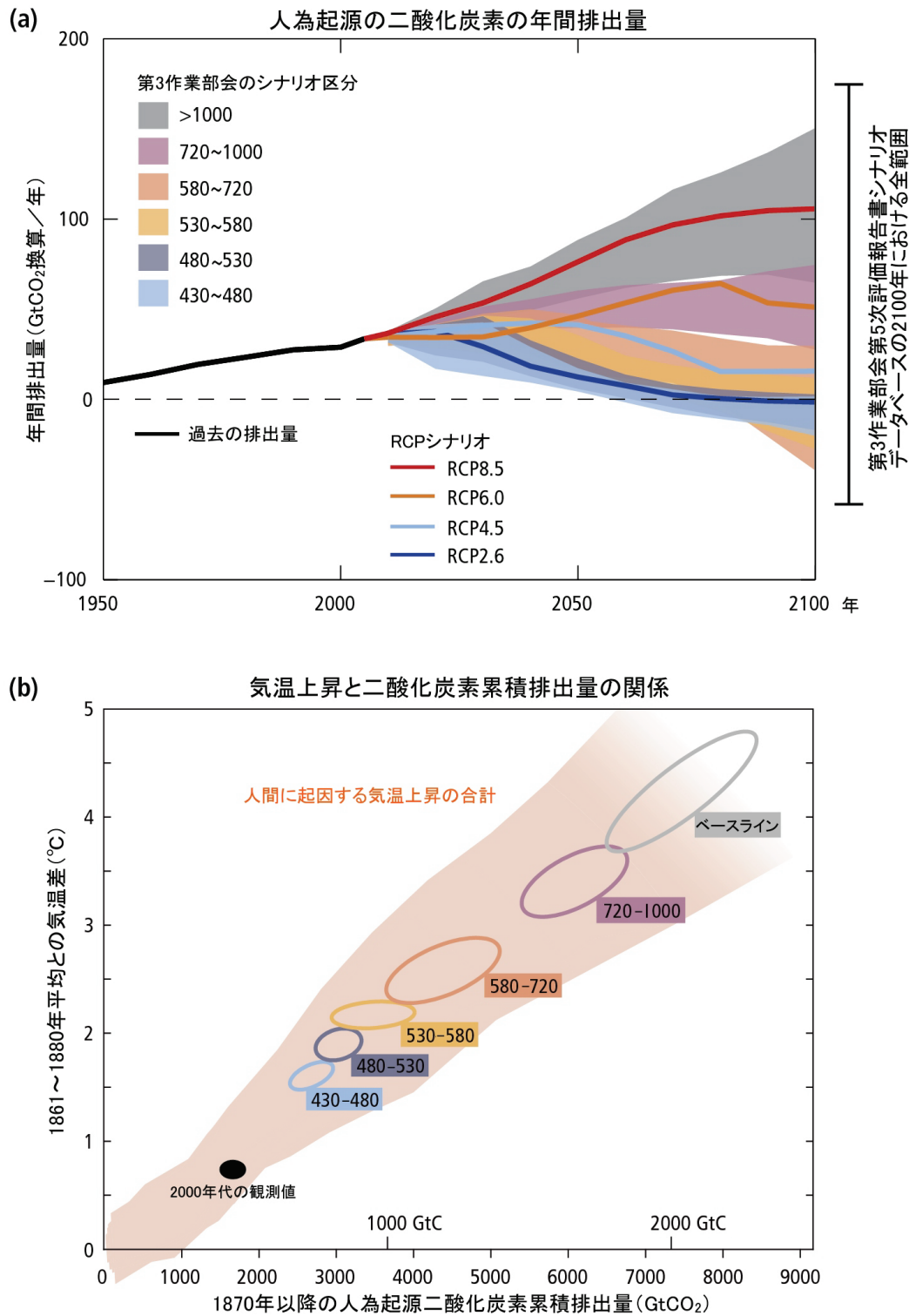
図SPM.5: (a) 代表的濃度経路シナリオ(RCP) (線) 及び第3作業部会で用いられた関連するシナリオ区分における二酸化炭素単独の排出量 (着色部分は5~95%の範囲)。第3作業部会のシナリオ区分は科学文献で公表された広範な排出シナリオをまとめたものであり、2100年における二酸化炭素換算の濃度水準 (単位はppm) に基づいて定義されている。その他の温室効果ガス排出量の時系列は、Box 2.2 図1に示されている。(b) 世界の二酸化炭素排出量がある正味の累積値に到達した時点の世界平均地上気温の上昇を、様々な証拠をもとに、その累積合計値の関数としてデータをグラフに配置した結果。プルーム (煙流) 状の着色域は、過去の排出量と2100年までの期間にわたる4つのRCPシナリオの排出量によって駆動された、様々な階層の気候-炭素循環モデルから得られる過去と将来予測の値の広がりを示し、利用できるモデル数の減少につれて色は薄くなる。楕円は、第3作業部会で使用されたシナリオ区分の下で簡易気候モデル (気候応答の中央値) から得られた、1870~2100年の二酸化炭素累積排出量に対する2100年における人為起源の全気温上昇量を示している。気温の観点における楕円の幅は二酸化炭素以外の気候駆動力が異なるシナリオの影響によって生じたものである。黒で塗りつぶされた楕円は、2005年までに観測された排出量に対する、観測された2000~2009年の10年間の気温を、不確実性とあわせて示したものである。[Box 2.2 図1, 図2.3]
