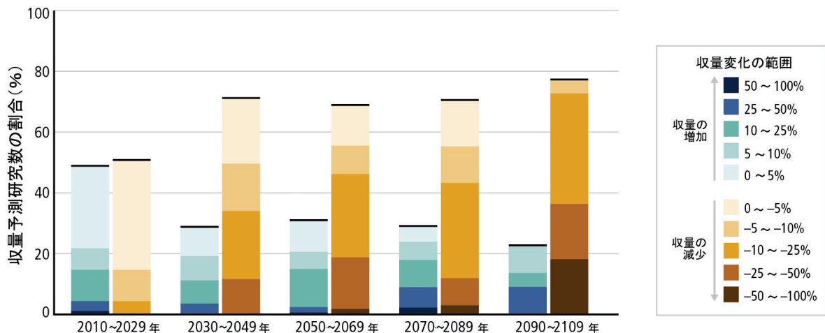
図SPM.9: (a) およそ1000種の魚類及び無脊椎動物の最大漁獲可能量の世界分布変化予測。予測は、乱獲又は海洋酸性化の潜在的影響分析は行わず、中程度から高い程度に温暖化するシナリオ下で単一の気候モデルに基づく海洋の状態を使用して、2001~2010年と2051~2060年の10年平均を比較した。 (b) 21世紀の気候変動による作物収量(大部分はコムギ、トウモロコシ、米及び大豆)の変化予測の図表化。各期間のデータはそれぞれ合計100%となっており、収量の増加及び減少を示す予測数をパーセンテージで示している。図中の予測(1090のデータ点に基づく)には、異なる排出シナリオ、熱帯及び温帯地域、並びに適応が有るケースと無いケースが併せて含まれている。作物収量の変化は20世紀終盤の水準を基準にしている。[図2.6.a, 図2.7]
