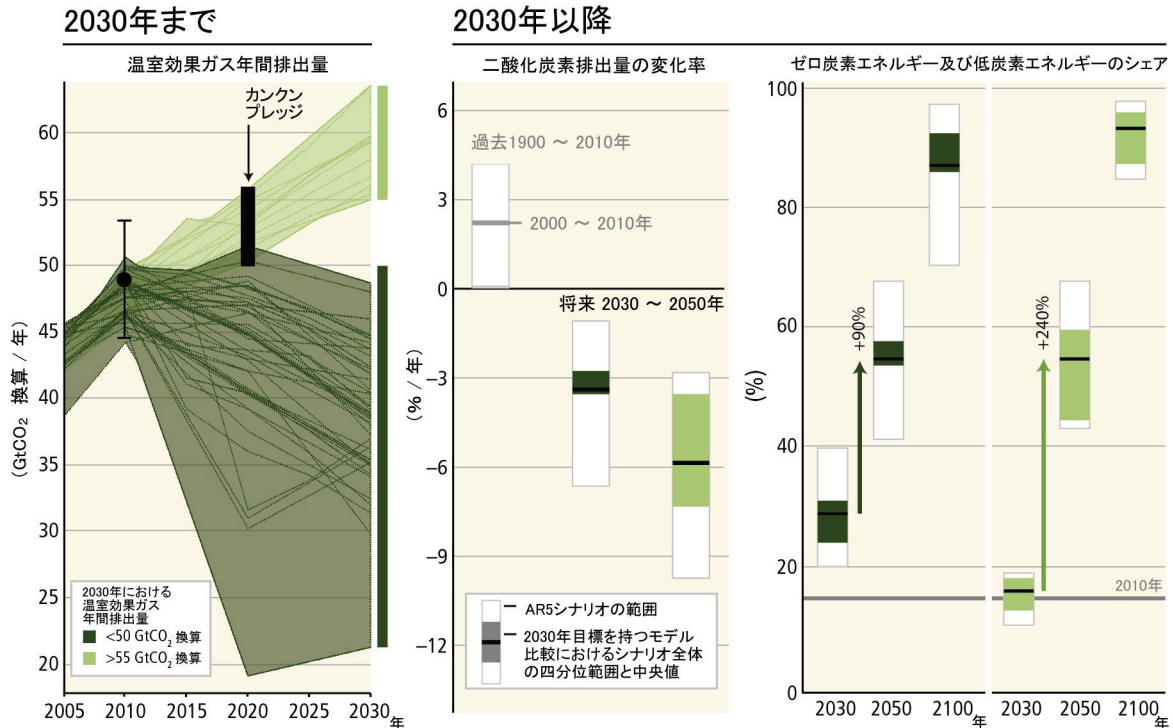
図SPM.12: 21世紀を通じて工業化以前と比べて気温上昇を 2^{\circ}\text{C} 未満に抑えられる可能性が少なくともどちらも同程度の緩和シナリオ（2100年の温室効果ガス濃度が430～530 ppm \text{CO}_2 換算）における、種々の2030年温室効果ガス排出水準と、二酸化炭素排出量削減率及び低炭素エネルギー拡大との関係。これらのシナリオは2030年までの排出水準によってグループ化されている（緑の濃さにより色分けされている）。左の図はそれぞれの2030年水準に達する温室効果ガス排出量（ \text{GtCO}_2 換算/年）の経路を示す。エラーバー付きの黒い丸は、図SPM.2に示した2010年における温室効果ガス排出水準及びその不確実性である。黒い棒は、カンクンプレッジが意味する温室効果ガス排出量の不確実性の範囲を推定したものである。中央の図には、2030～2050年の年間二酸化炭素排出量削減率の平均を示している。この図では、最近のモデル間比較に用いた明確な2030年中間目標を持つシナリオ間の削減率の中央値及び四分位範囲と、第3作業部会第5次評価報告書のシナリオデータベースのシナリオにおける削減率の範囲を対比している。過去の排出量の年変化率（20年間にわたって持続しているもの）と2000～2010年の期間における年間二酸化炭素排出量変化率の平均も同様に示した。右の図の矢印は、2030年の各温室効果ガス排出水準について2030年から2050年にかけてのゼロ炭素エネルギー及び低炭素エネルギーの供給拡大の規模を示している。ゼロ炭素エネルギー及び低炭素エネルギー供給には、再生可能エネルギー、原子力エネルギー及び二酸化炭素回収・貯留（CCS） 訳注S 付き化石エネルギー、あるいはCCS付バイオエネルギー（BECCS） 訳注T などがある。〔注：シナリオのうち、根拠になっているモデルにおいて制限のない緩和技術を最大限用いるポートフォリオを適用（初期設定技術の仮定）しているもののみを示している。世界全体の排出量が正味で大きな負になっている（ >20 \text{ GtCO}_2 換算/年）シナリオ、外生による炭素価格を仮定しているシナリオ及び2010年の排出量が過去の範囲を著しく逸脱しているシナリオは除いてある。〕〔図3.3〕
