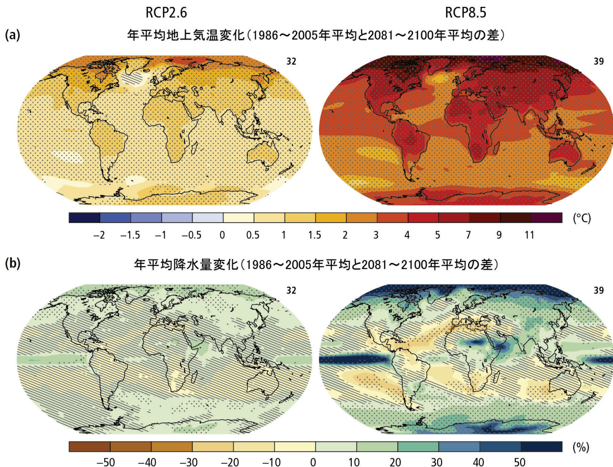
図SPM.7: RCP2.6(左)と RCP8.5(右)のシナリオについて、複数のモデルによる予測を平均した1986～2005年平均に対する2081～2100年平均の年平均地上気温の変化(a) 及び年平均降水量の変化(b)。それぞれの図の右上隅に、複数モデルの平均を算出するために使用したCMIP5のモデルの数を示している。点描影(ドット)は予測された変化が自然起源の内部変動性に比べて大きく、かつ少なくとも90%のモデルが同じ符号の変化をしている領域であることを示す。網掛け(斜線部)は、予測された変化量が自然起源の内部変動性の1標準偏差未満である領域である。{2.2, 図2.2}
