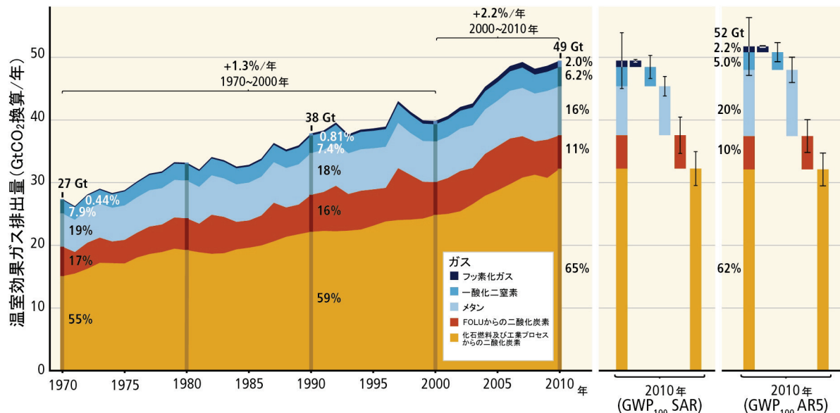
図 SPM.2: 1970～2010 年におけるガス種別人為起源温室効果ガス(GHG)年間総排出量(1 年あたり CO 2 換算ギガ(10 億)トン、GtCO 2 換算/年): 化石燃料の燃焼及び工業プロセス由来の二酸化炭素、林業及びその他の土地利用(FOLU)による二酸化炭素、メタン(CH 4 )、一酸化二窒素(N 2 O)、京都議定書の規定に含まれるフッ素化ガス(F-ガス)。右側には、第 2 次評価報告書及び第 5 次評価報告書による(地球温暖化係数 注 C )値に基づいた二酸化炭素換算排出量の重みづけ係数をそれぞれ用いた 2010 年の排出量を示した。特に明記しない限り、本報告書における二酸化炭素換算排出量 注 D は、第 2 次評価報告書による地球温暖化係数 100 年値(GWP 100 )に基づいて計算された京都議定書対象ガス(二酸化炭素、メタン、一酸化二窒素及びフッ素化ガス)を含んでいる(用語集を参照)。第 5 次評価報告書による最新の地球温暖化係数 100 年値を用いると(右側の棒グラフ)、メタンの寄与が増大するため、温室効果ガス年間総排出量はより大きくなるが(52 GtCO 2 換算/年)、長期変化傾向を著しく変えるものではない。{図 1.6, Box 3.2}
