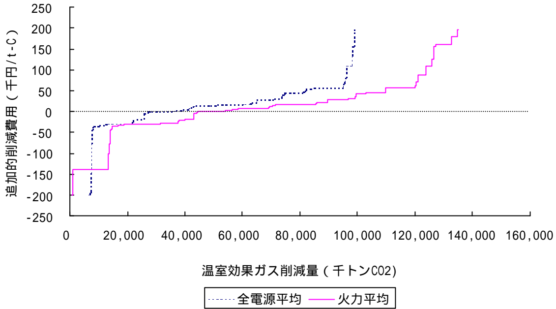
図 5 我が国の温室効果ガス排出削減量と費用の関係
