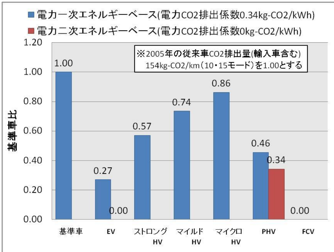
図 4-11 次世代自動車(ガソリン乗用車)CO2 排出量の比較
