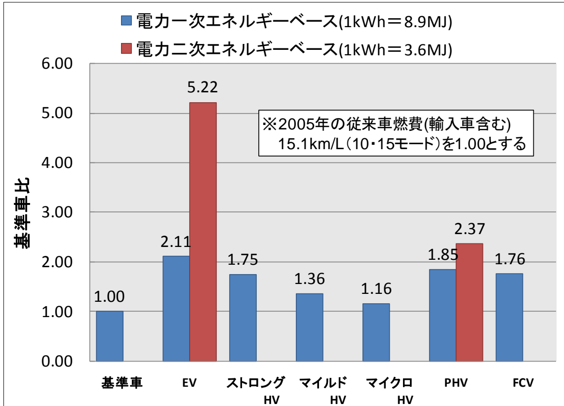
図 4-10 次世代自動車(ガソリン乗用車)効率の比較 (熱量ベース)
