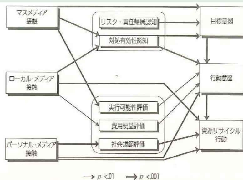
図5-4 3種のメディア接触から資源リサイクル行動にいたる意思決定のパス解析(野波ら,1997より作成)
