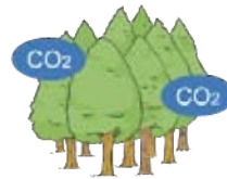
CO 2 吸収源
