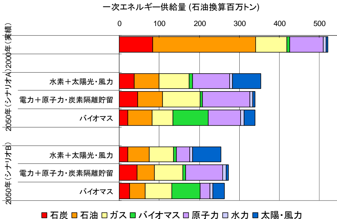
図8 2050年CO 2 排出量70%削減を可能にする供給側エネルギー構成例
