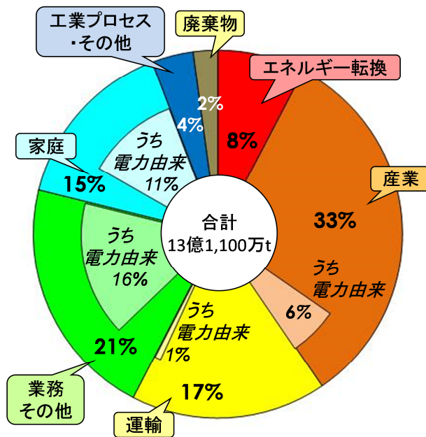
23 図2 我が国の部門別の二酸化炭素排出量 (2013年度)
