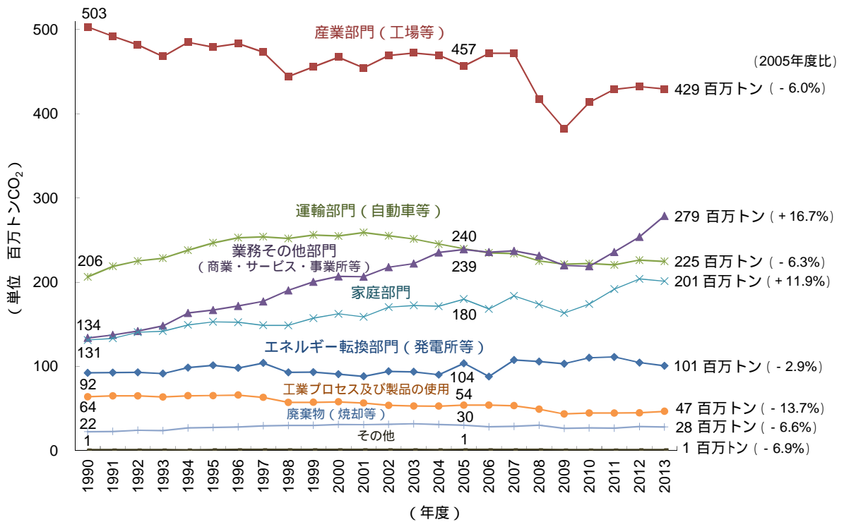
1 図1 我が国における二酸化炭素排出量の部門別の推移 2 (カッコ内の数字は各部門の2013年度排出量の2005年度排出量からの増減率)
