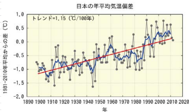
日本の年平均気温の変化 (1981~2010年平均からの偏差) 都市化の影響が比較的少ないとみられる17地点を用いた。黒線は年偏差、青線は5年移動平均、赤線は長期変化傾向。 出典 4 より
