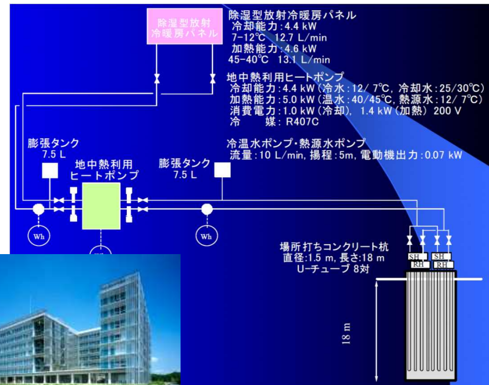
図 東京大学柏キャンパス環境棟システム概要
