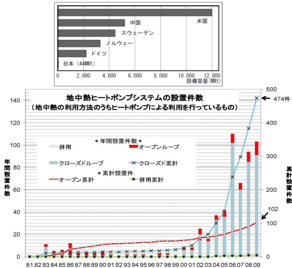
図 地中熱ヒートポンプシステムの導入実績 (上: 諸外国との比較 下: 日本における導入推移)
