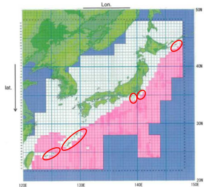
図 日本近海の波パワーの大きい海域(15kW/m以上)
