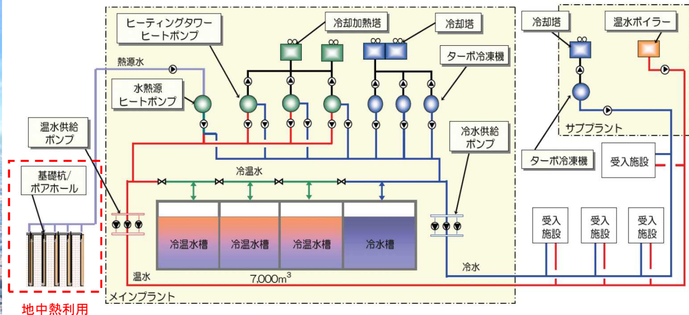
図 東京スカイツリー地区DHC システム概要
