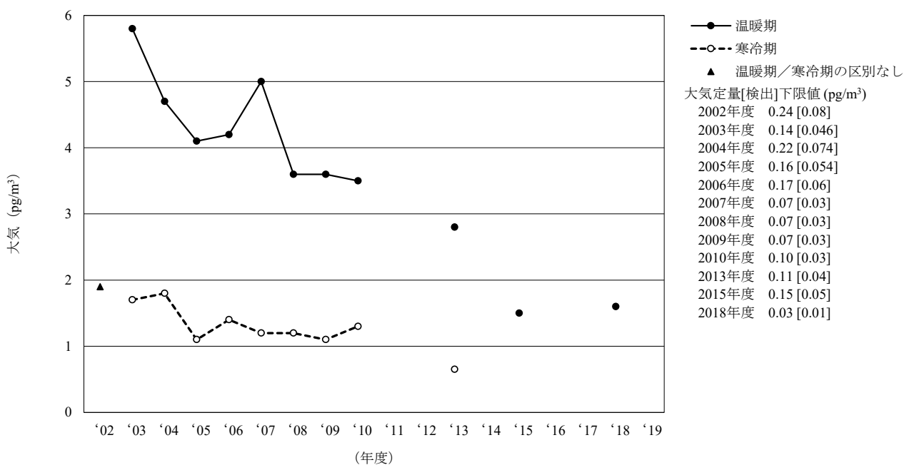
[6-1] p,p' -DDT
