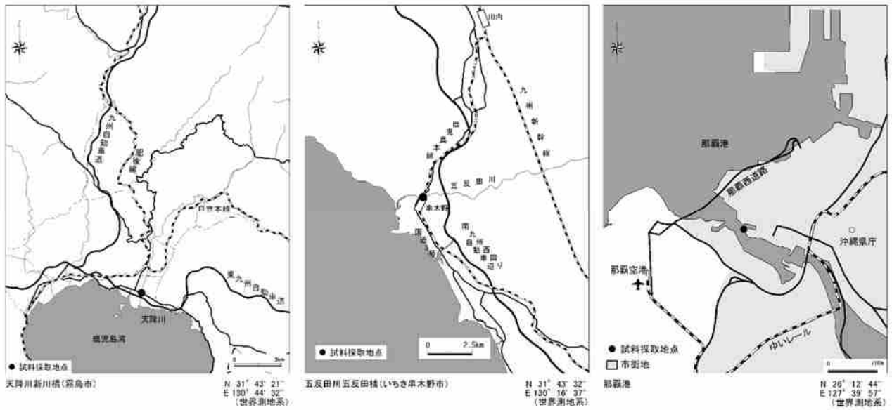
図 1-2 (6/6) 2019 年度モニタリング調査地点 (水質) 詳細
