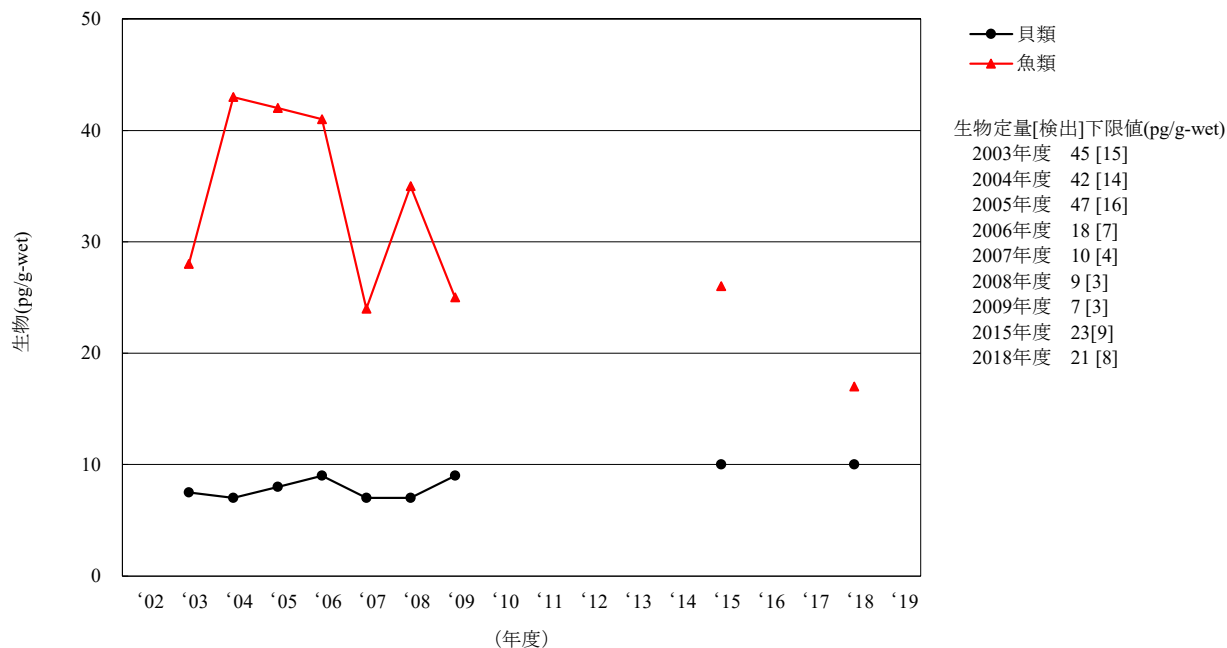
[9-1] Parlar-26
