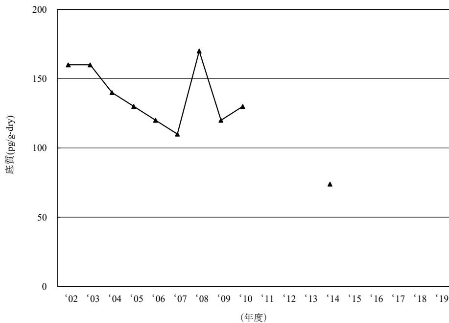
[6-6] o,p' -DDD
