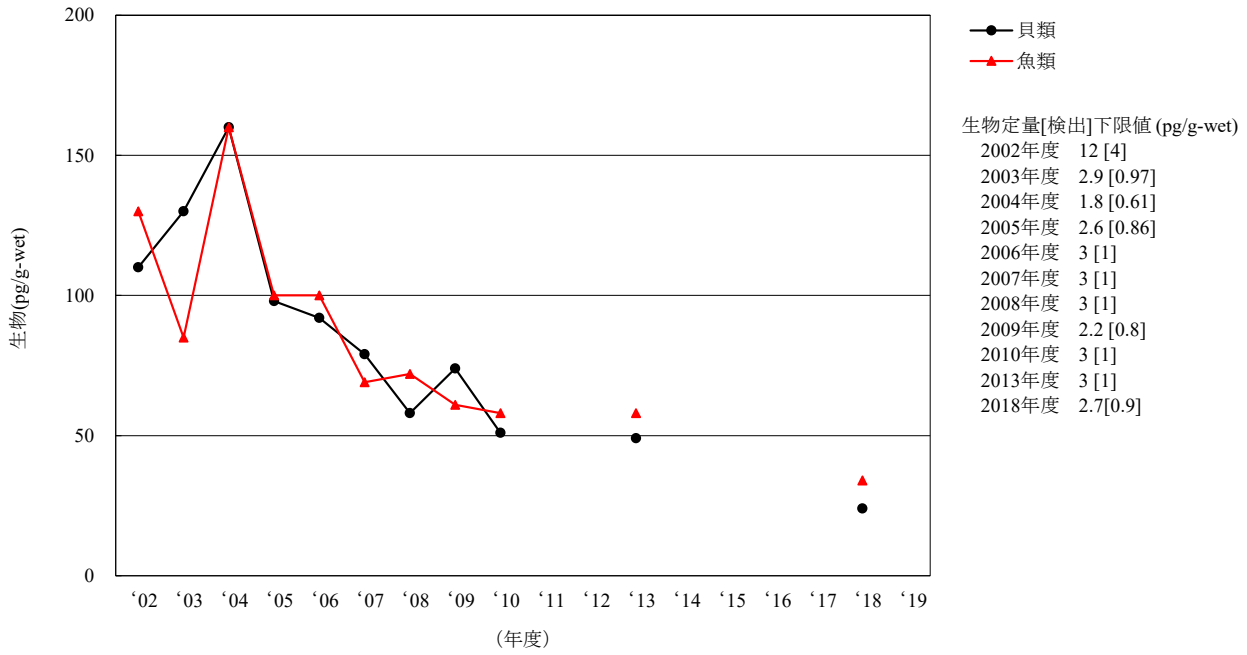
[6-4] o,p' -DDT
