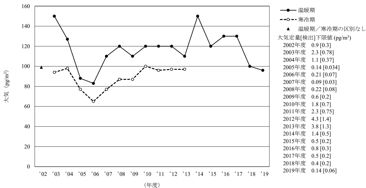
図 3-2-4 HCB の大気の経年変化 (幾何平均値)
