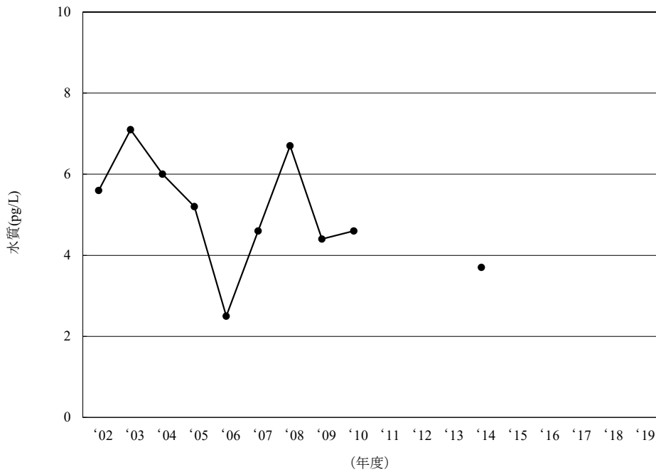
[6-6] o,p' -DDD
