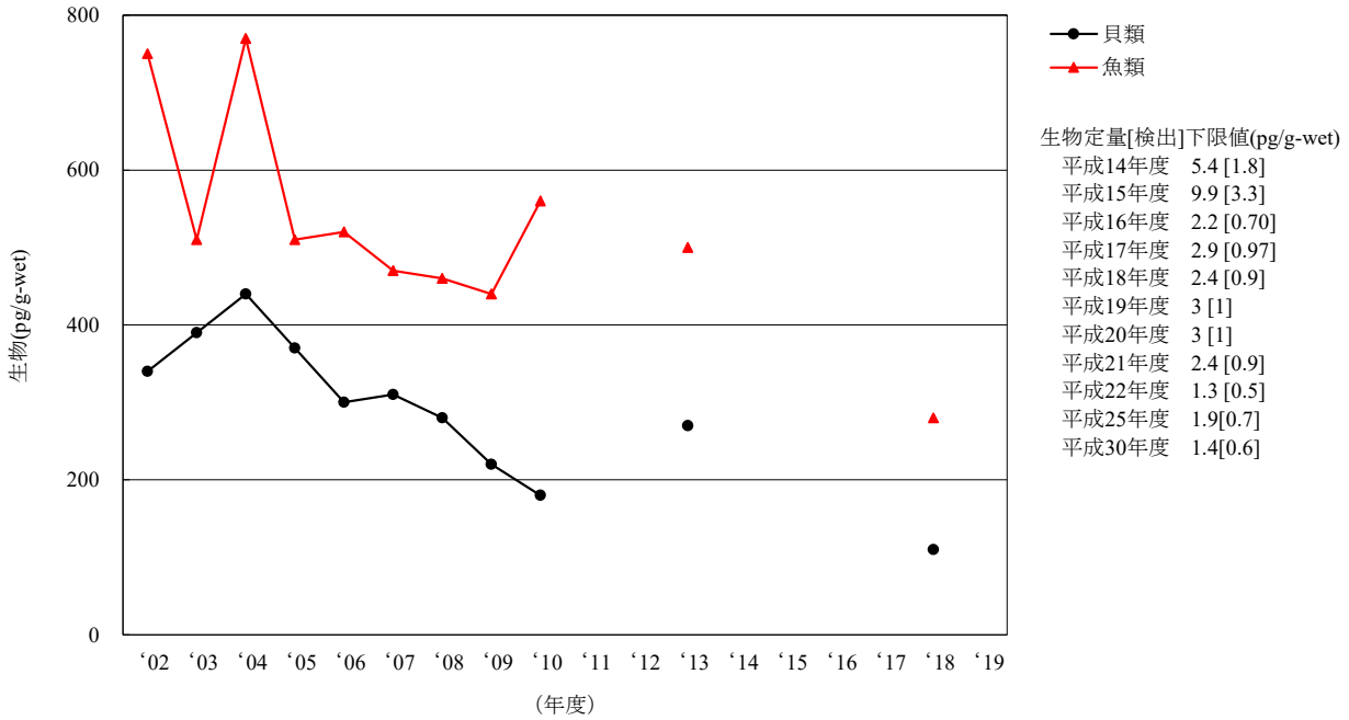
[6-3] p,p' -DDD
