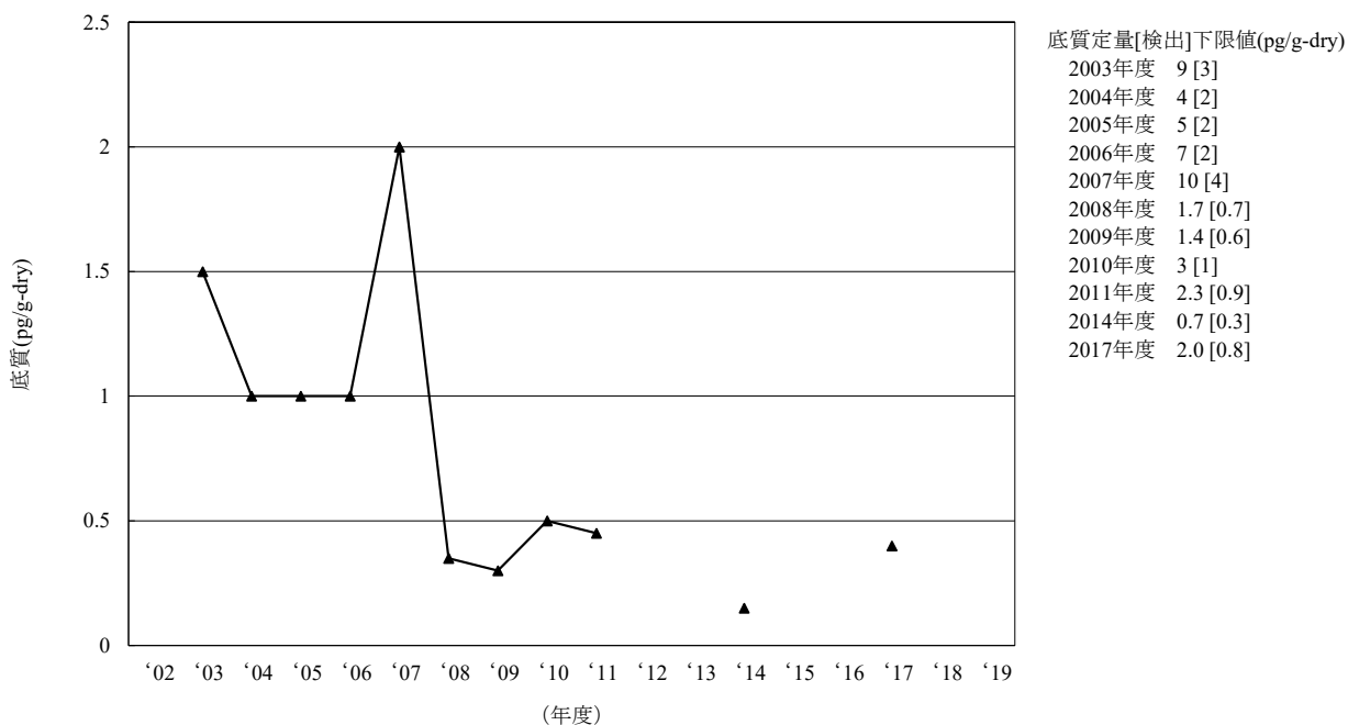
[8-3] trans -ヘプタクロルエポキシド
