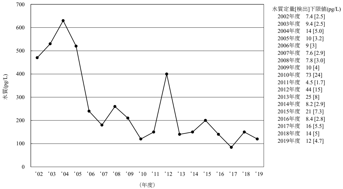
[1] 総PCB
