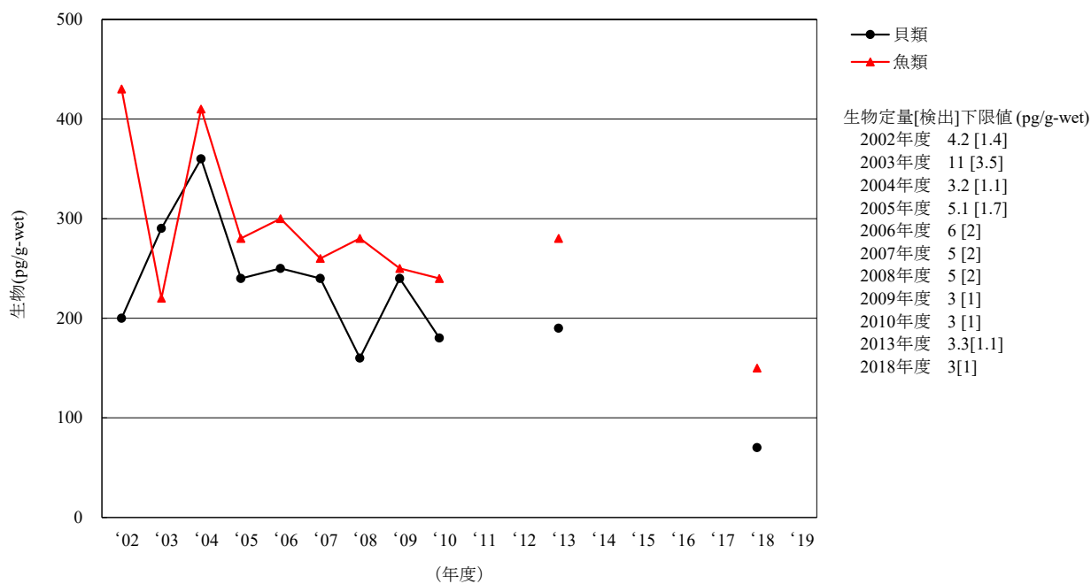
[6-1] p,p' -DDT
