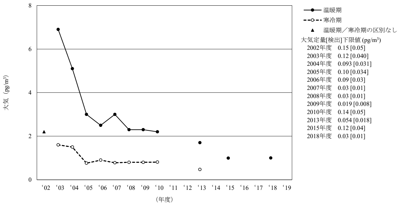
[6-4] o,p' -DDT
