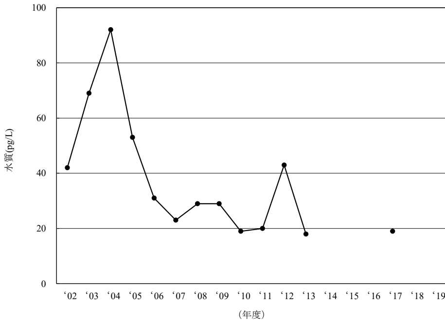
[7-1] cis-クロルデン
