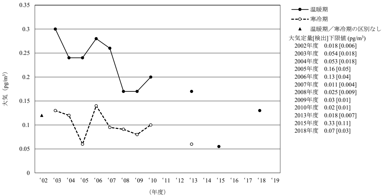
[6-3] p,p' -DDD
