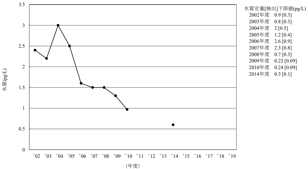
[6-5] o,p' -DDE
