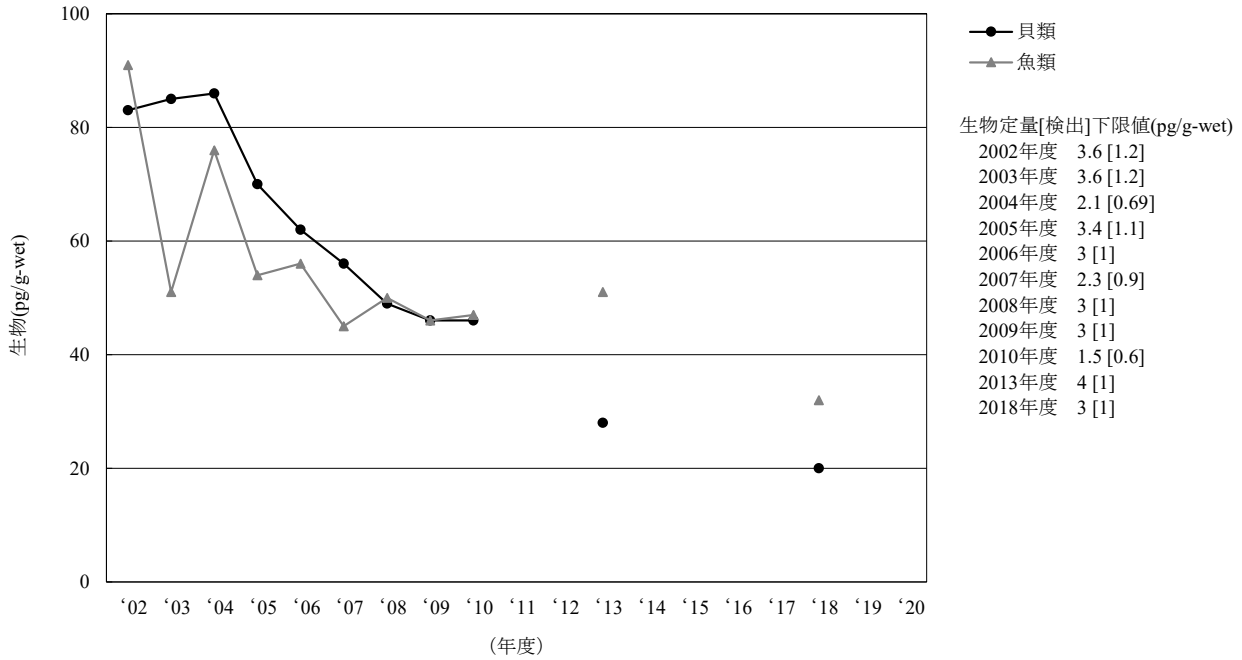
[6-5] o,p' -DDE
