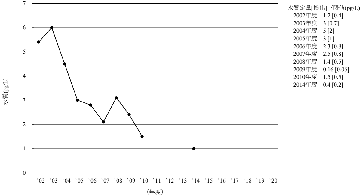
[6-4] o,p' -DDT
