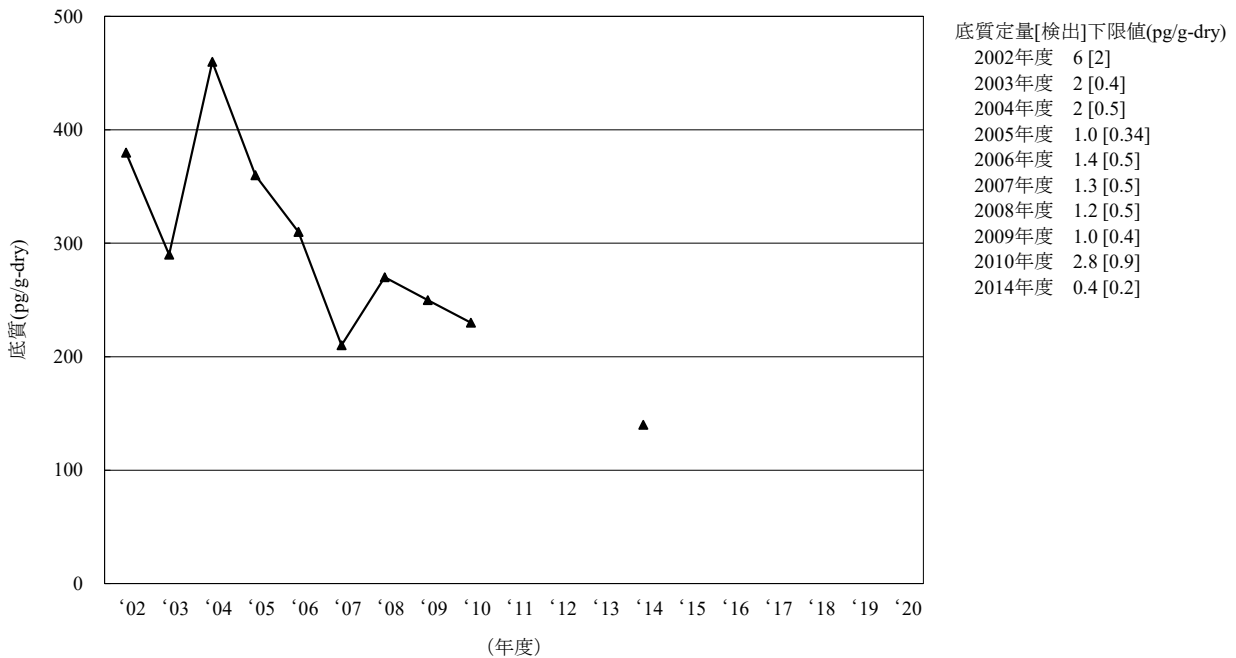
[6-1] p,p' -DDT
