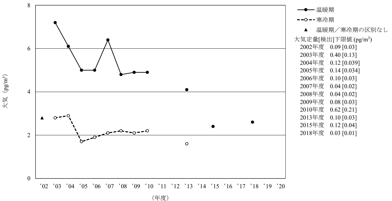
[6-2] p,p'-DDE
