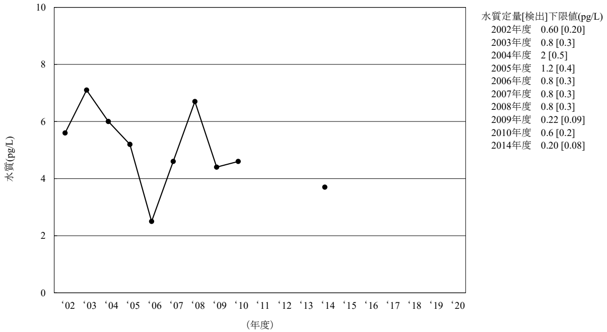
[6-6] o,p' -DDD
