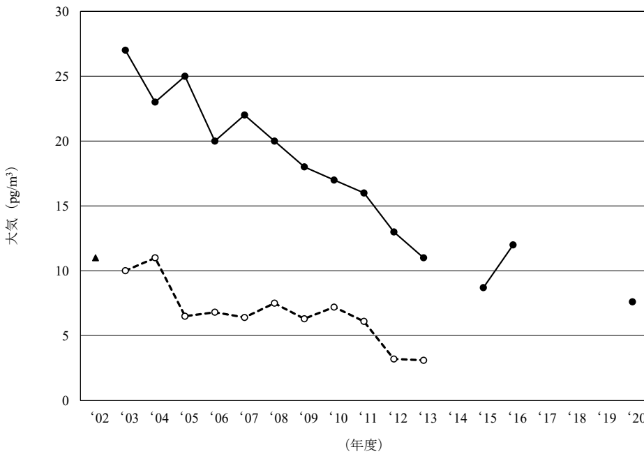
[8-1] ヘプタクロル
