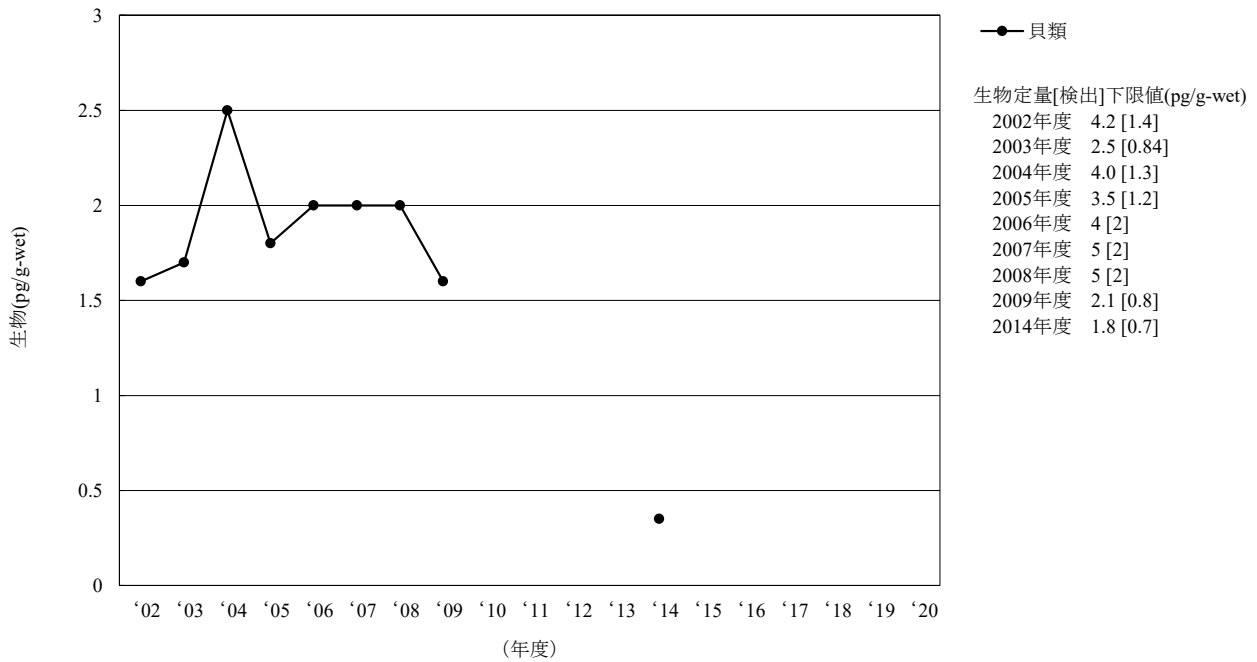
[3] アルドリン
