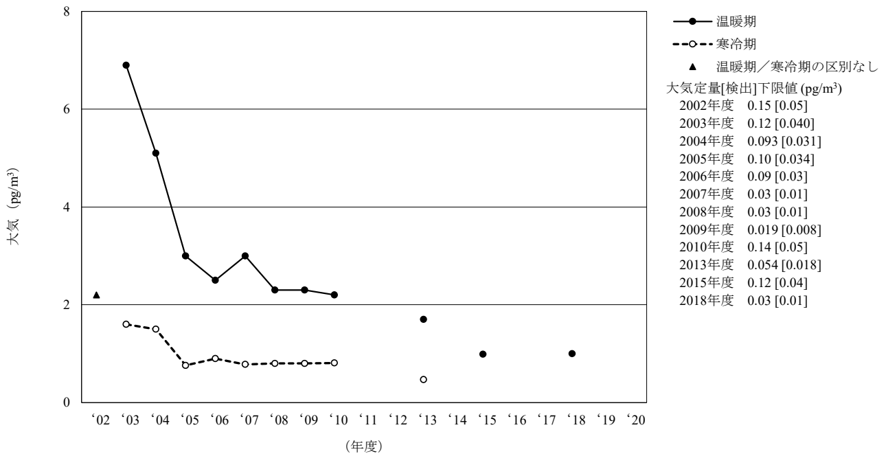
[6-4] o,p' -DDT
