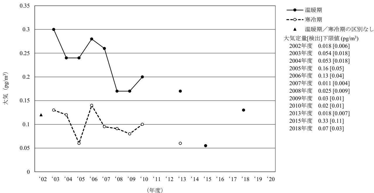
[6-3] p,p' -DDD
