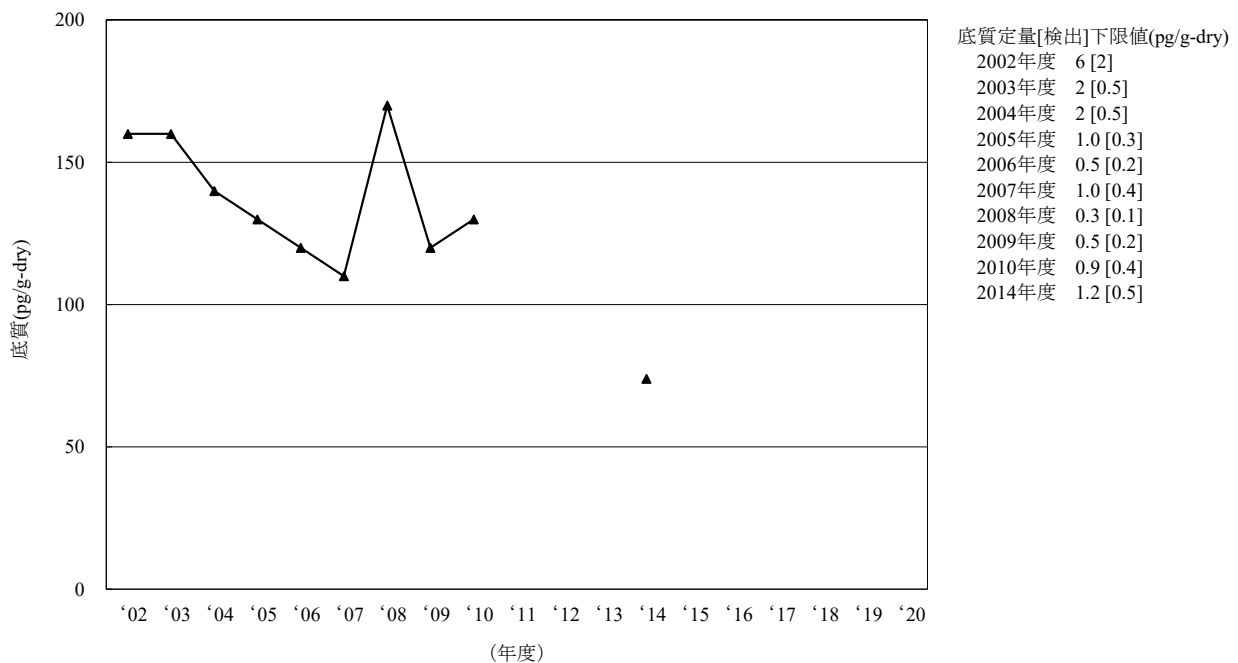
[6-6] o,p' -DDD
