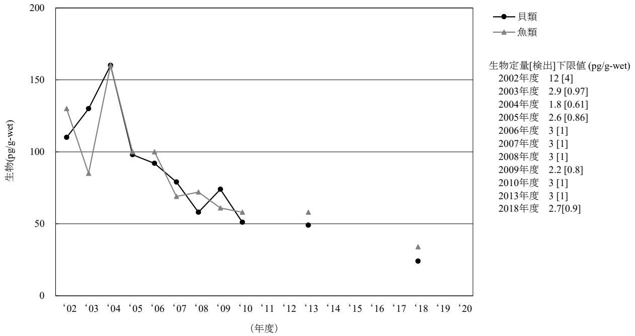
[6-4] o,p' -DDT
