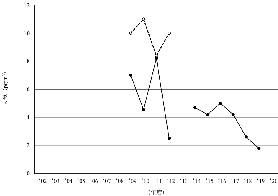
[14-7] デカブロモジフェニルエーテル類
