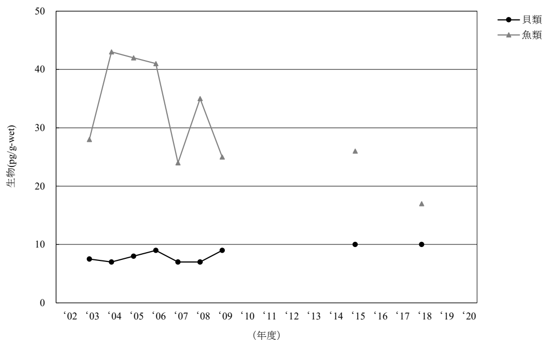
[9-1] Parlar-26
