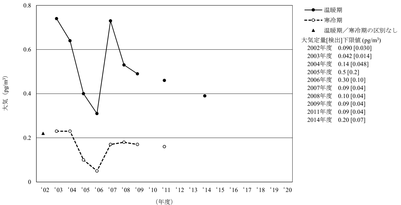
[5] エンドリン
