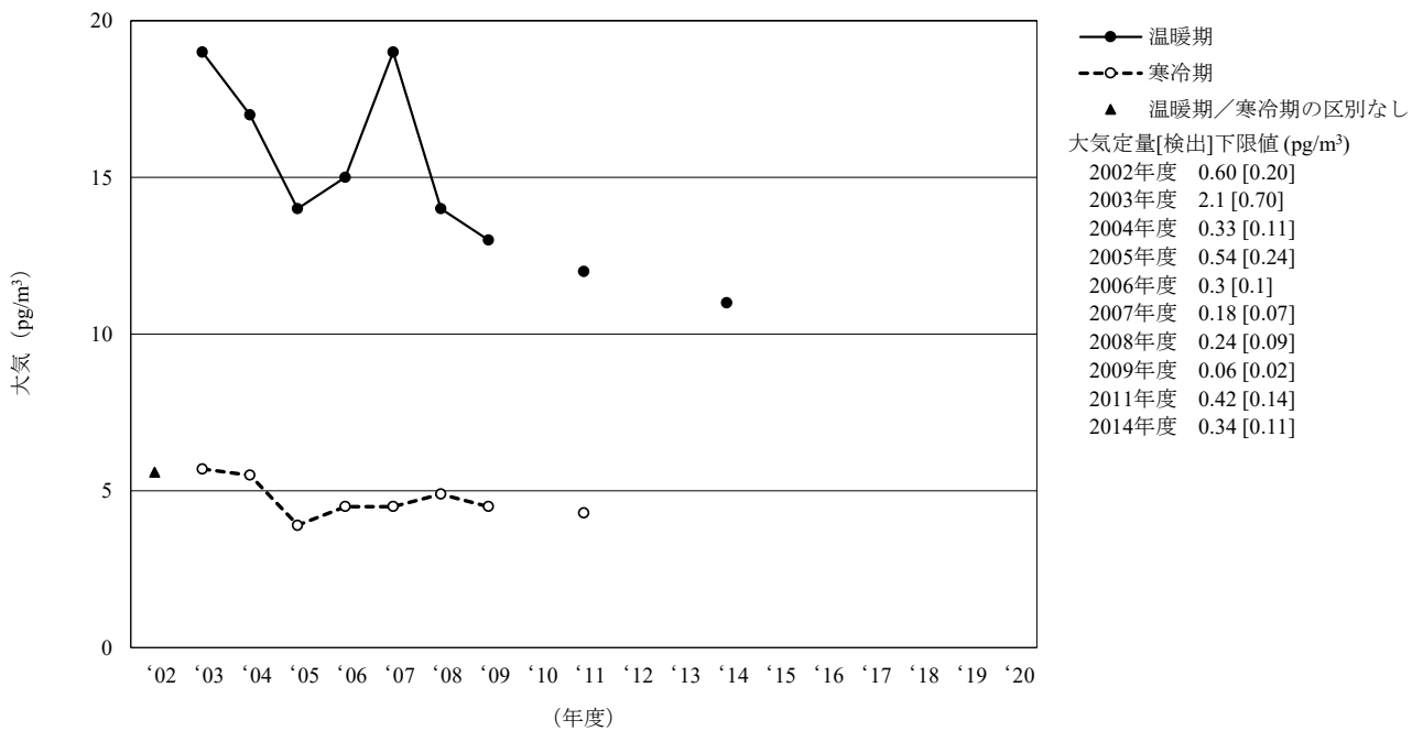
[4] ディルドリン
