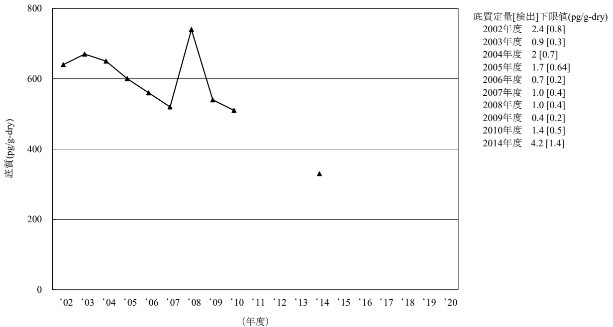
[6-3] p,p' -DDD
