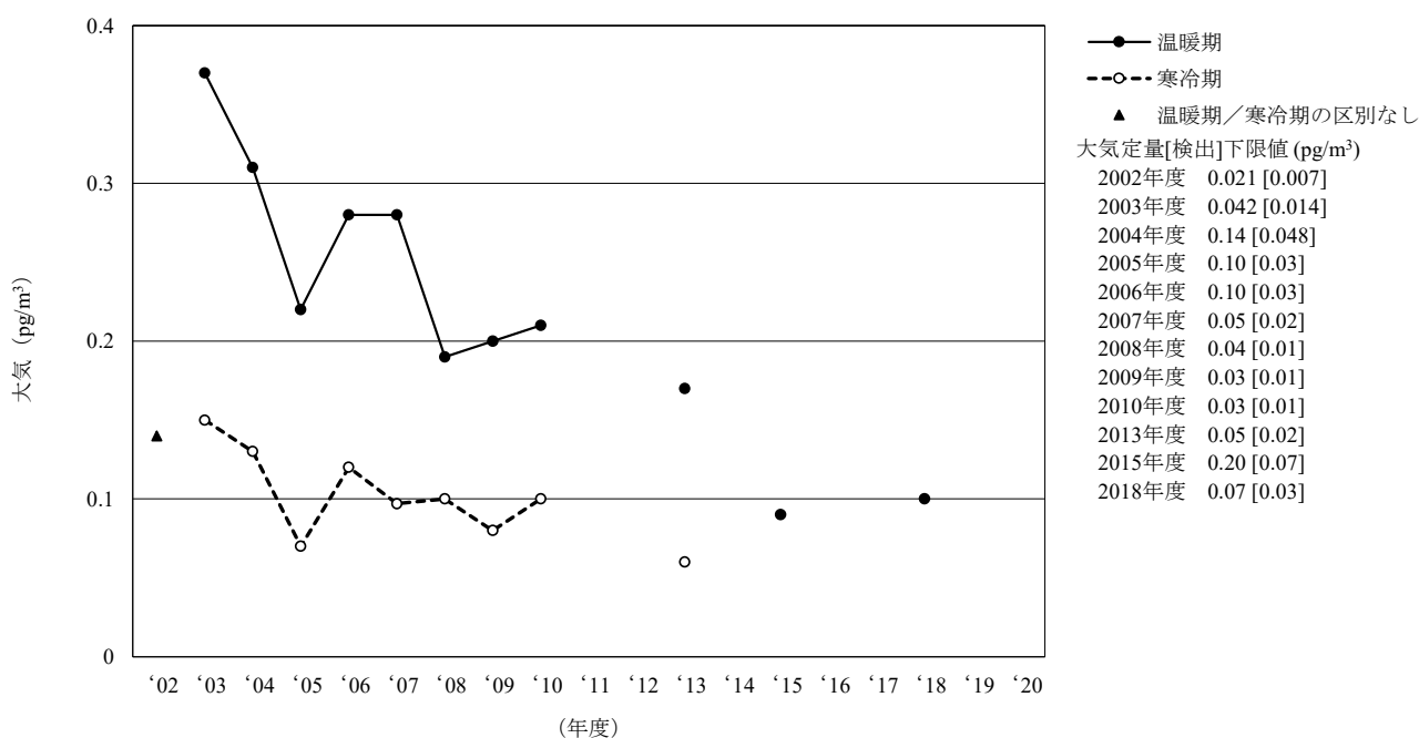
[6-6] o,p' -DDD
