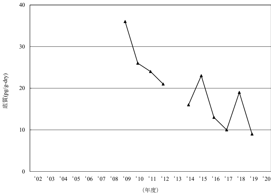
[14-2] ペンタブロモジフェニルエーテル類
