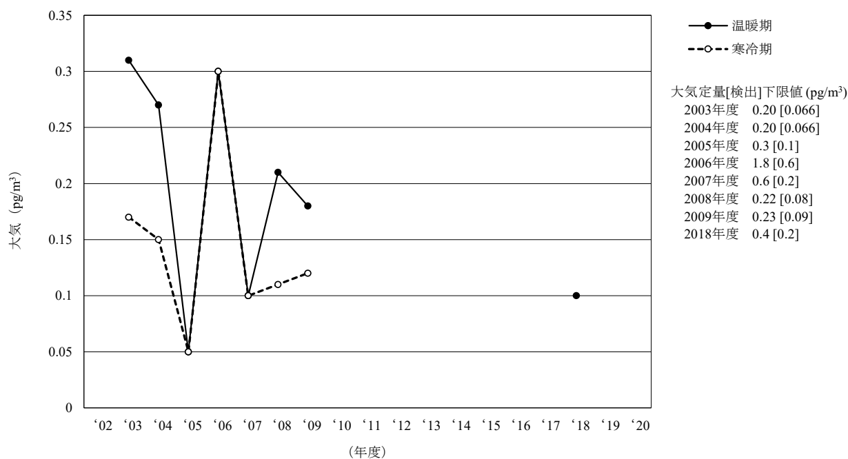
[9-1] Parlar-26
