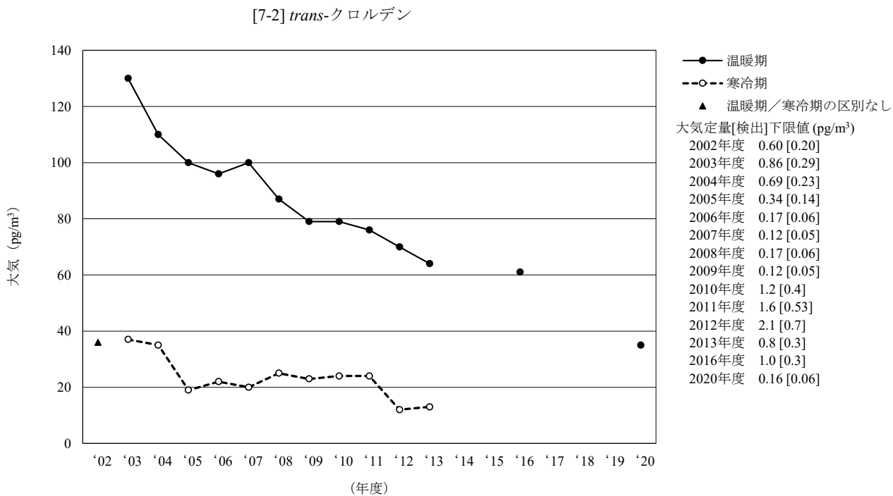
図 3-7-2-4 trans -クロロデンの大気の経年変化 (幾何平均値)
