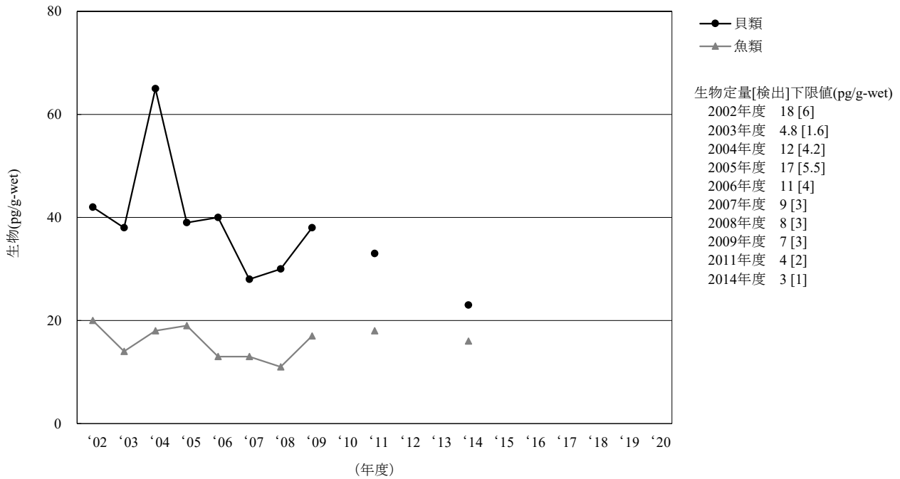
[5] エンドリン
