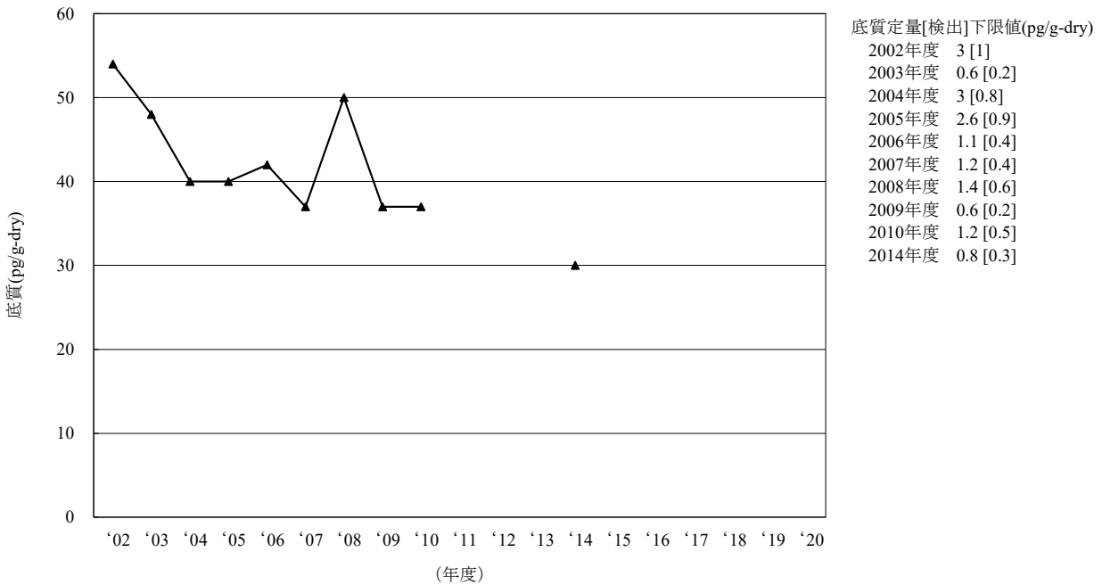
[6-5] o,p' -DDE
