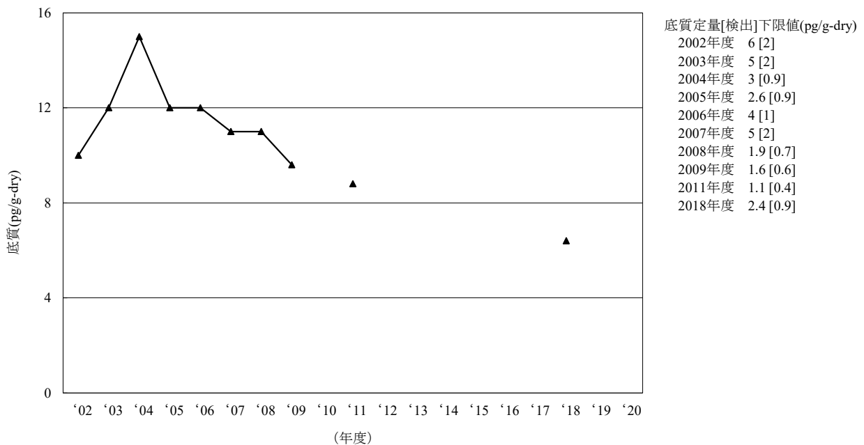
[5] エンドリン
