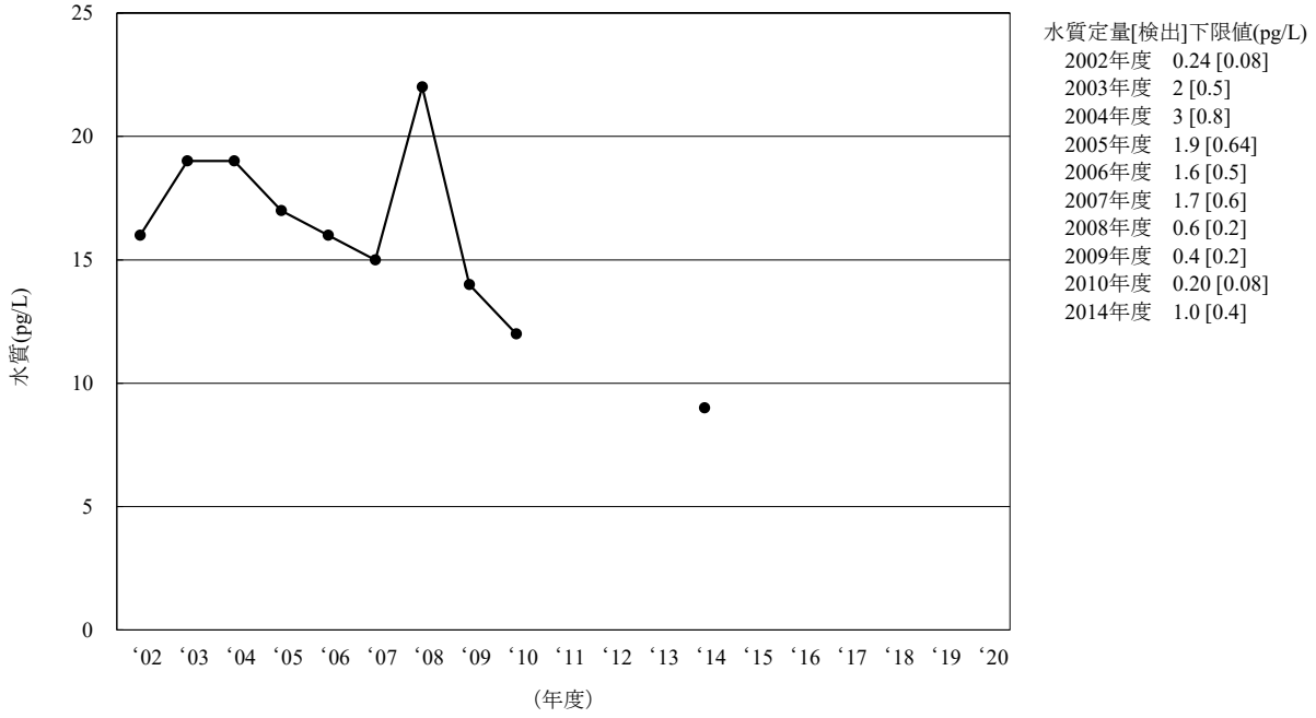
[6-3] p,p' -DDD
