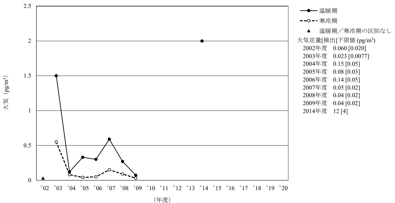
[3] アルドリン
