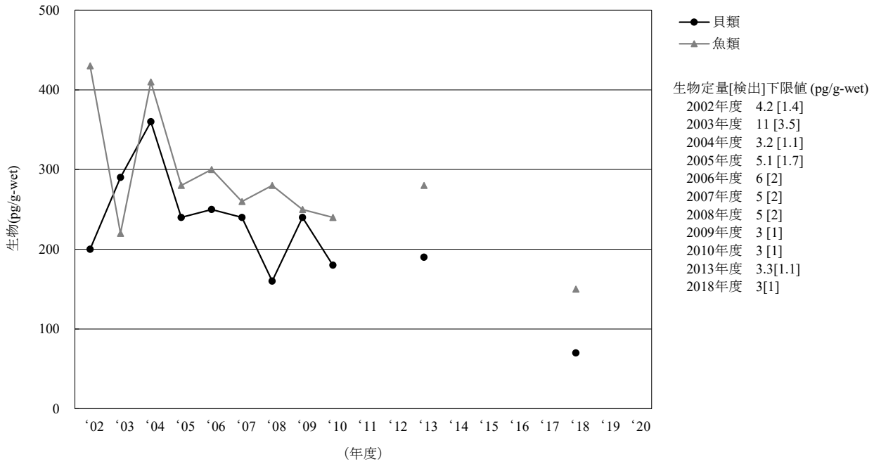
[6-1] p,p'-DDT
