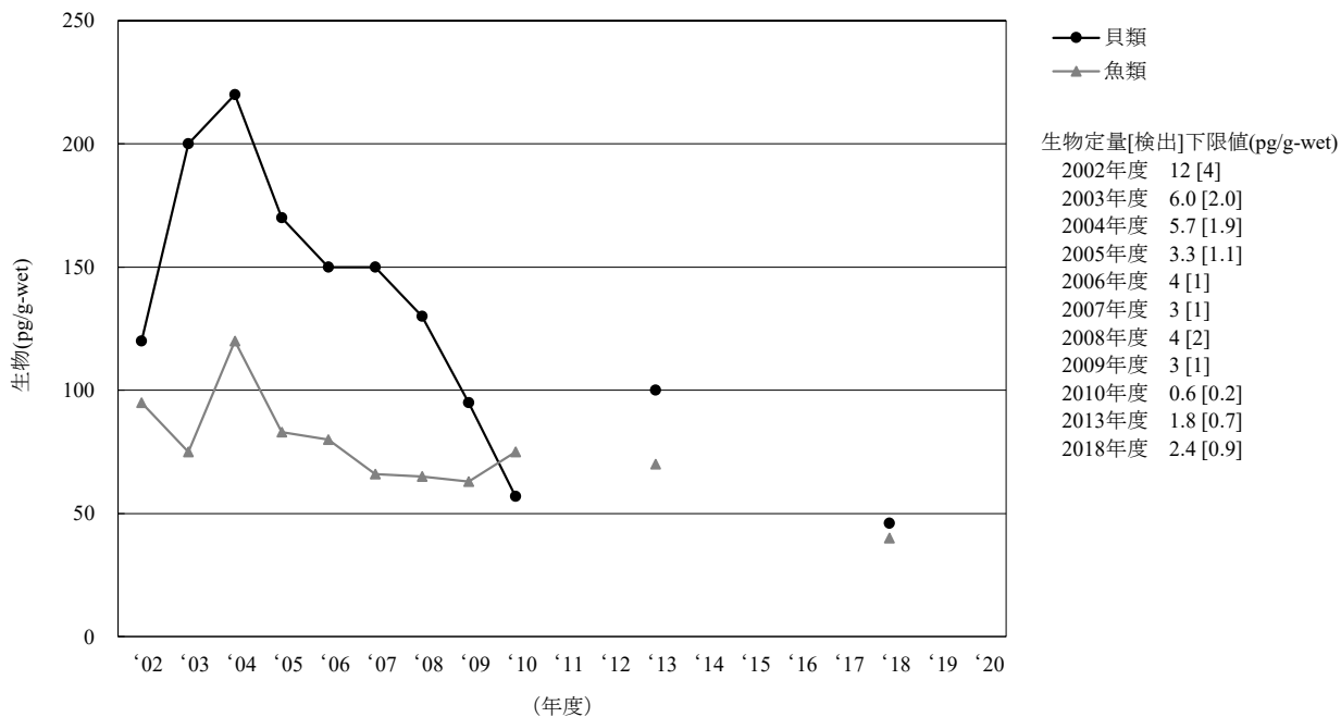
[6-6] o,p' -DDD
