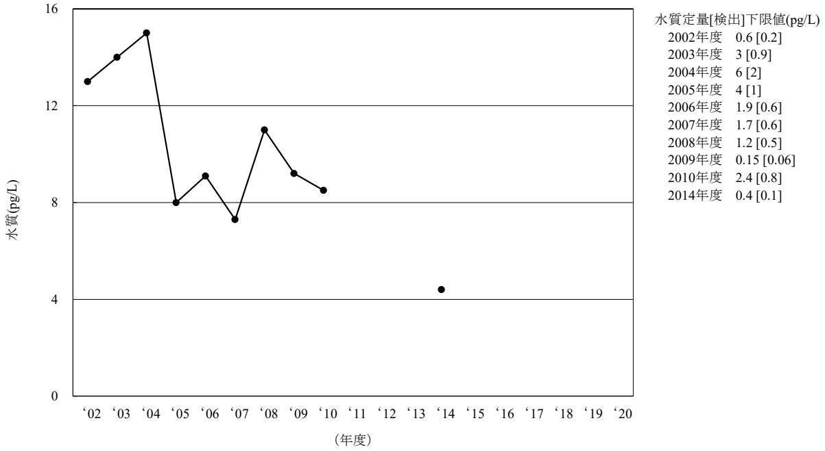
[6-1] p,p' -DDT
