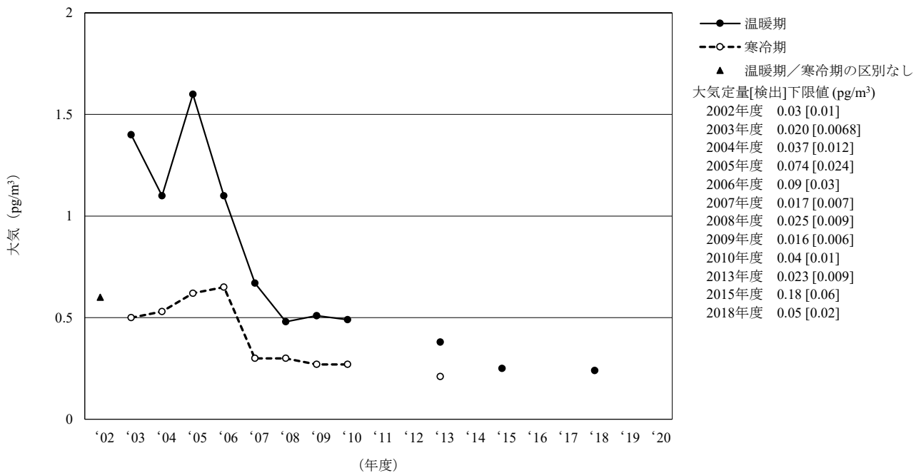
[6-5] o,p' -DDE
