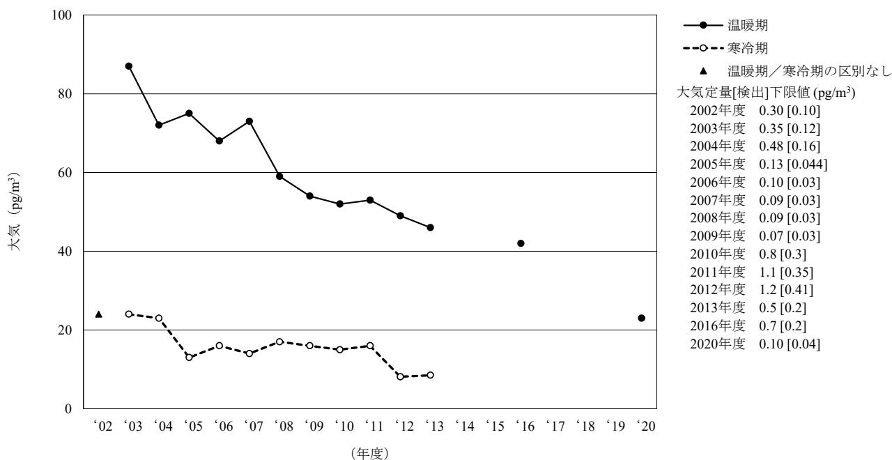
[7-5] trans -ノナクロール
