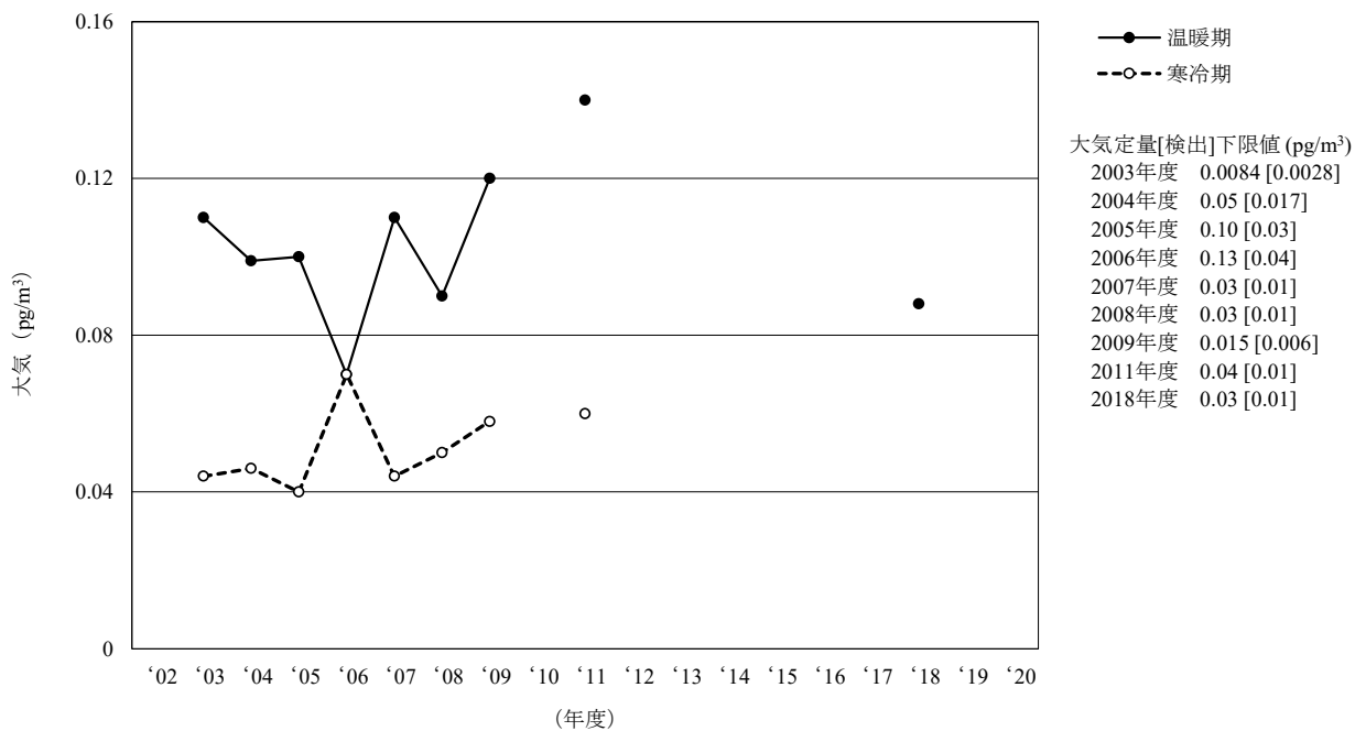
図 3-10-4 マイレックスの大気の変動 (幾何平均値)
