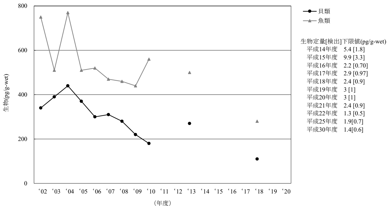
[6-3] p,p' -DDD
