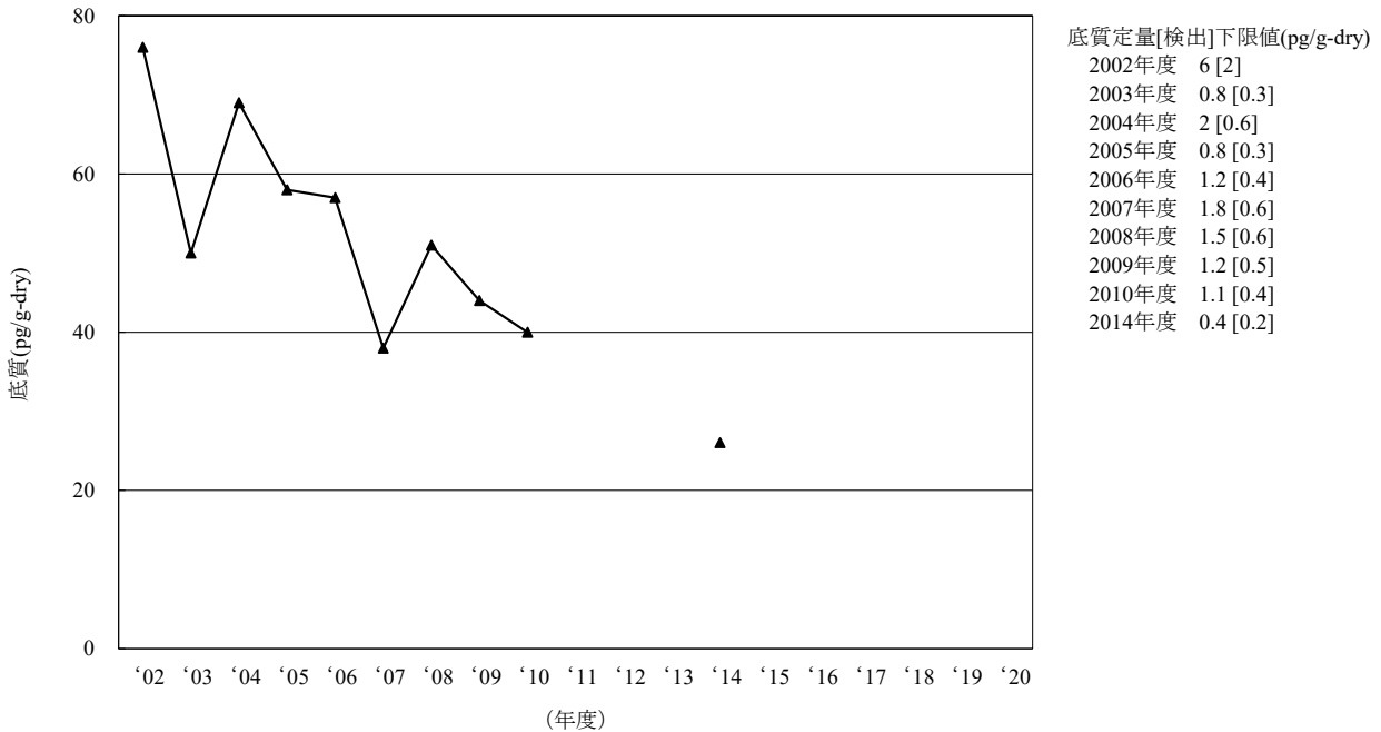
[6-4] o,p' -DDT
