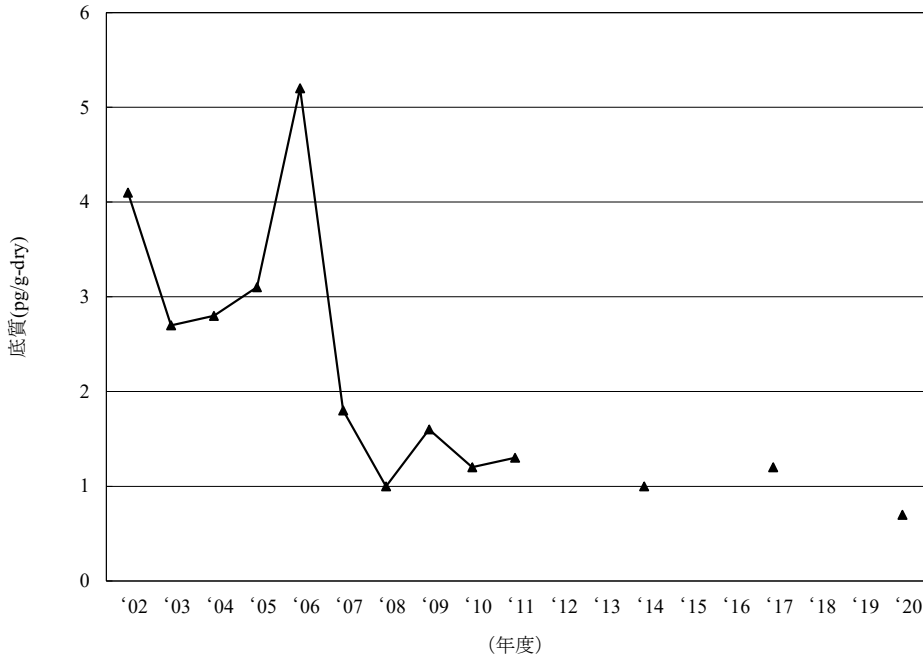
[8-1] ヘプタクロル
