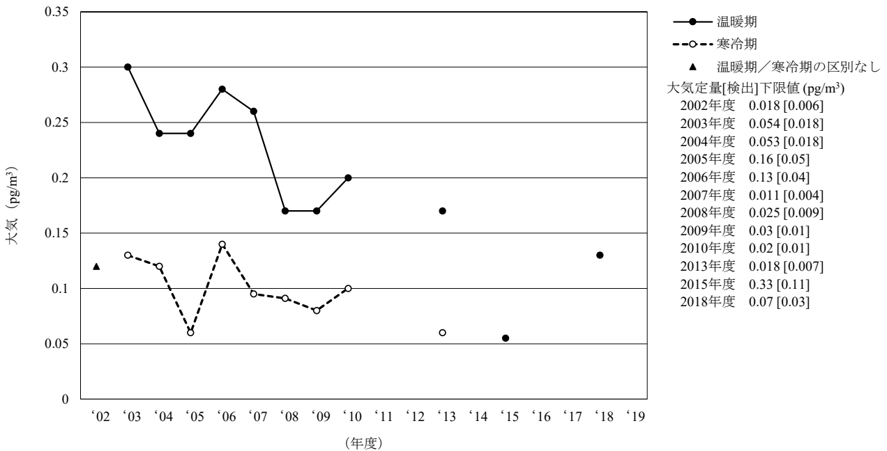
[6-3] p,p' -DDD
