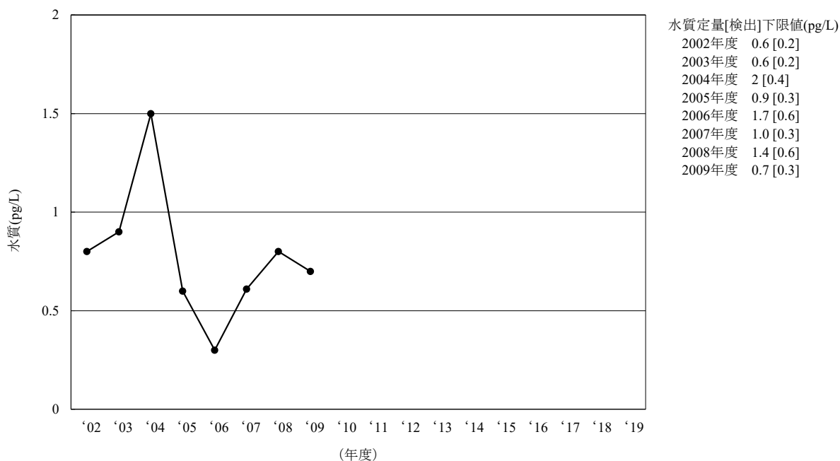
[3] アルドリン
