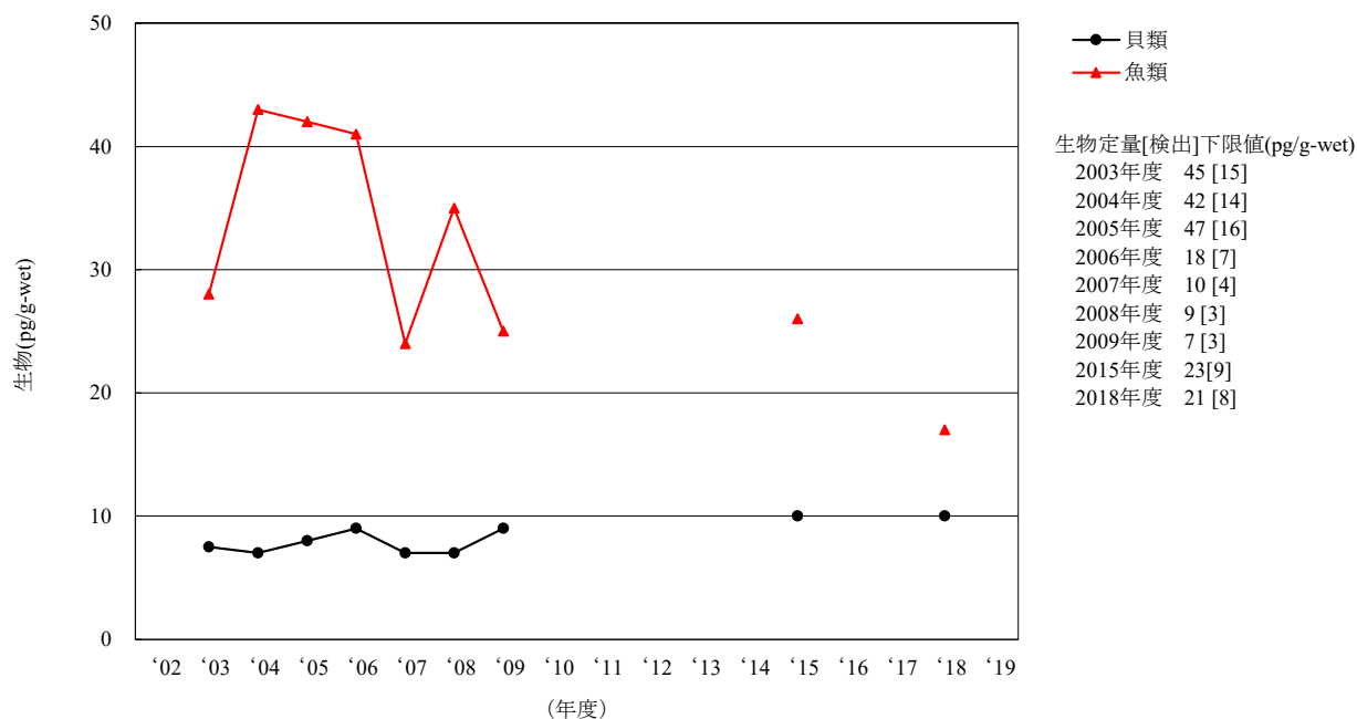
[9-1] Parlar-26
