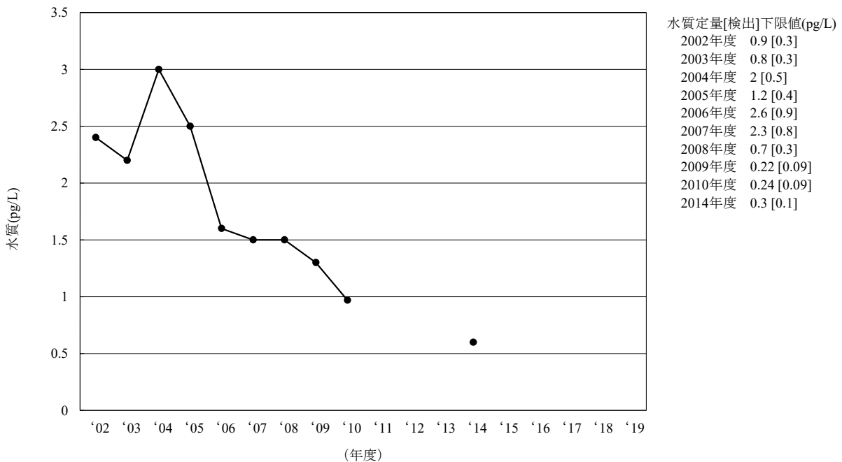
[6-5] o,p' -DDE
