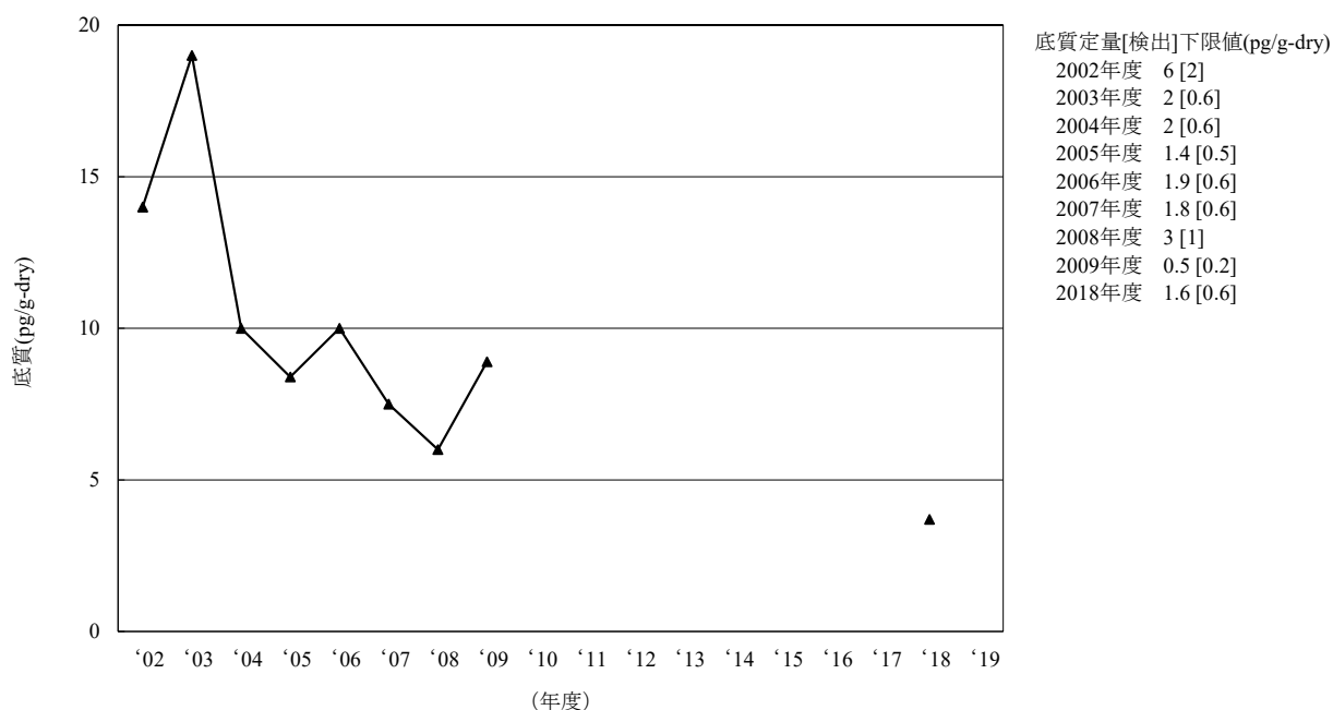
[3] アルドリン
