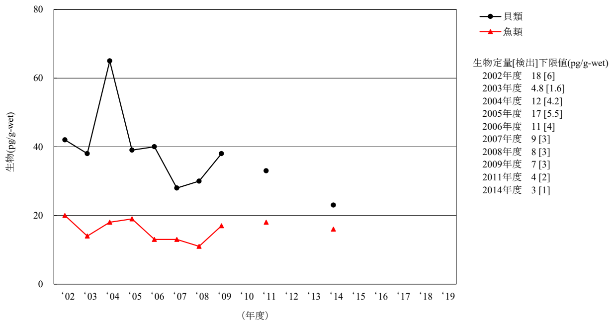
[5] エンドリン
