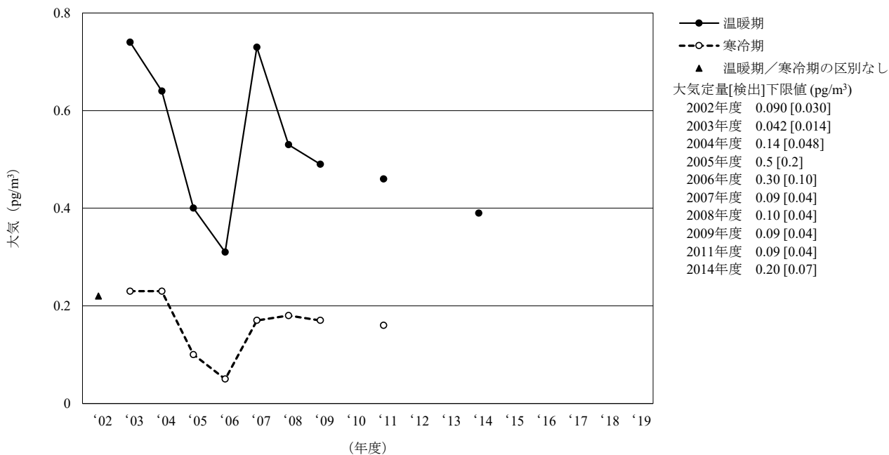
[5] エンドリン
