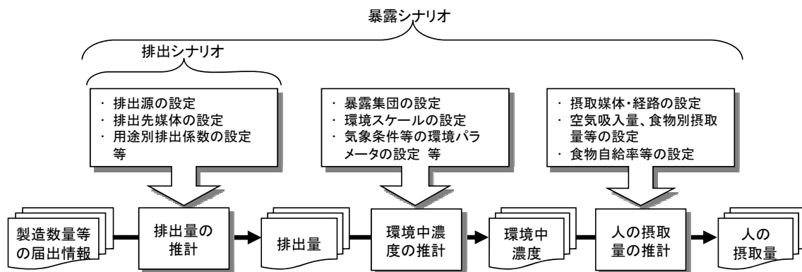
20 図表 V-5 製造数量等の届出制度の情報から人の摂取量を推計する流れ
